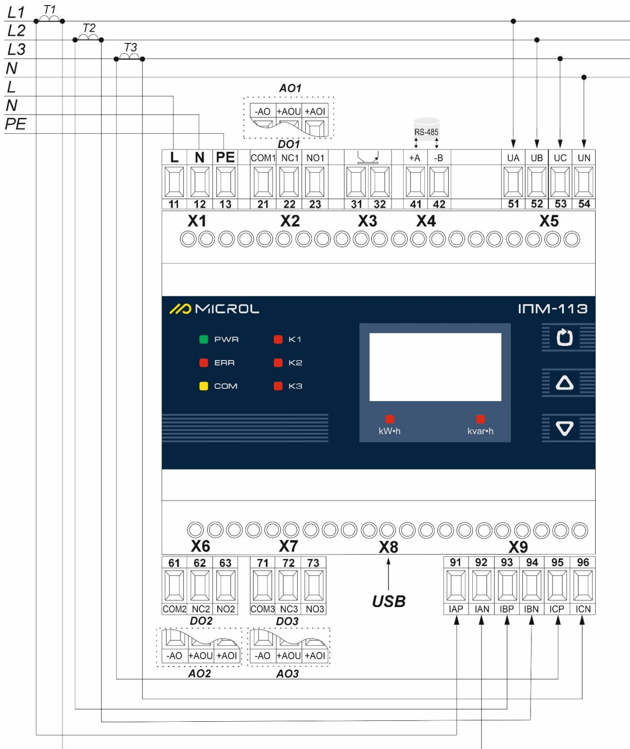
Рисунок Б.2 - Підключення зовнішніх ланцюгів індикатора ІПМ-113 до трьох фазної мережі через трансформатори струму.
