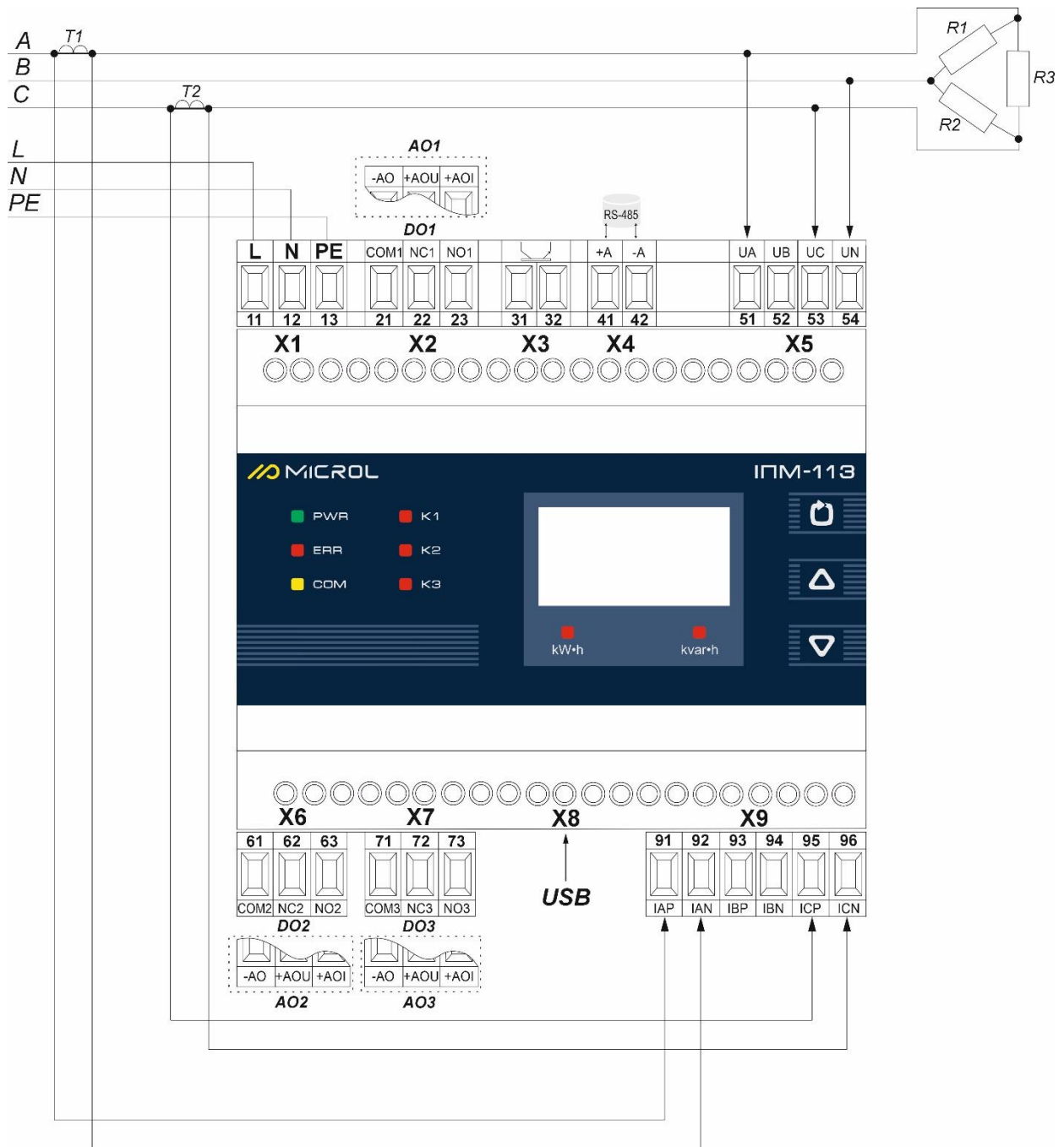
Рисунок Б.5 - Підключення зовнішніх ланцюгів індикатора ІПМ-113 до трьох фазної мережі за схемою трикутника (схема Арона). Перед підключенням індикатора за схемою трикутника, додатково програмним способом в конфігурації індикатора в параметрі CONN MODE встановити значення 1.
