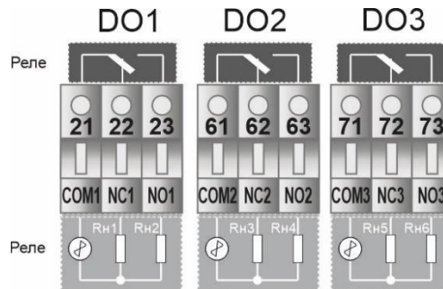
Рисунок Б.2.2 – Схема підключення виходу, тип «Р» - перекидне реле
