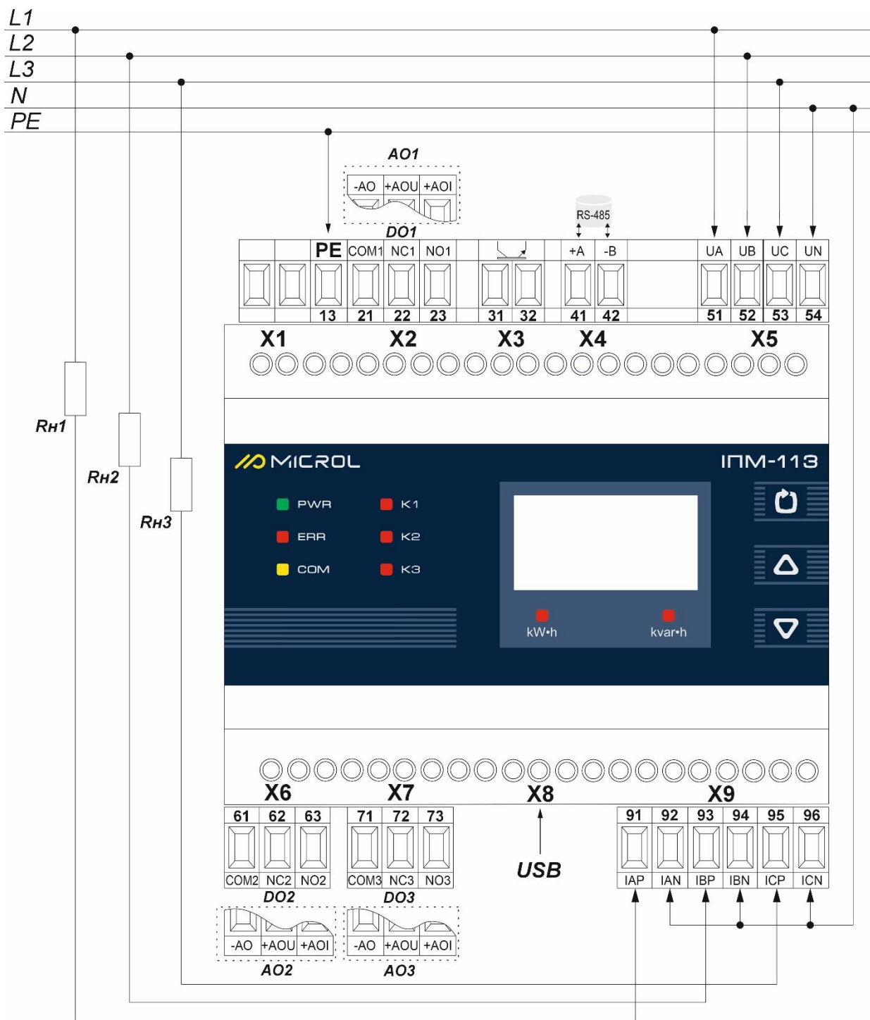
Рисунок Б.4 - Підключення зовнішніх ланцюгів індикатора ІПМ-113 з живленням від вимірювальної мережі.
