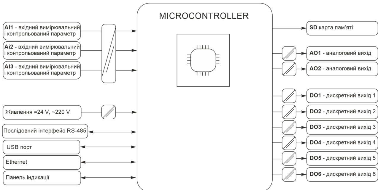
Рисунок 3.2 - Структурна схема індикатора ITM-320 (ITM-320A)
