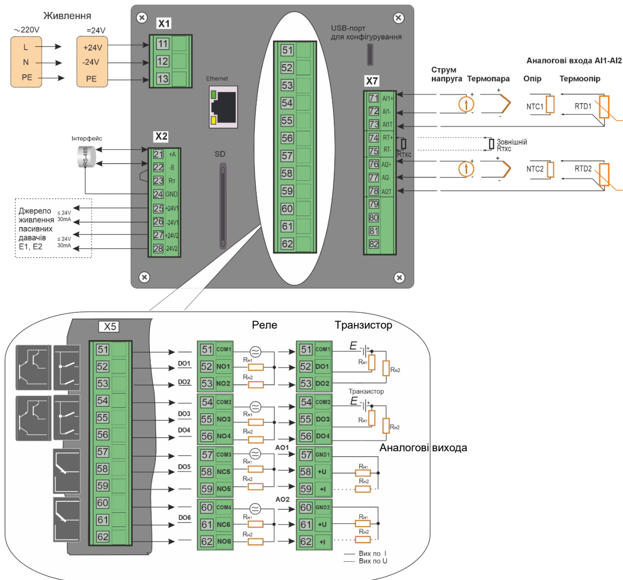
Рисунок Б.1 - Схема зовнішніх з'єднань індикатора ITM-320 (ITM-320A)
