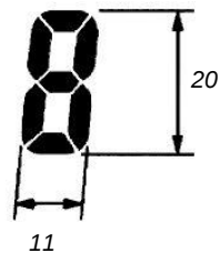
Рисунок А.1 – Зовнішній вигляд індикатора ITM-320 та розміри цифрових індикаторів(тип індикаторів - 0)
