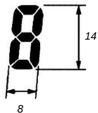
Рисунок А.2 – Зовнішній вигляд індикатора ITM-320A та розміри цифрових індикаторів(тип індикаторів - 0)
