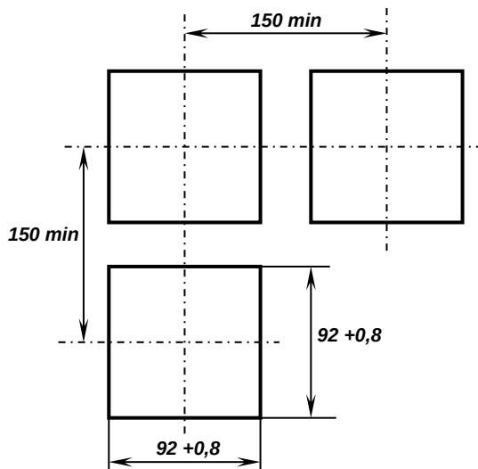
Рисунок А.4 – Розмітка отворів на щиті для встановлення індикатора
