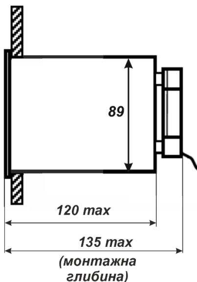
Рисунок А.3 – Габаритні розміри індикатора
