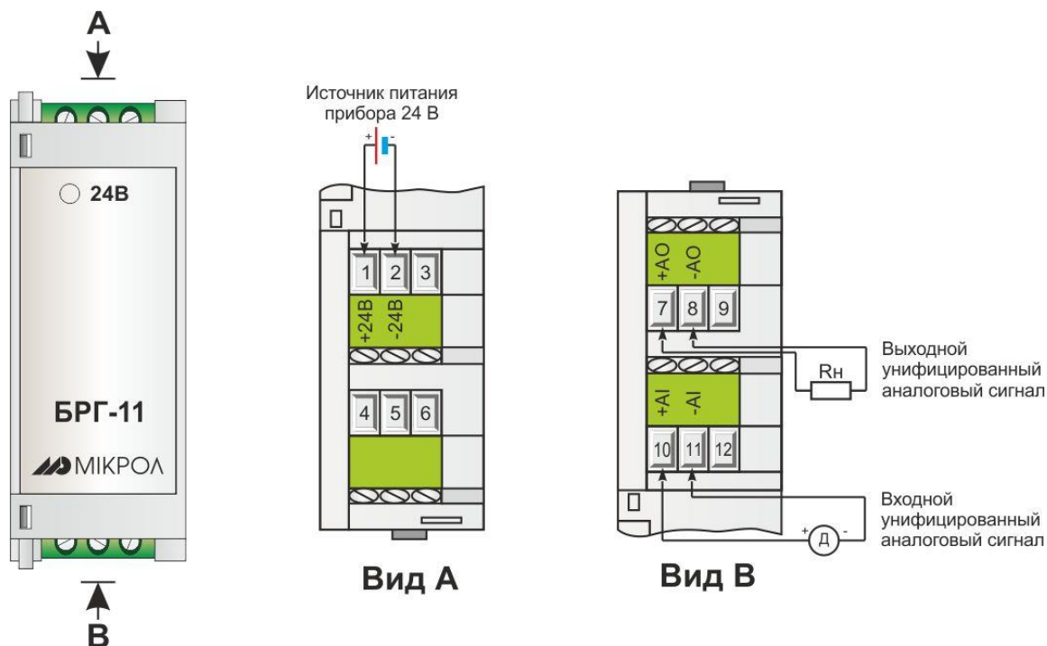
Рисунок 3.3 - Схема электрической подключений блока БРГ-11
