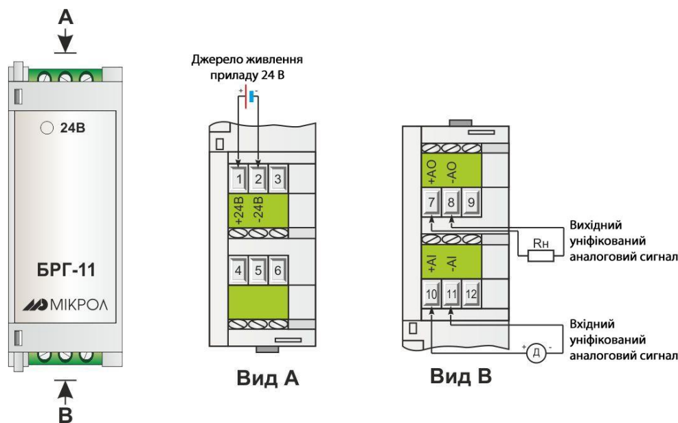
Рисунок 3.3 - Схема електрична підключень блоку БРГ-11
