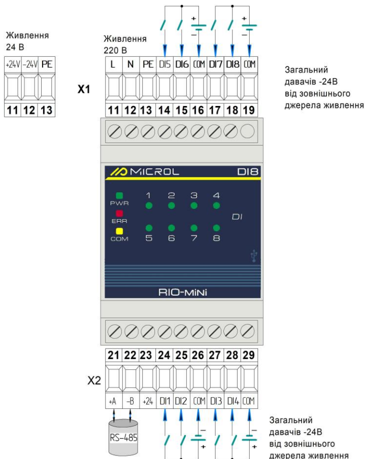
Малюнок Б.2 - Підключення зовнішніх ланцюгів модуля RIO-MINI DI8 із зовнішнім джерелом живлення та спільним «-»
