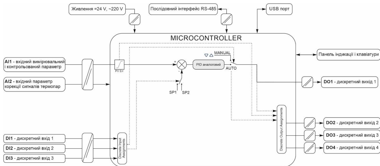
Рисунок 4.5 - Функціональна схема регулятора МІК-311-К4 в режимі роботи ПІД-ШІМ регулятора
