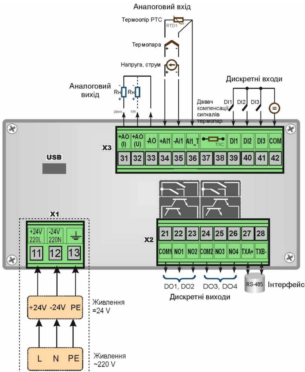
Рисунок Б.1 - Схема зовнішніх з'єднань регулятора МІК-311-К4 (версія без джерела живлення пасивного датчика та трьох дискретними входами)
