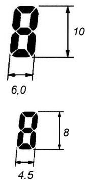
Рисунок А.1 – Зовнішній вигляд регулятора МІК-311-К4 та розміри цифрових індикаторів
