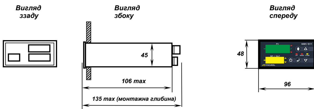
Рисунок А.1 – Зовнішній вигляд регулятора МІК-311-К4 та розміри цифрових індикаторів
