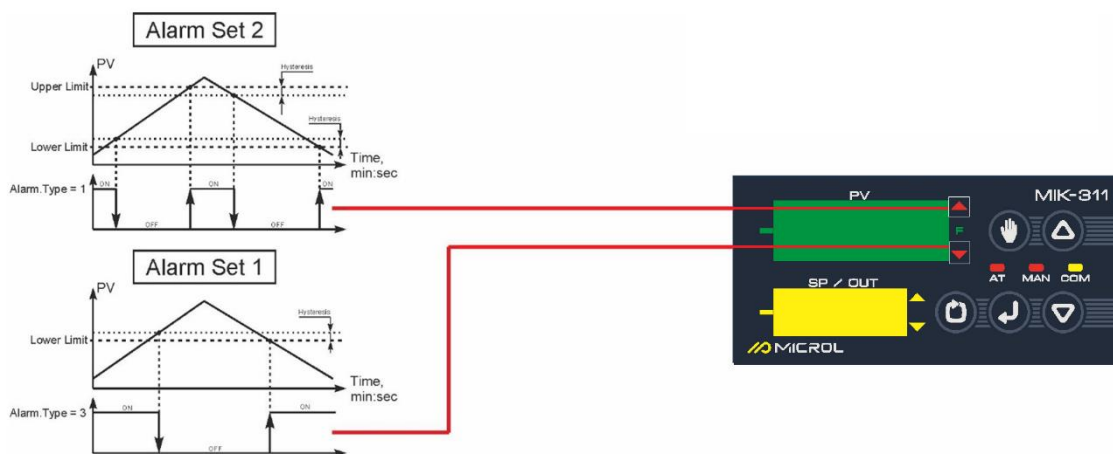
Рисунок 4.8 – Принцип роботи сигналізації
