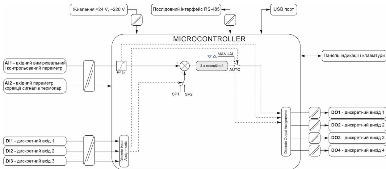
Рисунок 4.4 - Структурна схема регулятора MIK-311-K11 в режимі роботи 3-х позиційного регулятора
