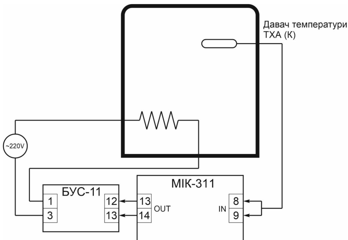
Рисунок 4.12 – Схема та процес термічної обробки
