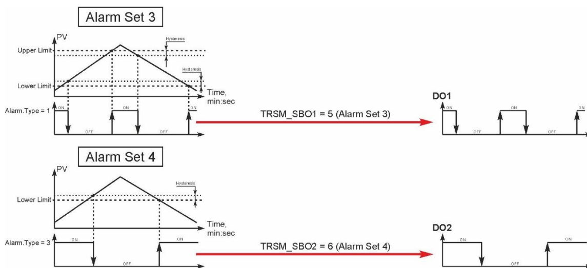
Рисунок 4.11 – Приклад налаштування роботи дискретних виходів
