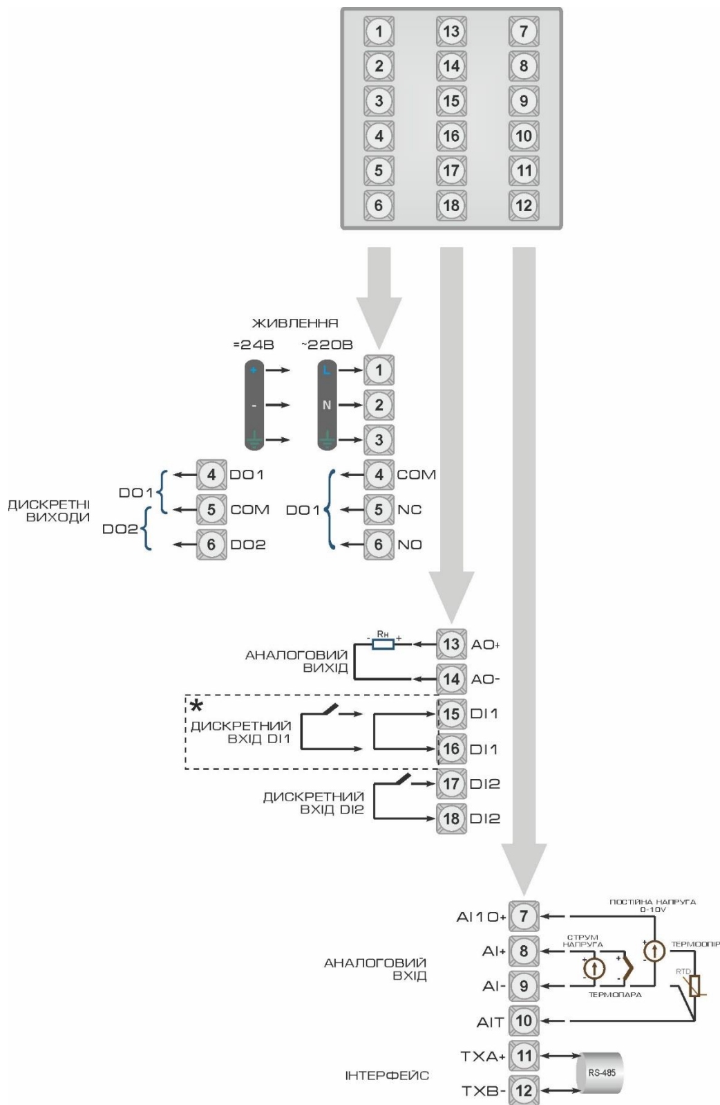
Рисунок Б.1 - Схема зовнішніх з'єднань регулятора MIK-311-K11
