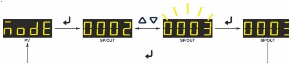
Рисунок 3.5 – Фіксація зміни параметру регулятора MIK-311-K11
