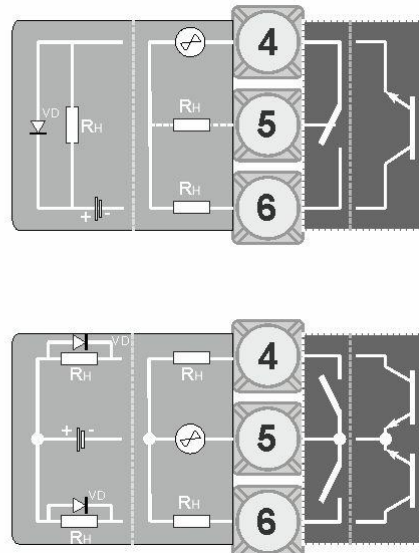
Рисунок Б.4 - Підключення дискретних навантажень до регулятора МІК-311-К11
