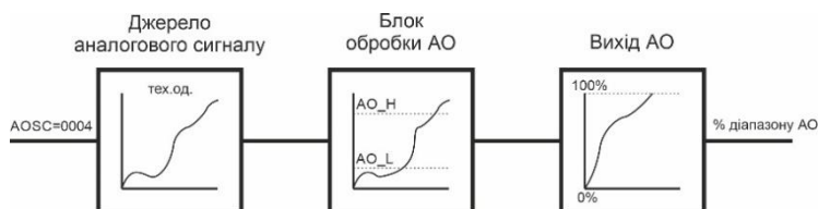
Рисунок 3.8 - Робота блоку аналогового виходу в режимі перетворення
