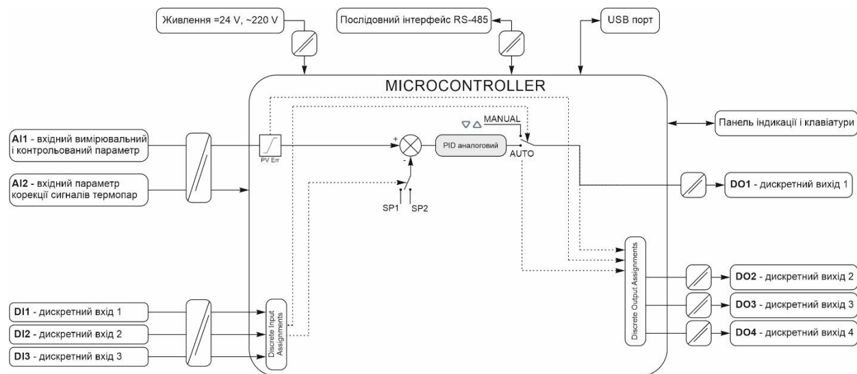
Рисунок 4.7 - Структурна схема регулятора МІК-311-К11 в режимі роботи ПІД-ШИМ регулятора
