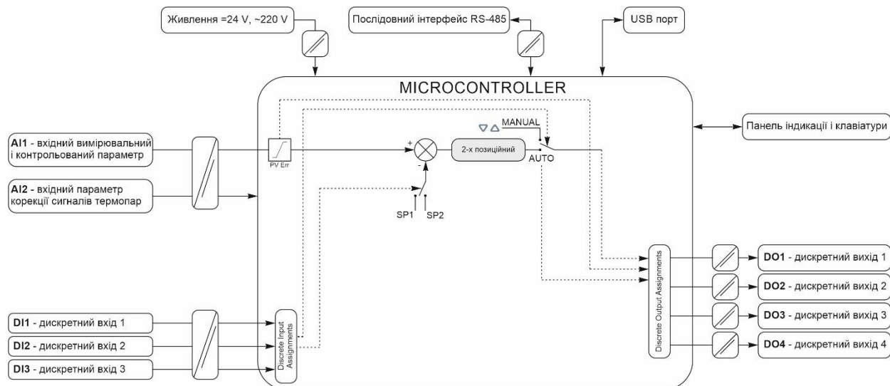
Рисунок 4.1 - Структурна схема регулятора МІК-311-К11 в режимі роботи 2-х позиційного регулятора
