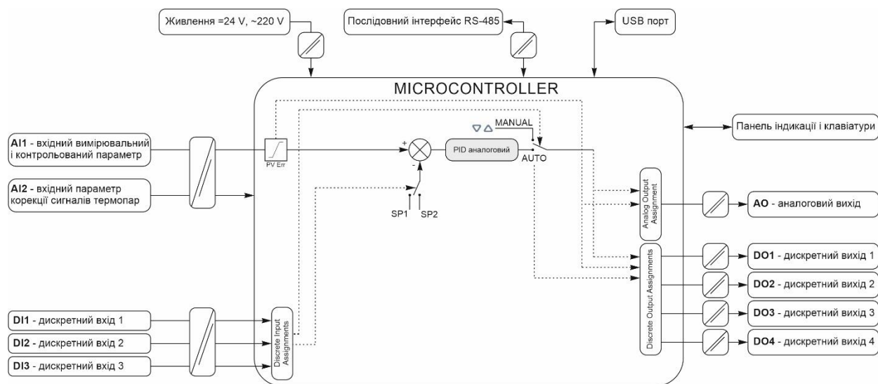
Рисунок 4.6 - Структурна схема регулятора MIK-311-K11 в режимі ПІД-аналогового регулятора
