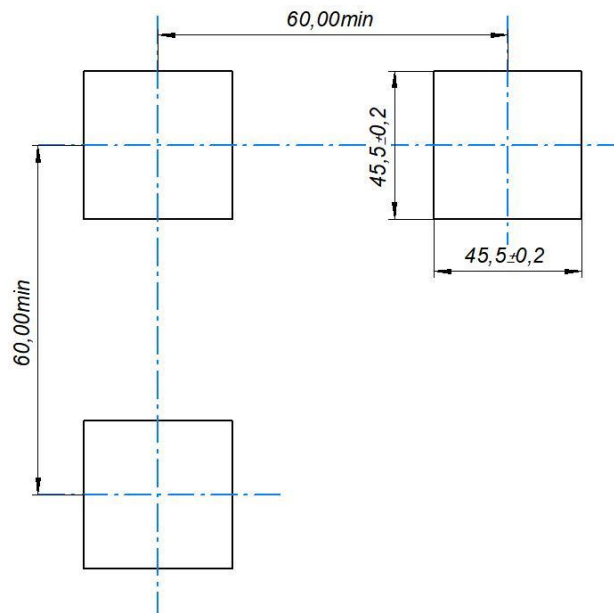
Рисунок А.3 – Розмітка отворів на щиті для встановлення регулятора
