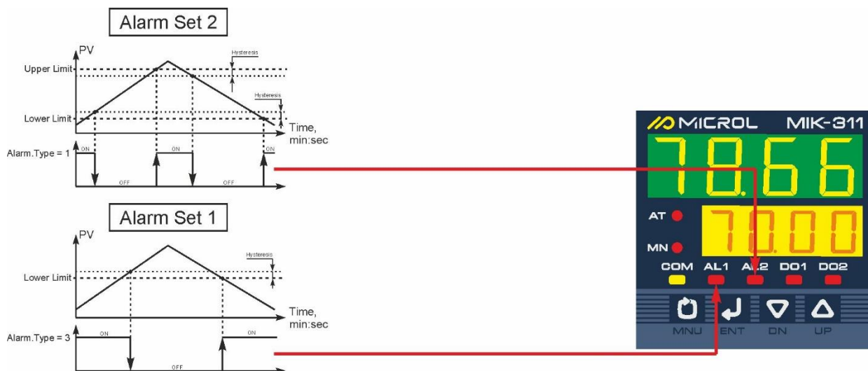
Рисунок 4.10 – Принцип роботи сигналізації
