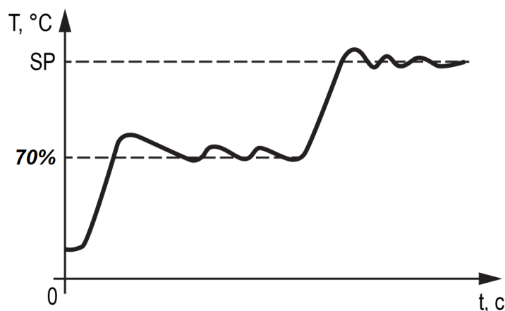
Рисунок 3.3 – Процес автоналаштування
