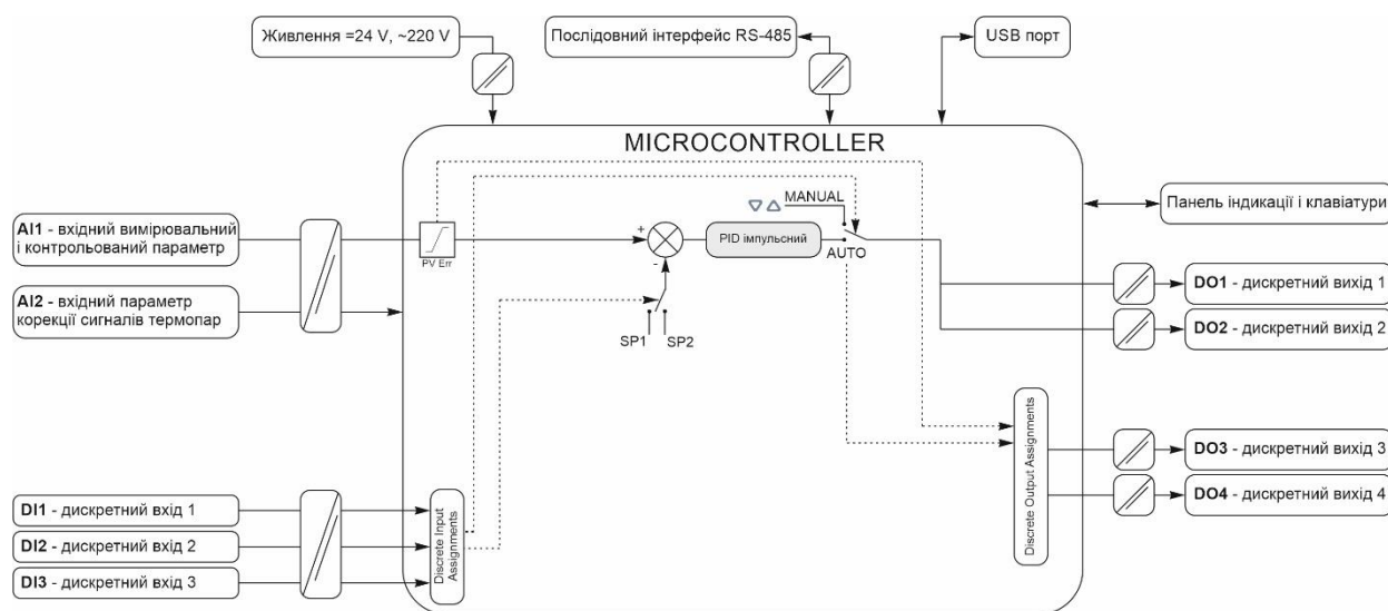
Рисунок 4.8 - Структурна схема регулятора МІК-311-К11 в режимі роботи ПІД імпульсного регулятора
