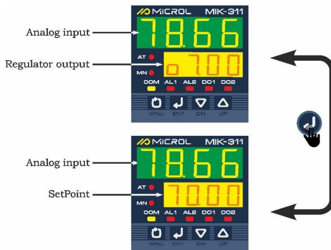
Рисунок 3.2 – Діаграма відображення режиму РОБОТА
