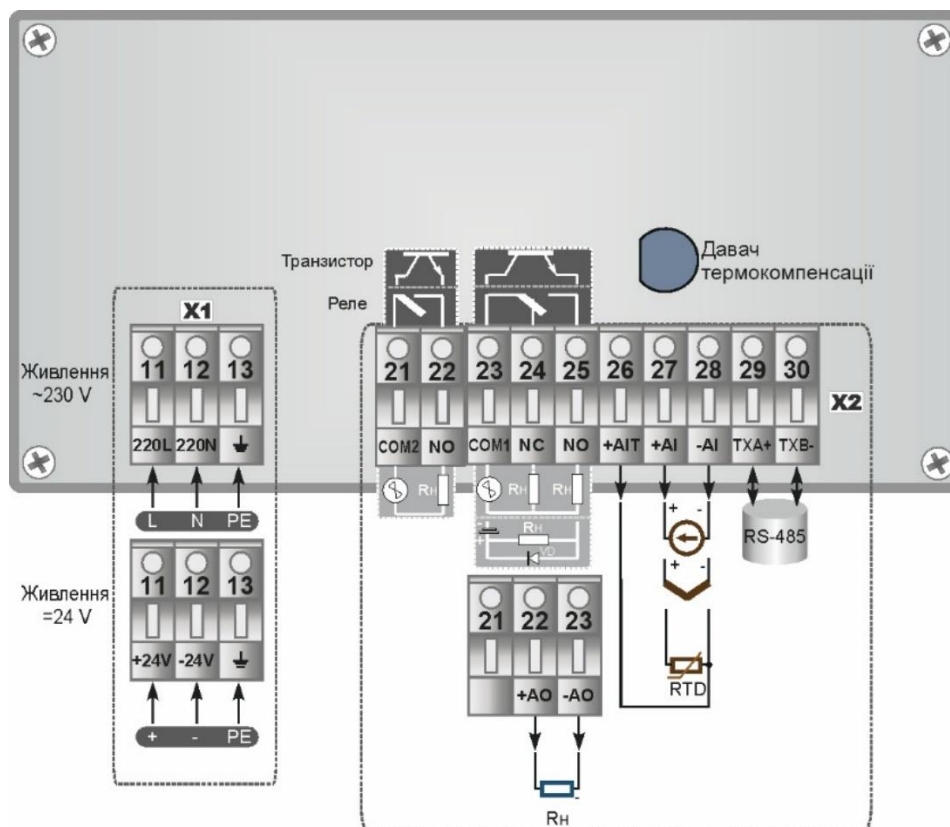
Рисунок Б.2 - Схема зовнішніх з'єднань індикатора ITM-300A
