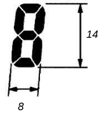
Рисунок А.1 – Зовнішній вигляд індикатора ITM-300A та розміри цифрових індикаторів (тип індикаторів - 0)
