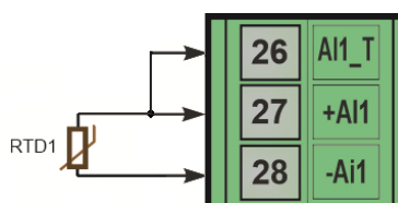
Рисунок Б.2.2 – Двох провідна схема підключення термоопорів
