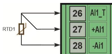
Рисунок Б.2.1 – Трьох провідна схема підключення термоопорів
