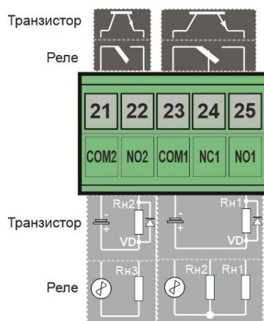
Рисунок Б.3.1 - Підключення дискретних навантажень до індикатора ITM-300A
