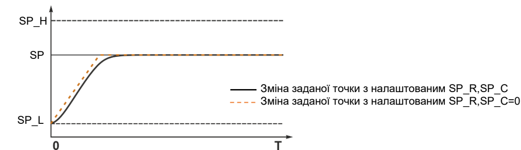
Рисунок 3.2 - Графік роботи «Постійна часу фільтра заданої точки»
