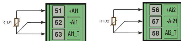
Рисунок Б.2.1 – Трьох провідна схема підключення термоопорів
