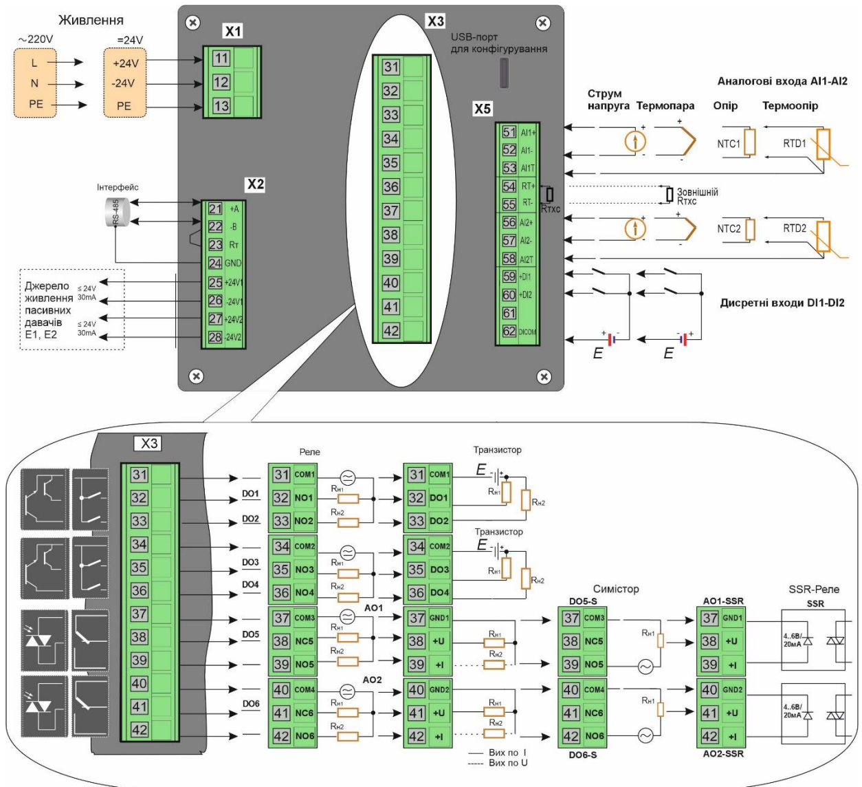
Рисунок Б.1 – Схема зовнішніх з'єднань регулятора MIK-322-K7
