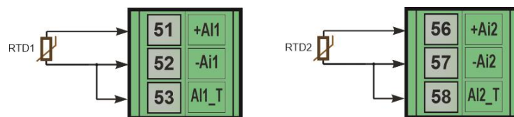
Рисунок Б.2.2 – Двох провідна схема підключення термоопорів
