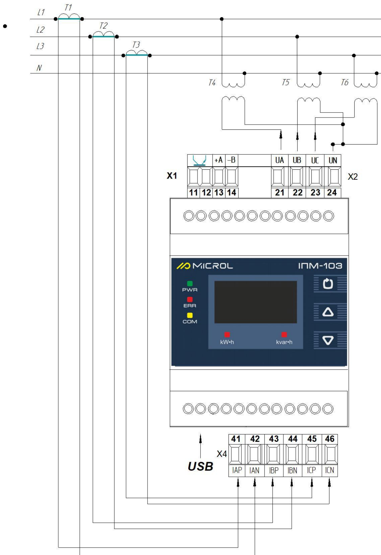
Рисунок Б.3 - Підключення зовнішніх ланцюгів індикатора ІПМ-103 трьох фазної мережі через трансформатори струму і трансформатори напруги.
