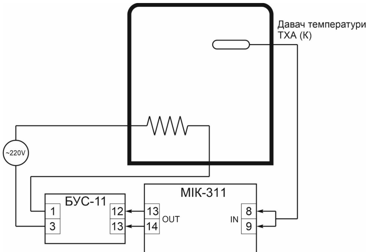
Рисунок 4.11 – Схема та процес термічної обробки
