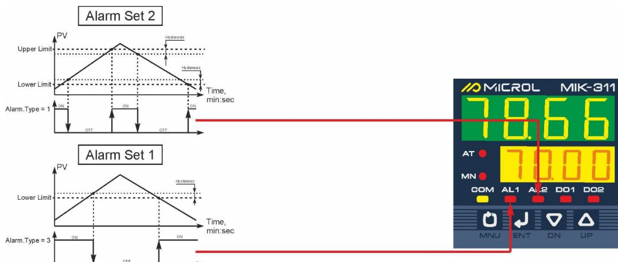
Рисунок 4.9 – Принцип роботи сигналізації
