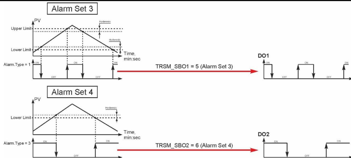
Рисунок 4.10 – Приклад налаштування роботи дискретних виходів
