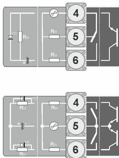
Рисунок Б.4 - Підключення дискретних навантажень до регулятора MIK-311-K11
