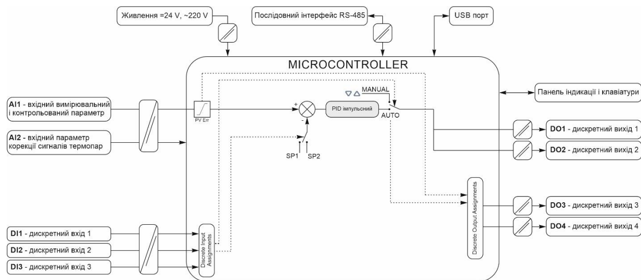
Рисунок 4.8 - Структурна схема регулятора МІК-311-К11 в режимі роботи ПІД імпульсного регулятора
