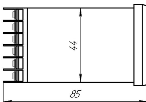
Рисунок А.2 – Габаритні розміри регулятора
