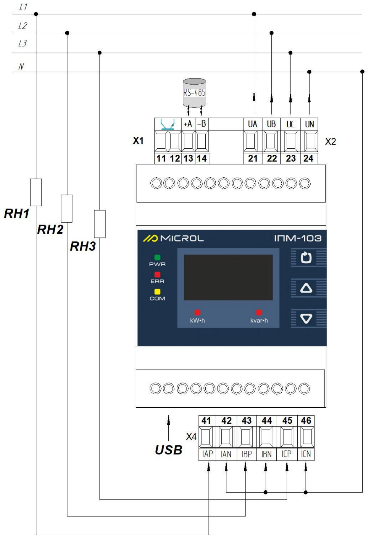
Рисунок Б.1 - Підключення зовнішніх ланцюгів індикатора ІПМ-103 до трьох фазної мережі.
