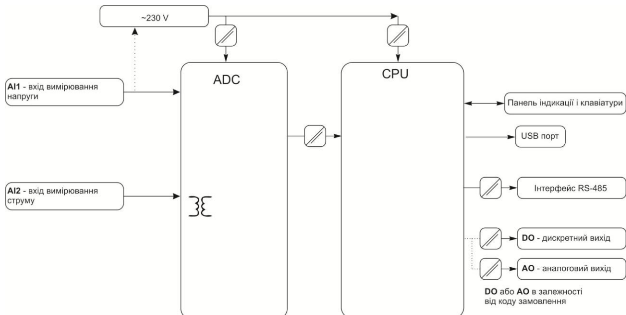
Рисунок 3.4 - Структурна схема iндикатора IПМ-101
