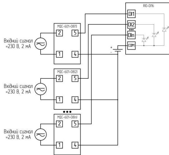
Рисунок 2 – Приклад підключення декількох модулів МДС-601 до модуля RIO-DI16
