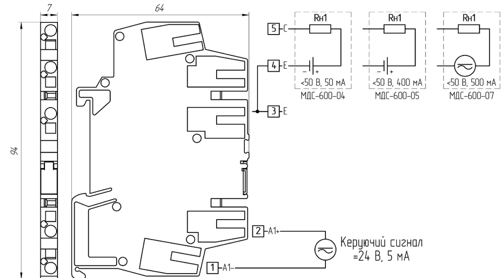
Рисунок 1 – Габаритні розміри та схема зовнішніх з'єднань модуля
