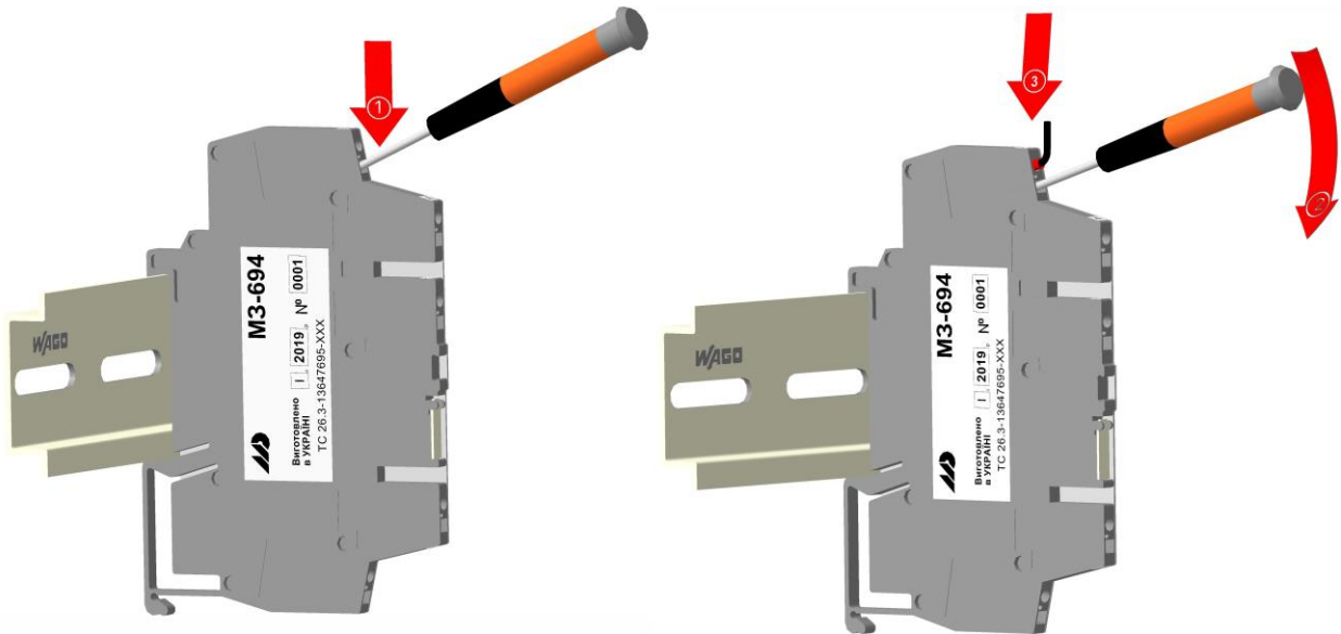
Рисунок 3.2 - Схема установки дротів за допомогою плоскої викрутки
