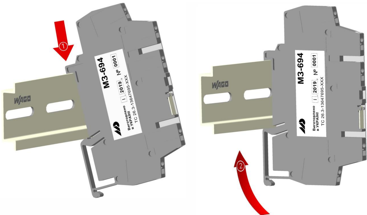
Рисунок 3.1 - Схема кріплення модуля M3-694 на DIN-рейку
