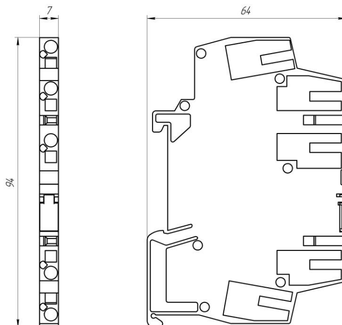
Рисунок 1.1 - Зовнішній вигляд і габаритні розміри модуля МЗ-694
