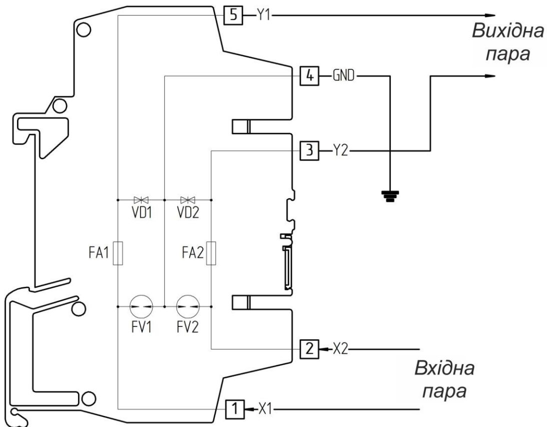
Рисунок 3.3 - Схема зовнішніх з'єднань перетворювача БП-694
