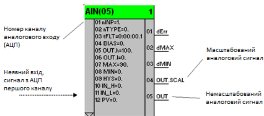
Рисунок 2.3 - Функціональний блок аналогового вводу з неявними входами
