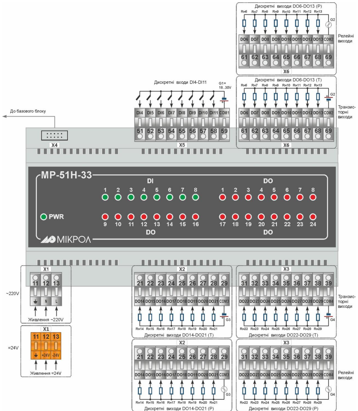
Рисунок 8.2.10 - Схема зовнішніх з'єднань модуля розширення MP-51H-33
