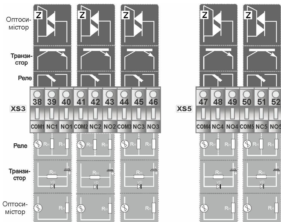
Рисунок 8.1.3 - Схема підключення дискретних виходів контролера MIK-51H
