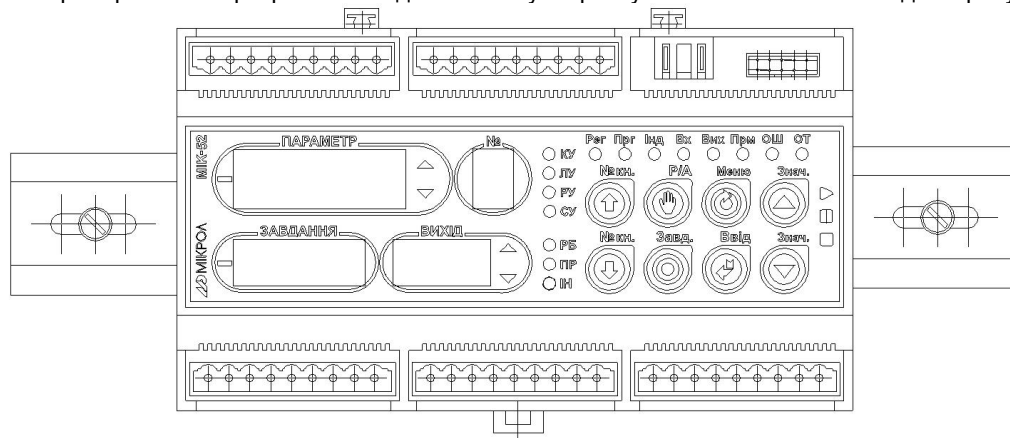
Рисунок 7.1 - Положення МІК-51Н при монтажі на DIN-Рейку
