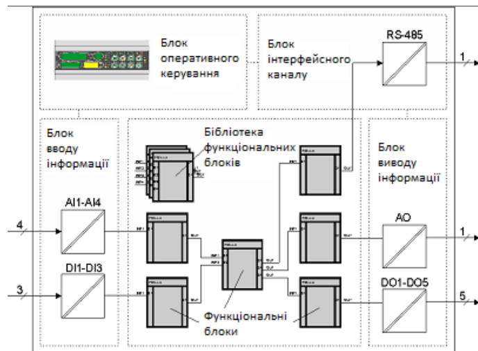
Рисунок 2.1 - Архітектура контролера MIK-51
