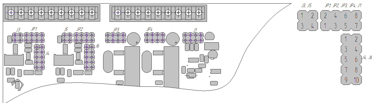
Рисунок 8.1.1 - Положення перемичок аналогових входів
