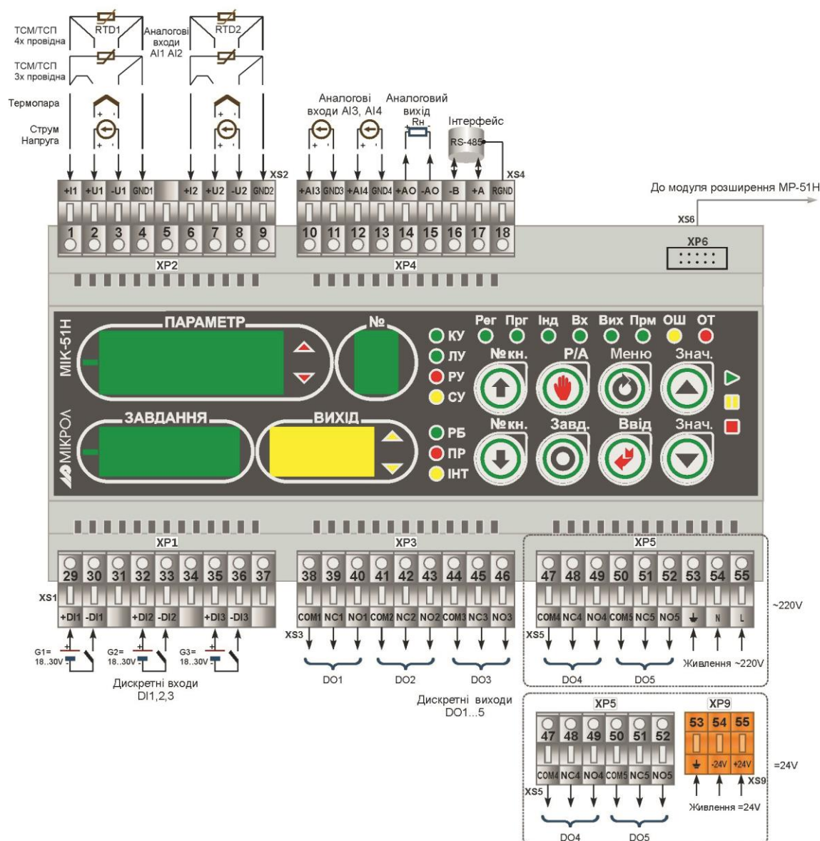
Рисунок 8.1 - Нумерація клем і сигнали контролера MIK-51H
