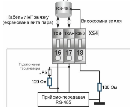
Рисунок 8.1.5 - Схема підключення інтерфейсу
