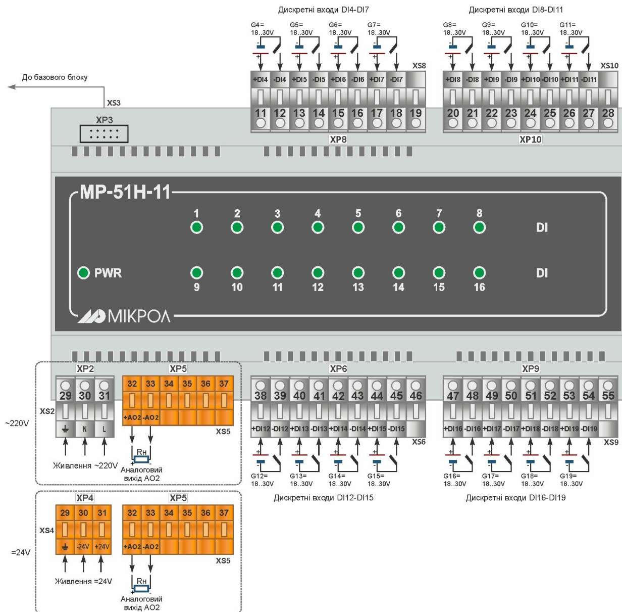
Рисунок 8.2.1 - Нумерація клем і сигнали модуля розширення MP-51H-11
