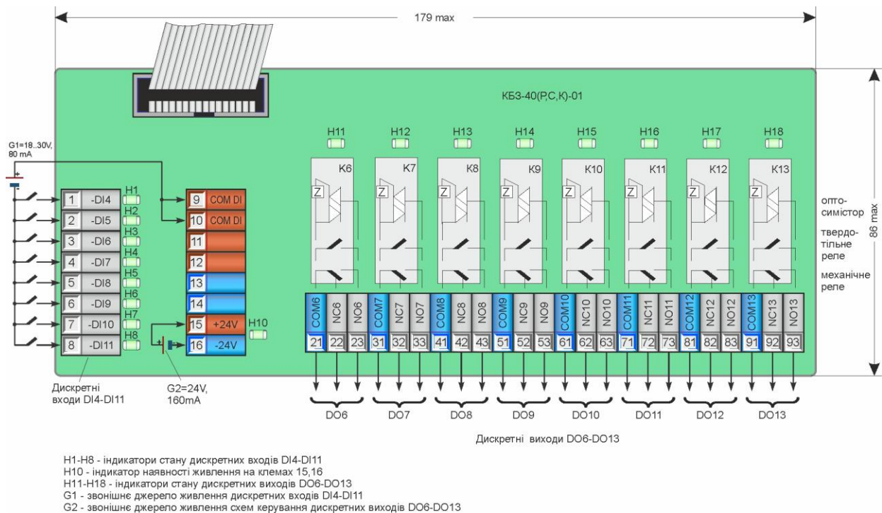
Рисунок 8.4.10 - Підключення сигналів модуля розширення МР-52-12 (МР-51-12) за допомогою клемно-блочного з'єднувача КБ3-40(Р,С,К)-01
