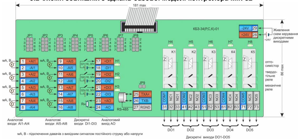
Рисунок 8.2.1 - Підключення клемно-блокового з'єднувача КБ3-34(Р,С,К)-01 до контролера МІК-52
