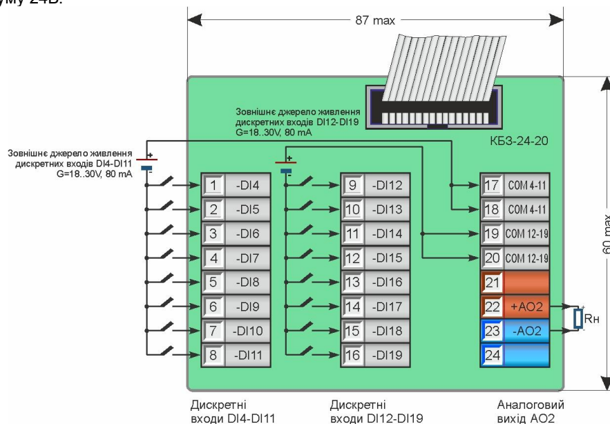
Рисунок 8.4.8 - Підключення сигналів модуля розширення MP-52-11 (MP-51-11) за допомогою клемно-блочного з'єднувача KB3-24-20
