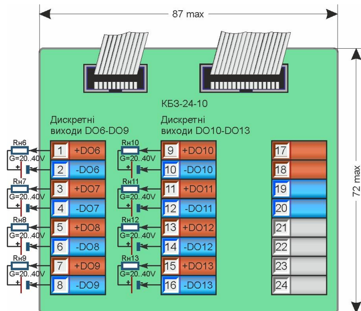
Рисунок 8.4.2 - Підключення сигналів модуля розширення MP-52-03 (MP-51-03) за допомогою клемно-блочного з'єднувача KB3-24-10
