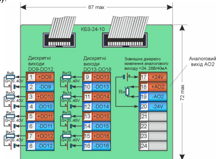
Рисунок 8.4.5 - Підключення сигналів модуля розширення MP-52-06 (MP-51-06) за допомогою клемно-блочного з'єднувача КБ3-24-10
