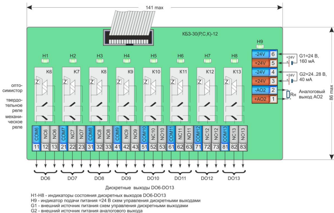
Рисунок 8.4.6 - Підключення сигналів модуля розширення MP-52-06 (MP-51-06) за допомогою клемно-блочного з'єднувача КБ3-30 (Р, С, К) -12
