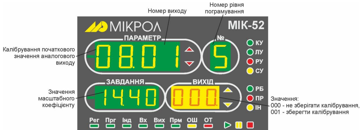
Рисунок 9.4.2.1 - Зовнішній вигляд індикаторів при калібруванні нуля аналогового виходу
