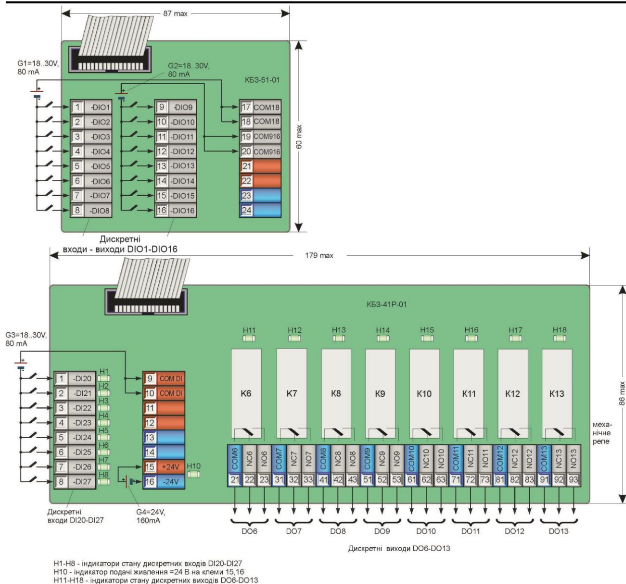
Рисунок 8.4.17 - Підключення сигналів модуля розширення MP-52-31 за допомогою клемно-блочного з'єднувача KB3-41P-01 (KB3-51-01 + KB3-40P-01)
