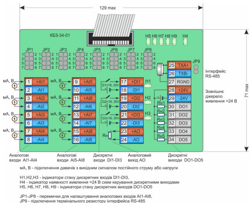
Рисунок 8.2.2 - Підключення клемно-блокового з'єднувача КБ3-34-01 до контролера МІК-52
