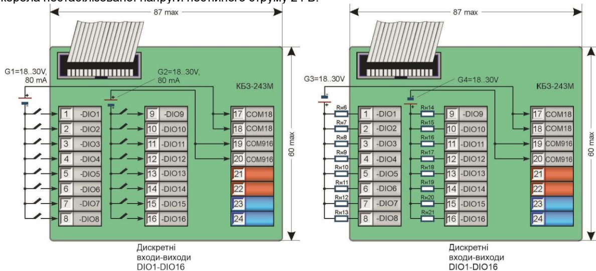
Рисунок 8.4.22 - Підключення сигналів модуля розширення MP-52-34 за допомогою клемно-блокових з'єднувачів КБ3-51-01 (КБ3-243М+КБ3-243М)
