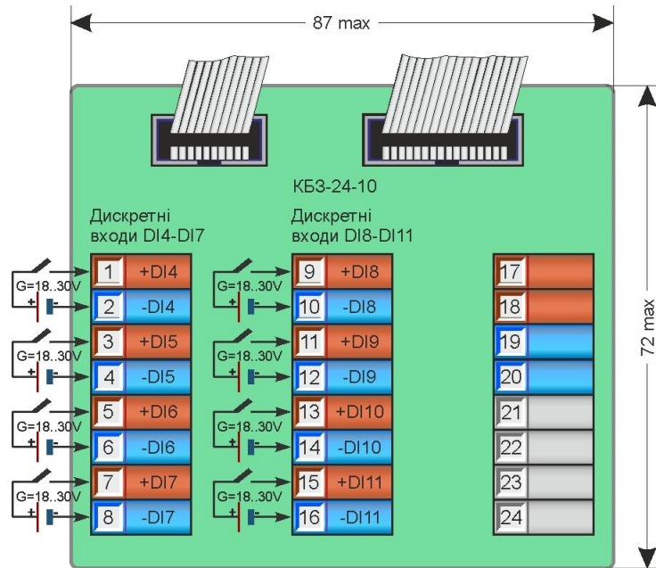
Рисунок 8.4.1 - Підключення сигналів модуля розширення MP-52-01 (MP-51-01) за допомогою клемно-блочного з'єднувача KB3-24-10
