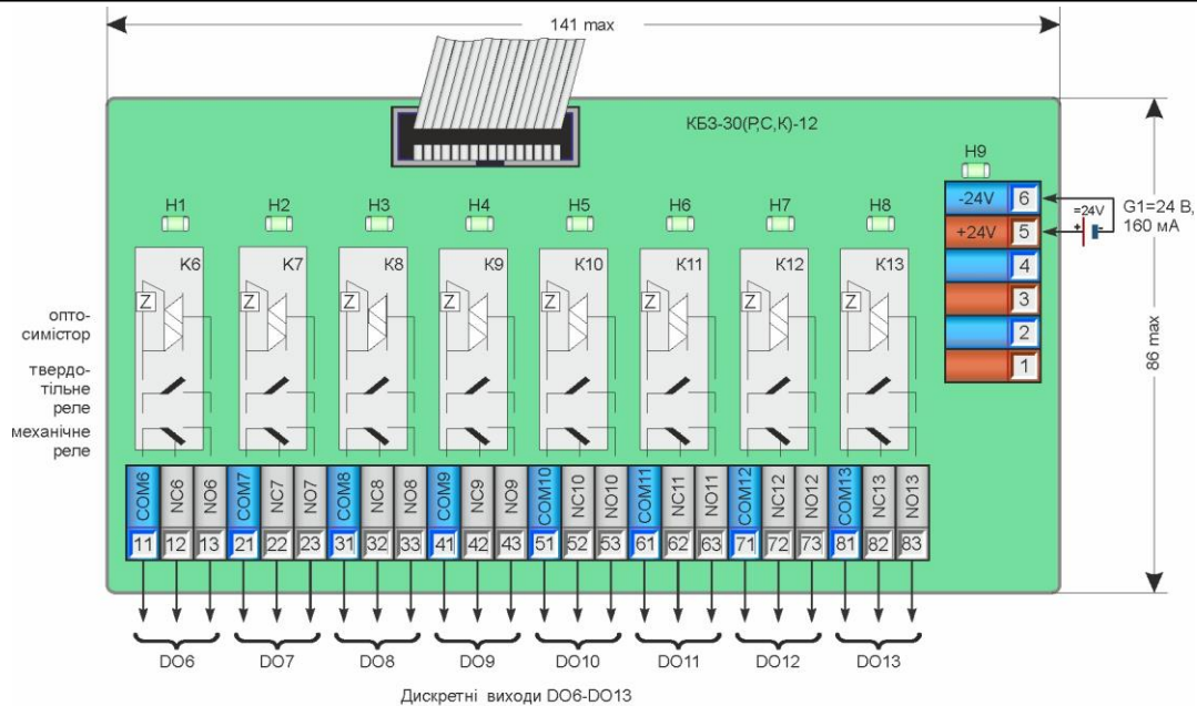
Рисунок 8.4.3 - Підключення сигналів модуля розширення MP-52-03 (MP-51-03) за допомогою клемно-блочного з'єднувача KB3-30(P,C,K)-12
