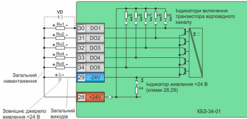
Рисунок 8.3.3 - Підключення дискретних виходів за допомогою клемно-блочного з'єднувача КБ3-34-01
