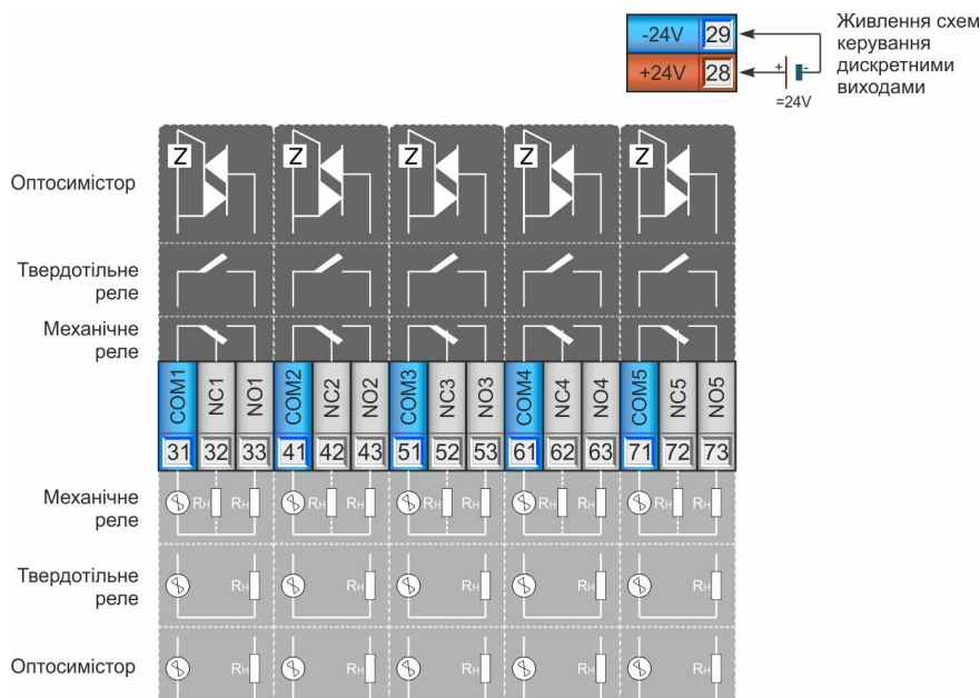
Рисунок 8.3.2 - Підключення дискретних виходів за допомогою клемно-блочного з'єднувача КБЗ-34 (Р, С, К) -01
