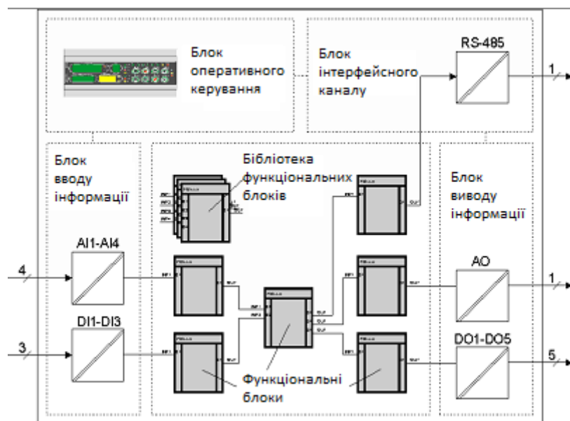
Рисунок 2.1 - Архітектура контролера MIK-52
