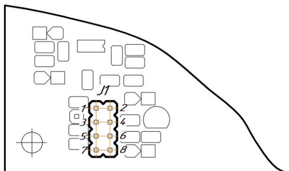
Рисунок 8.3.1 - Положення перемичок на платі контролера MIK-52
