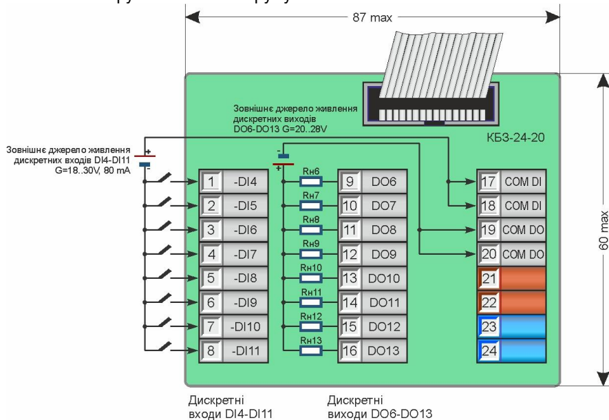
Рисунок 8.4.9 - Підключення сигналів модуля розширення МР-52-12 (МР-51-12) за допомогою клемно-блочного з'єднувача КБ3-24-20
