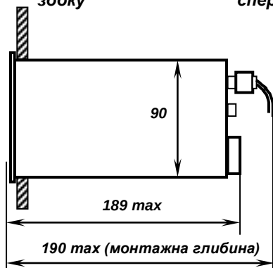
Вид збоку
