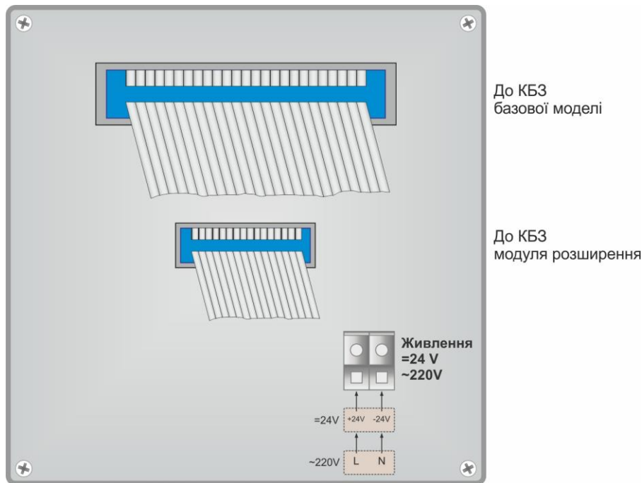
Рисунок 8.1.1 - Зовнішній вигляд задньої стінки контролера МІК-52 при підключенні до нього модулів розширення МР-51-01 ... 15 (контролер, випущений до 2016 року включно)
