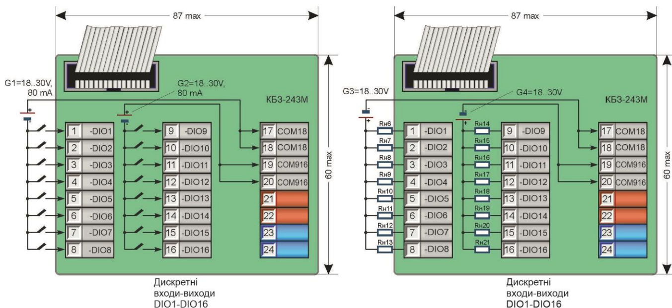
Рисунок 8.4.15 - Підключення сигналів модуля розширення MP-52-30 за допомогою клемно-блокових з'єднувачів КБ3-51-01(КБ3-243М+КБ3-243М)
