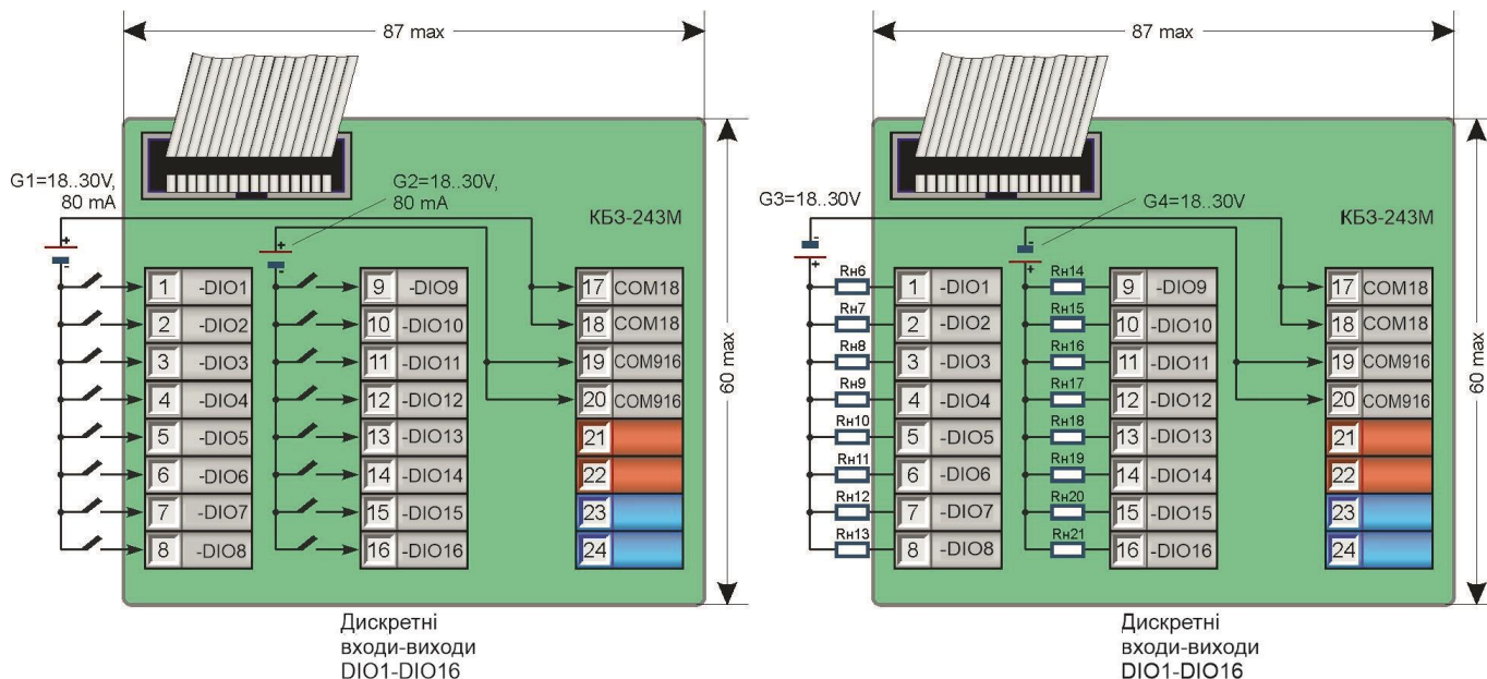
Рисунок 8.4.16 - Підключення сигналів модуля розширення MP-52-31 за допомогою клемно-блокових з'єднувачів КБ3-51-01 (КБ3-243М+КБ3-243М)
