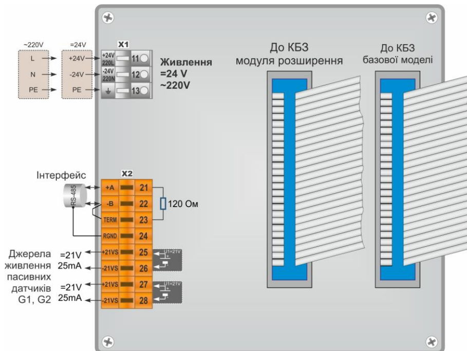
Рисунок 8.1.2 - Зовнішній вигляд задньої стінки контролера МІК-52 при підключенні до нього модулів розширення МР-52-30 ... 34 (контролер, випущений після 2016 року)
