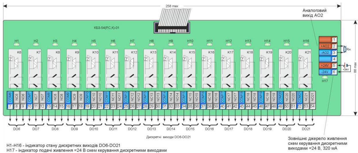
Рисунок 8.4.14 - Підключення сигналів модуля розширення MP-52-15 (MP-51-15) за допомогою клемно-блочного з'єднувача КБ3-54 (Р,С,К)-01
