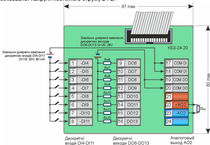
Рисунок 8.4.11 - Підключення сигналів модуля розширення МР-52-13 (МР-51-13) за допомогою клемно-блокового з'єднувача KB3-24-20
