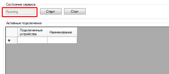
Рисунок 7.1.5 - Сервер запущено
