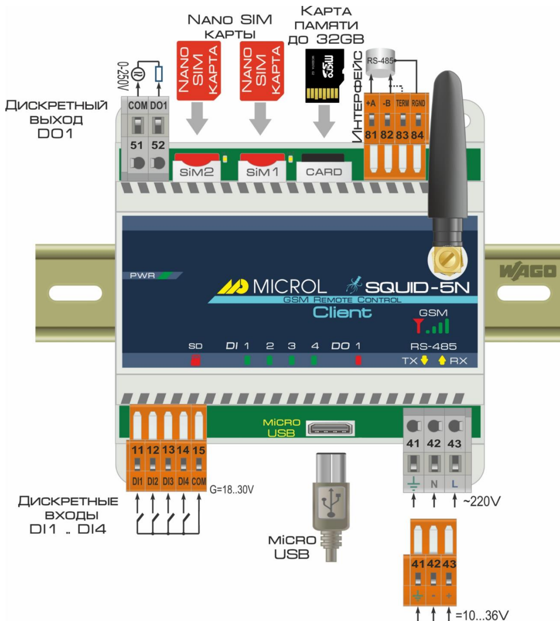
Рисунок А – Схема зовнішніх з'єднань GSM-контролера Squid-5N-Client
