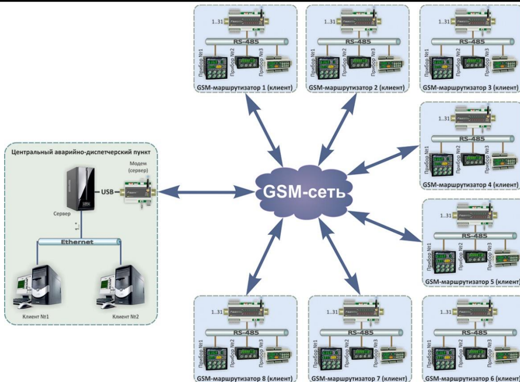
Рисунок 1.2 – Схема системи зі Squid-1H як сервер вісьмома віддаленими GSM-контролерами Squid-5N-Client
