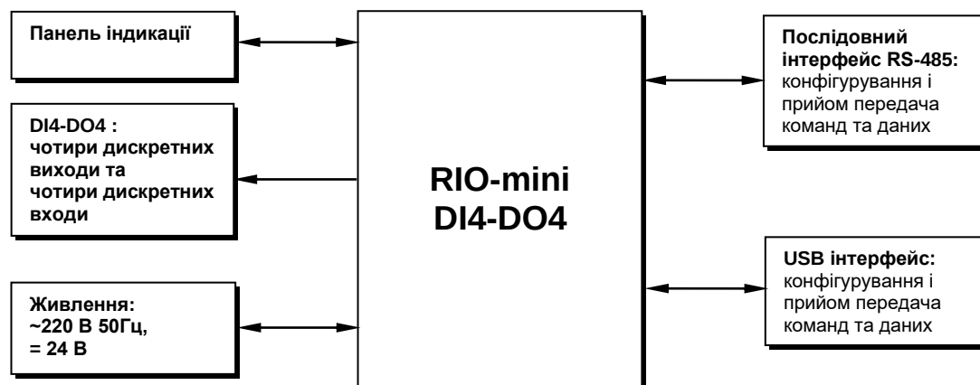
Малюнок 3.1 – Структурна схема модуля RIO-mini DI4-DO4
