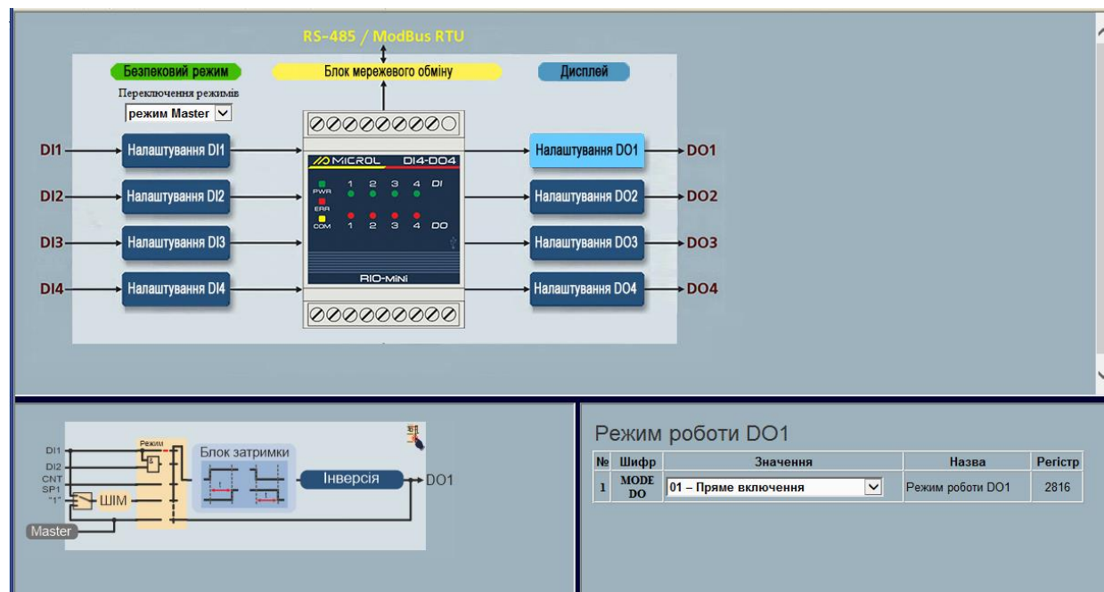
Малюнок 4.2 – Вікно налаштування дискретного виходу DO1
