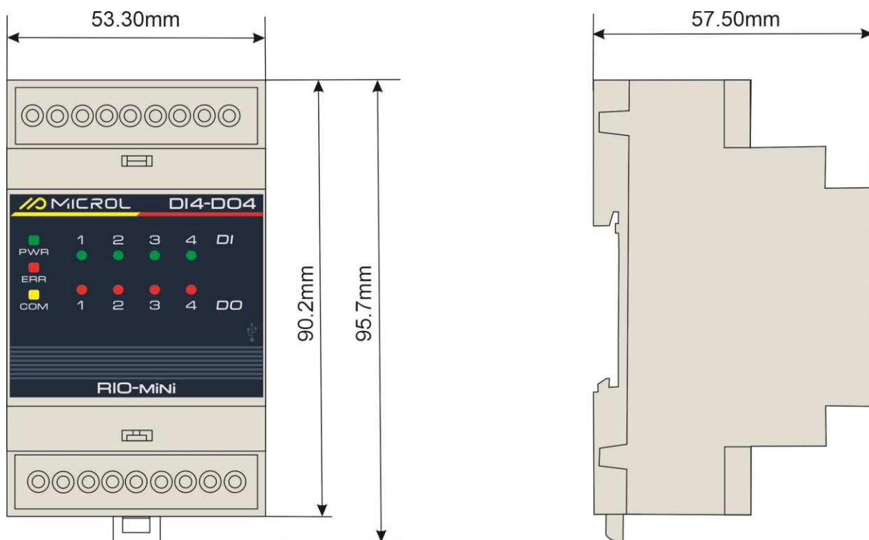
Малюнок А.2 - Габаритні розміри RIO-mini DI4-DO4
