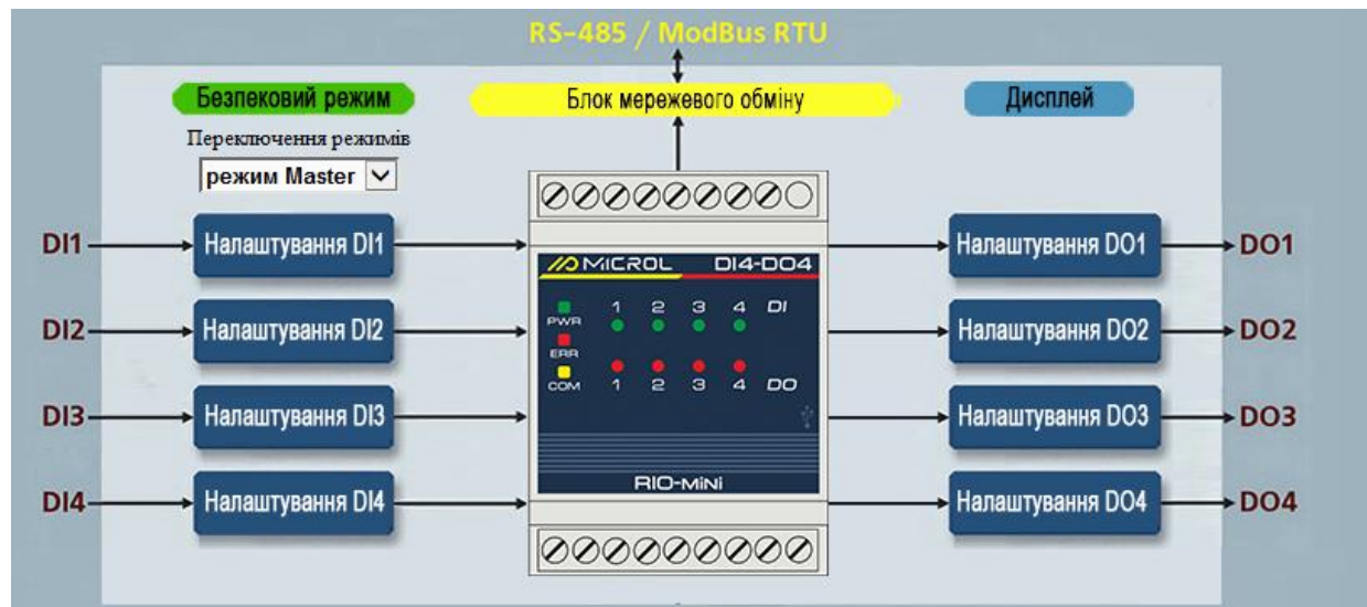
Малюнок 4.1 – Початковий екран RIO-mini DI4-DO4 в програмі MIK-Programmer
