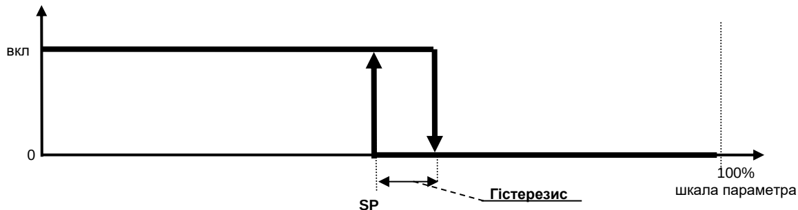
Рисунок 3.7 – Приклад роботи вихідного пристрою з логіки зворотного 2-х позиційного управління п.10.03 = 0005, п. 10.04 = 0000
