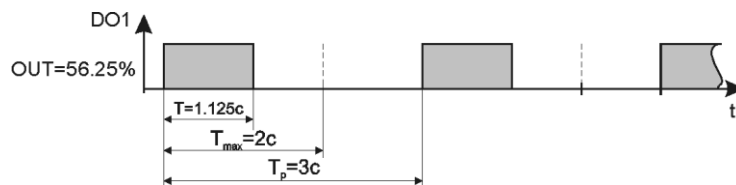
Рисунок 3.6 – Графік формування виходу П-регулятора
