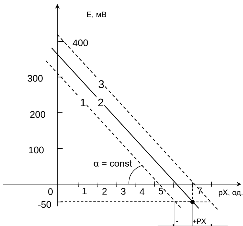
Рисунок 3.12-Корекція зміщення pX_{CM} електродної характеристики
