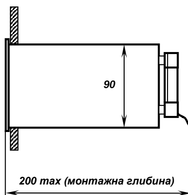
Рисунок А.2-габаритні розміри
