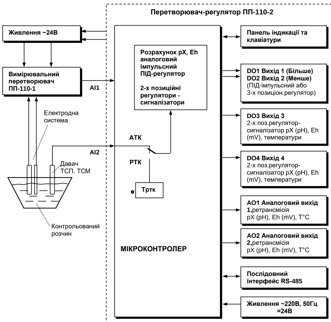
Рисунок 3.2-Структурна схема мікропроцесорного перетворювача-регулятора потенціометричного ПП-110-2, у комплекті з вимірювальним перетворювачем ПП-110-1
