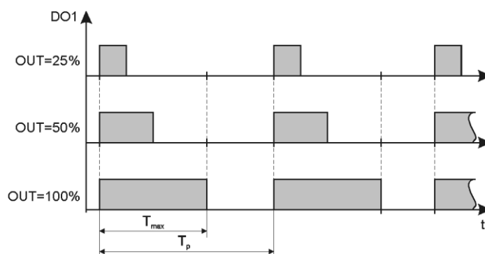
Рисунок 3.5 – Графік формування імпульсного виходу П-регулятора
