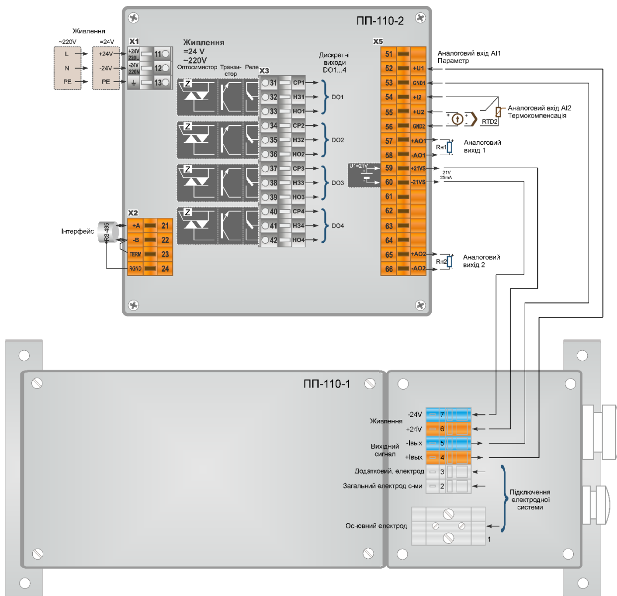
Рисунок Б.8 – Схема підключення приладів
