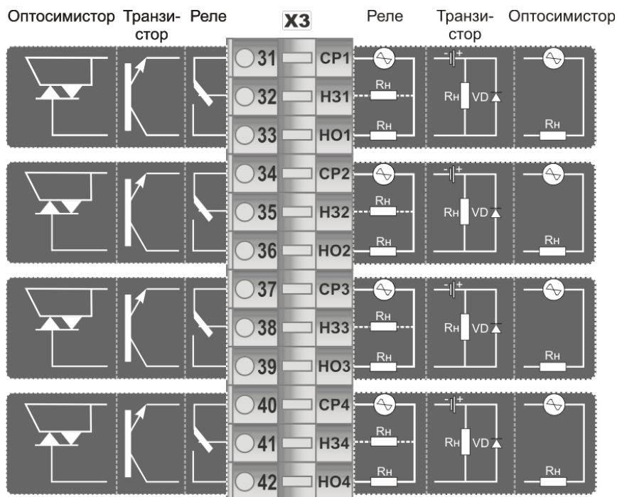
Рисунок Б.4-Підключення дискретних навантажень до перетворювача ПП-110
