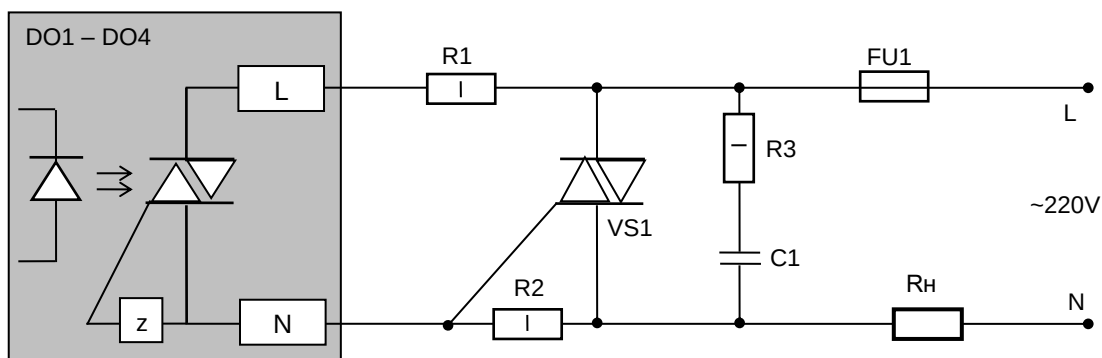
Рисунок Б.6 – Схема підключення зовнішнього симістора
