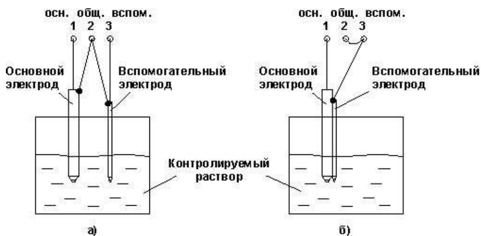
Рисунок Б.3-Підключення електродної системи до вимірювального перетворювача ПП-110-1
