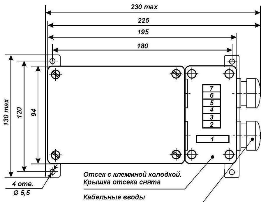
Рисунок А.4-Габаритні розміри ПП-110-1
