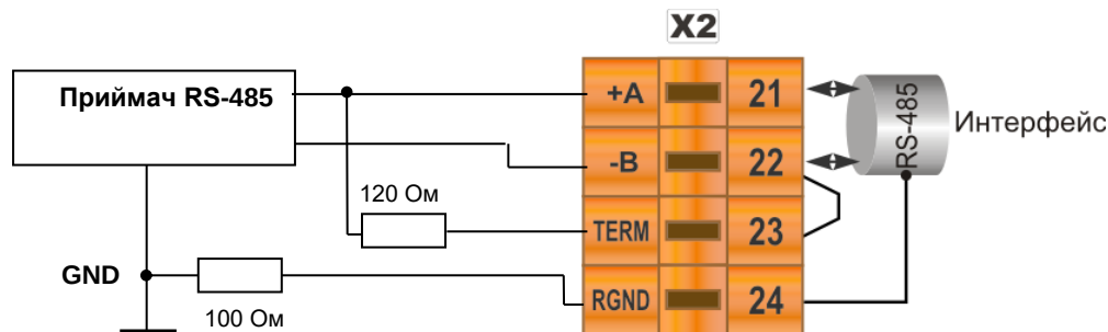
Рисунок Б.10-Рекомендована схема підключення інтерфейсу RS-485
