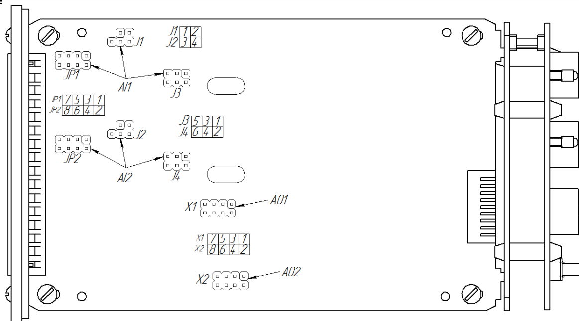
Рисунок 4.5 – Положення перемичок на платі процесора
