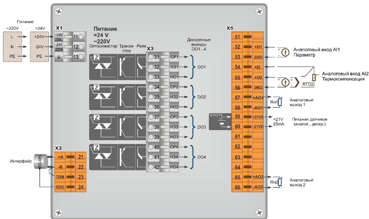
Рисунок Б.2 – Схема зовнішніх з'єднань перетворювача ПП-110-2
