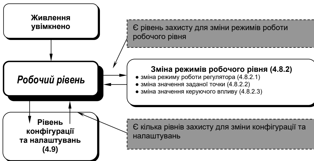
Рисунок 4.1-Діаграма рівнів роботи, захисту та налаштувань перетворювача-регулятора ПП-110
