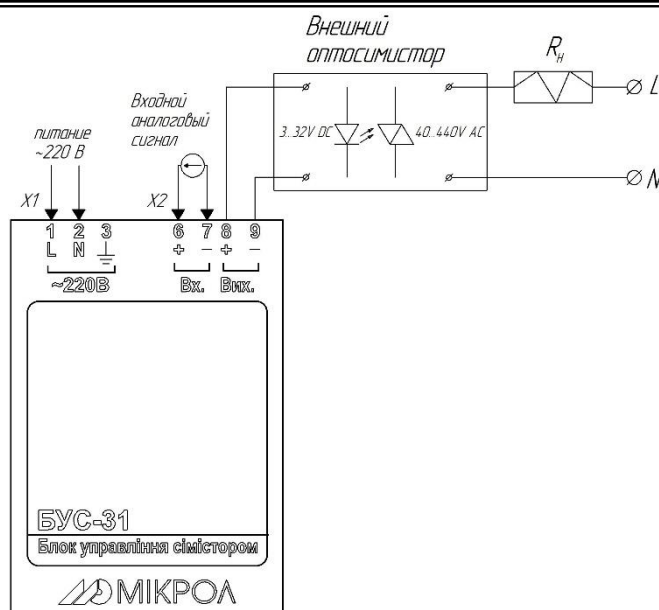
Рисунок 4.2.2 – Схема зовнішніх з'єднань блоку БУС-31
