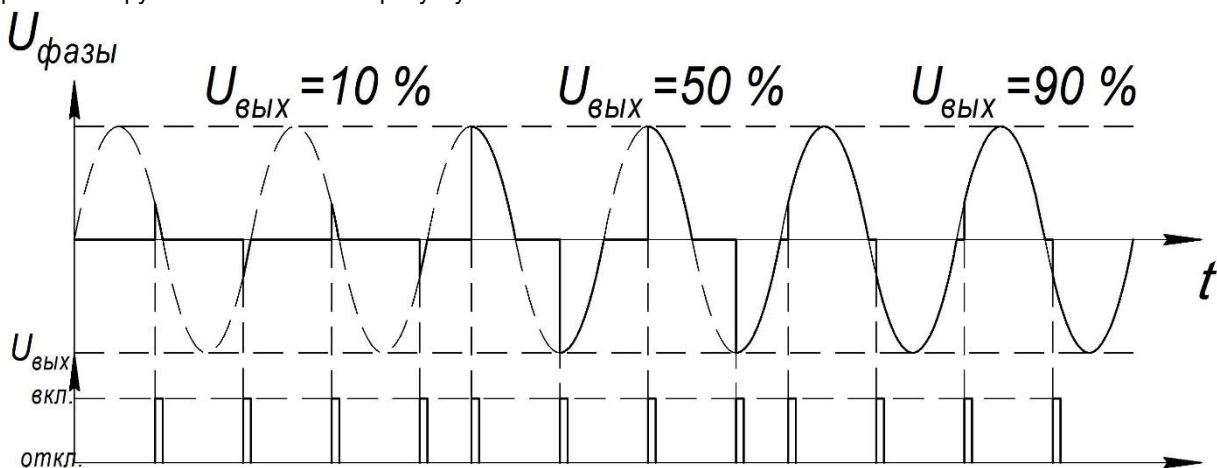
Рисунок 2.1 – Принцип роботи блоку БУС-31
