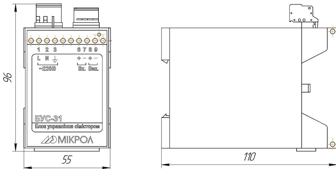
Рисунок 1.4– Зовнішній вигляд та габаритні розміри блоку БУС-31
