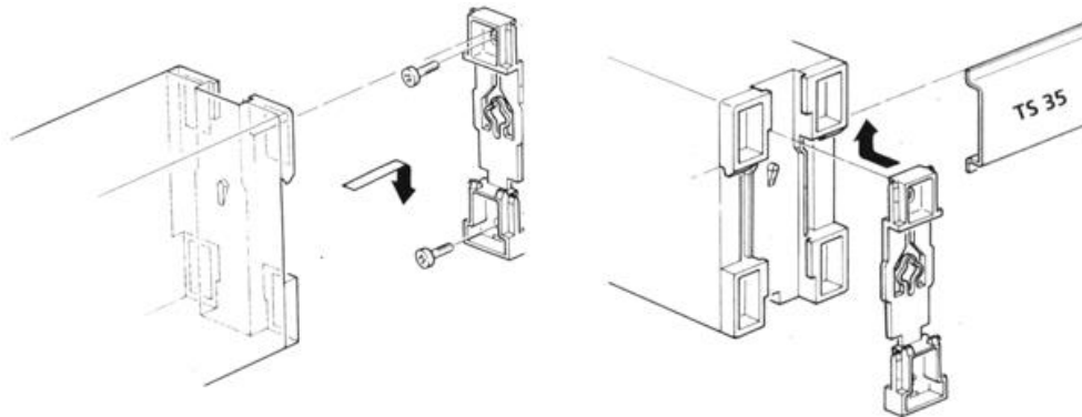
Рисунок 4.2.1 – Схема кріплення блоку БУС-31 на DIN-рейці
