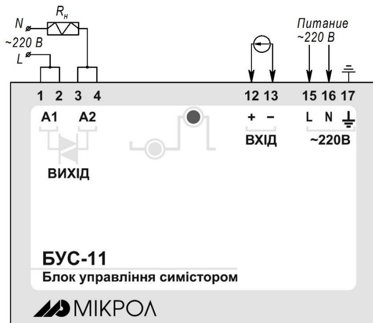
Рисунок 4.2.2 – Схема зовнішніх з'єднань блоку БУС-11
