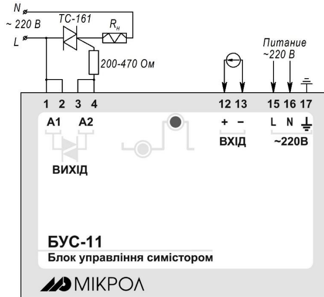
Рисунок 4.2.3 – Схема зовнішніх з'єднань БУС-11 для керування зовнішнім симістором (тиристором)
