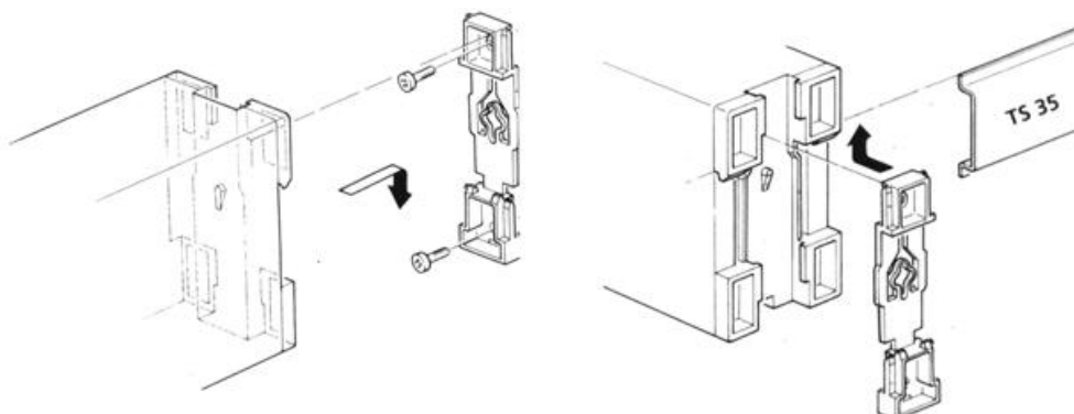
Рисунок 4.2.1 – Схема кріплення блоку БУС-11 на DIN-рейці
