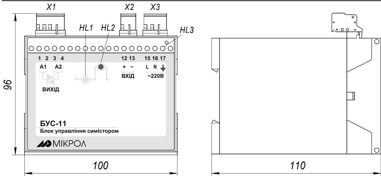
Рисунок 1.4– Зовнішній вигляд та габаритні розміри блоку БУС-11
