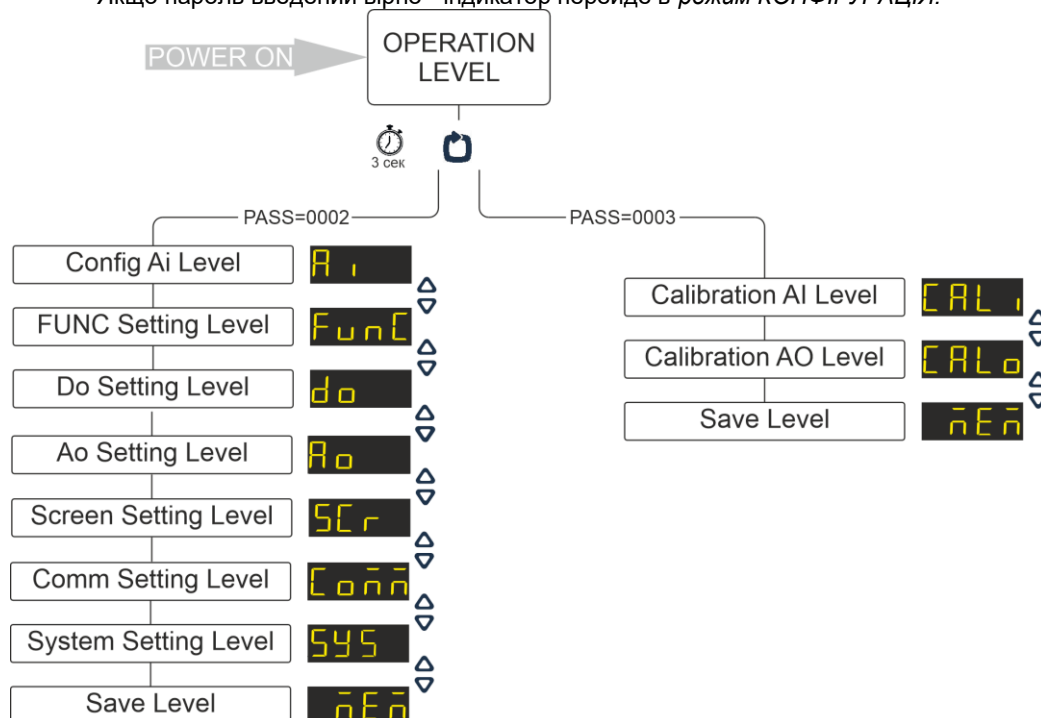
Рисунок 4.16 – Діаграма режиму конфігурації індикатора
