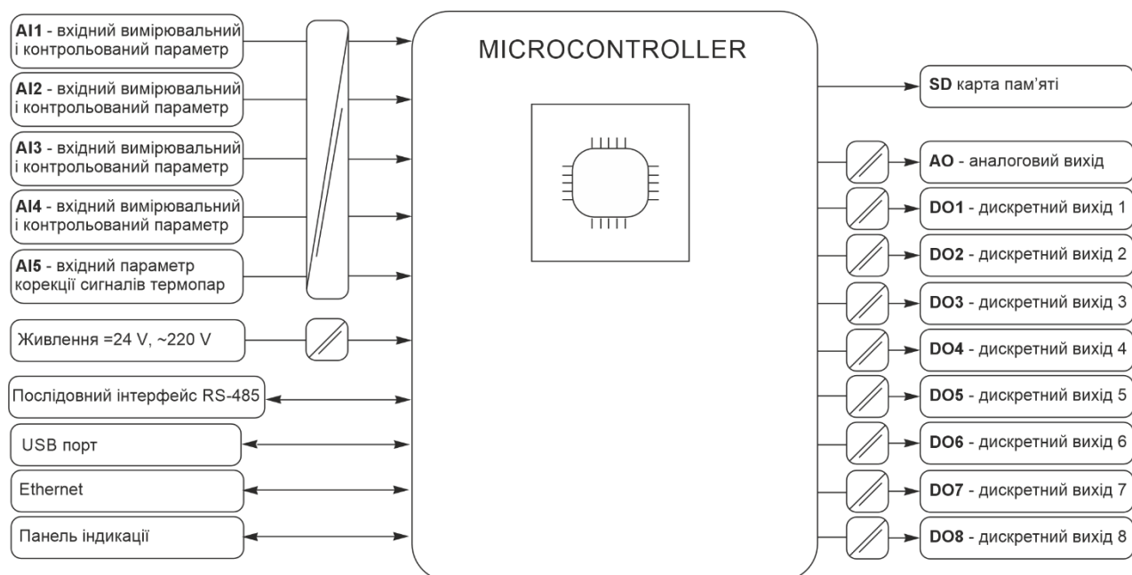
Рисунок 3.2 - Структурна схема індикатора ITM-304
