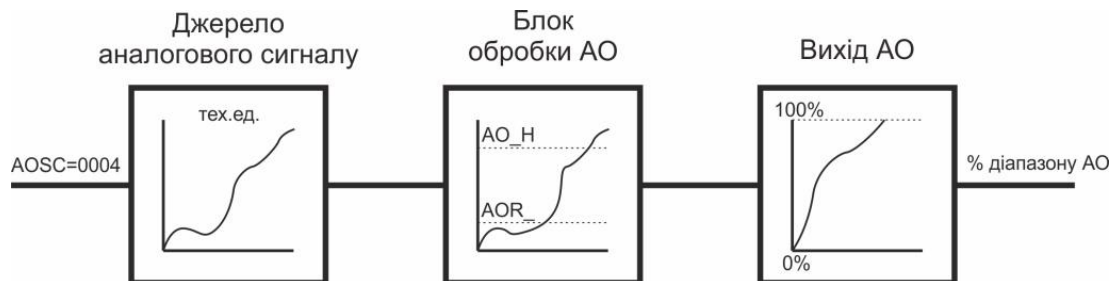
Рисунок 3.5- Робота блоку аналогового виведення в режимі перетворення
