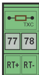
Рисунок Б.2.4 – Схема підключення датчика термокомпенсації
