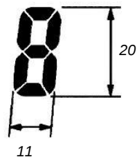
Рисунок А.1 – Зовнішній вигляд індикатора ITM-304 та розміри цифрових індикаторів(тип індикаторів - 0)
