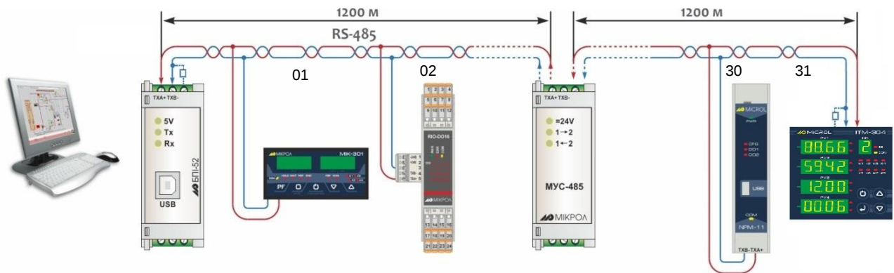
Рисунок Б.4.1 - Організація інтерфейсного зв'язку між комп'ютером і перетворювачами
