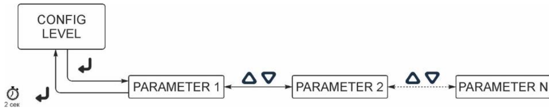
Рисунок 4.17 – Перехід між конфігураційними параметрами індикатора ITM-304
