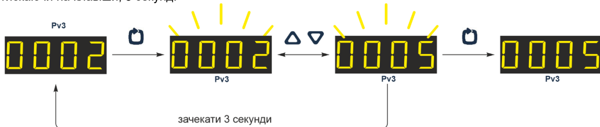
Рисунок 4.18 – Фіксація та відміна зміни параметру індикатора ITM-304
