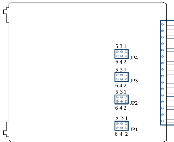
Рисунок 4.20 - Положення перемичок на платі приладу
