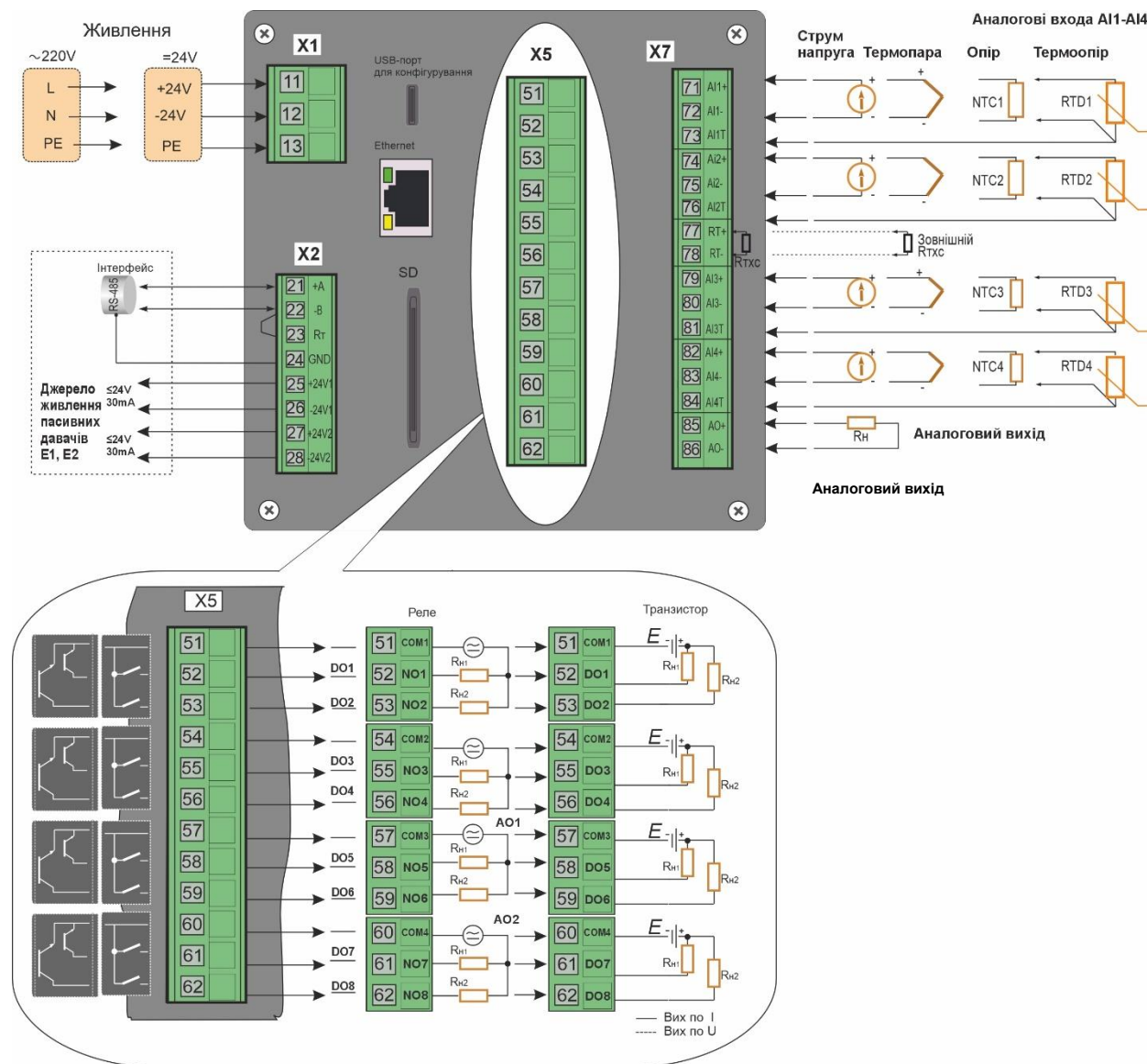
Рисунок Б.1 - Схема зовнішніх з'єднань індикатора ITM-304
