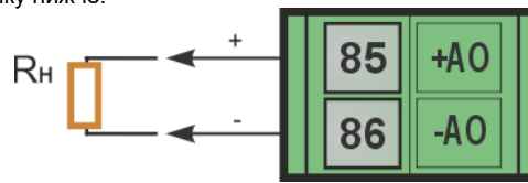
Рисунок Б.3.3– Схема підключення виходу постійної напруги
