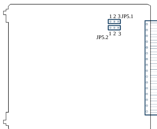
Рисунок 4.21 - Положення перемичок на платі приладу
