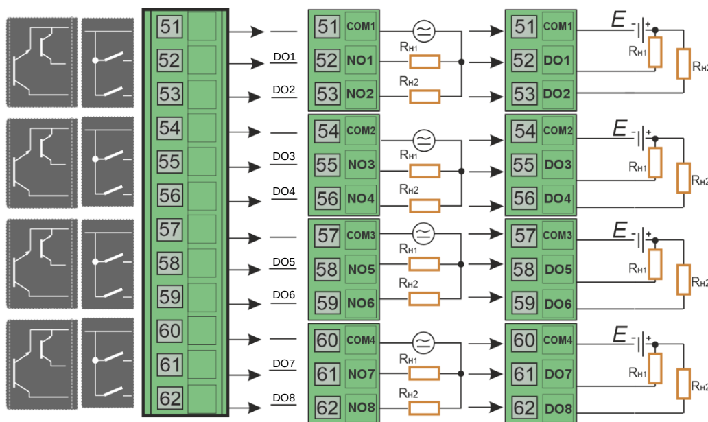
Рисунок Б.3.1 - Підключення дискретних навантажень до індикатора ITM-304
