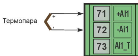
Рисунок Б.2.3 – Схема підключення термопар
