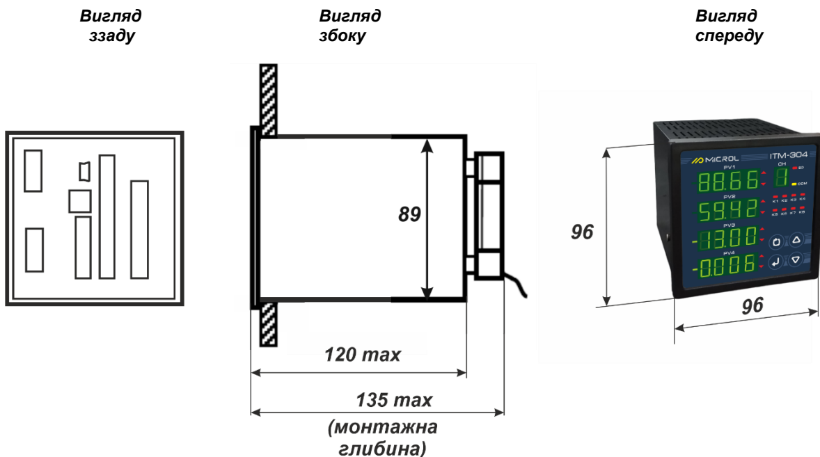
Рисунок А.2 – Габаритні розміри індикатора
