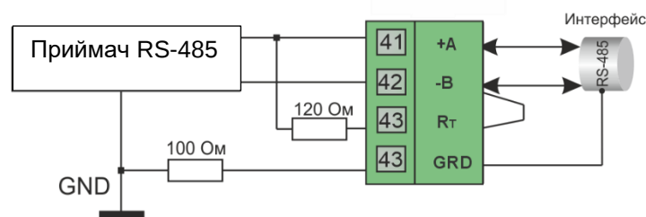
Рисунок Б.4.2 - Рекомендована схема підключення інтерфейсу RS-485
