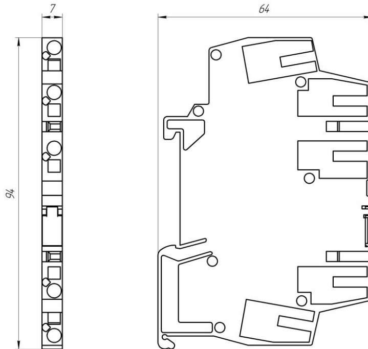
Рисунок 1.1 - Зовнішній вигляд і габаритні розміри перетворювача ППМ-645
