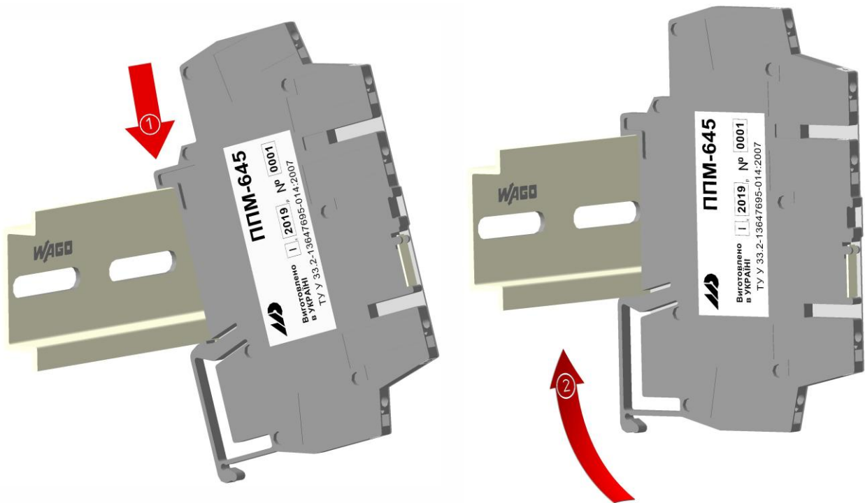
Рисунок 3.1 - Схема кріплення перетворювача ППМ-645 на DIN-рейку
