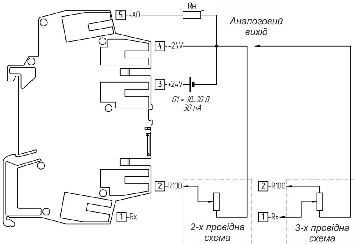
Рисунок 3.3 - Схема зовнішніх з'єднань перетворювача ППМ-645
