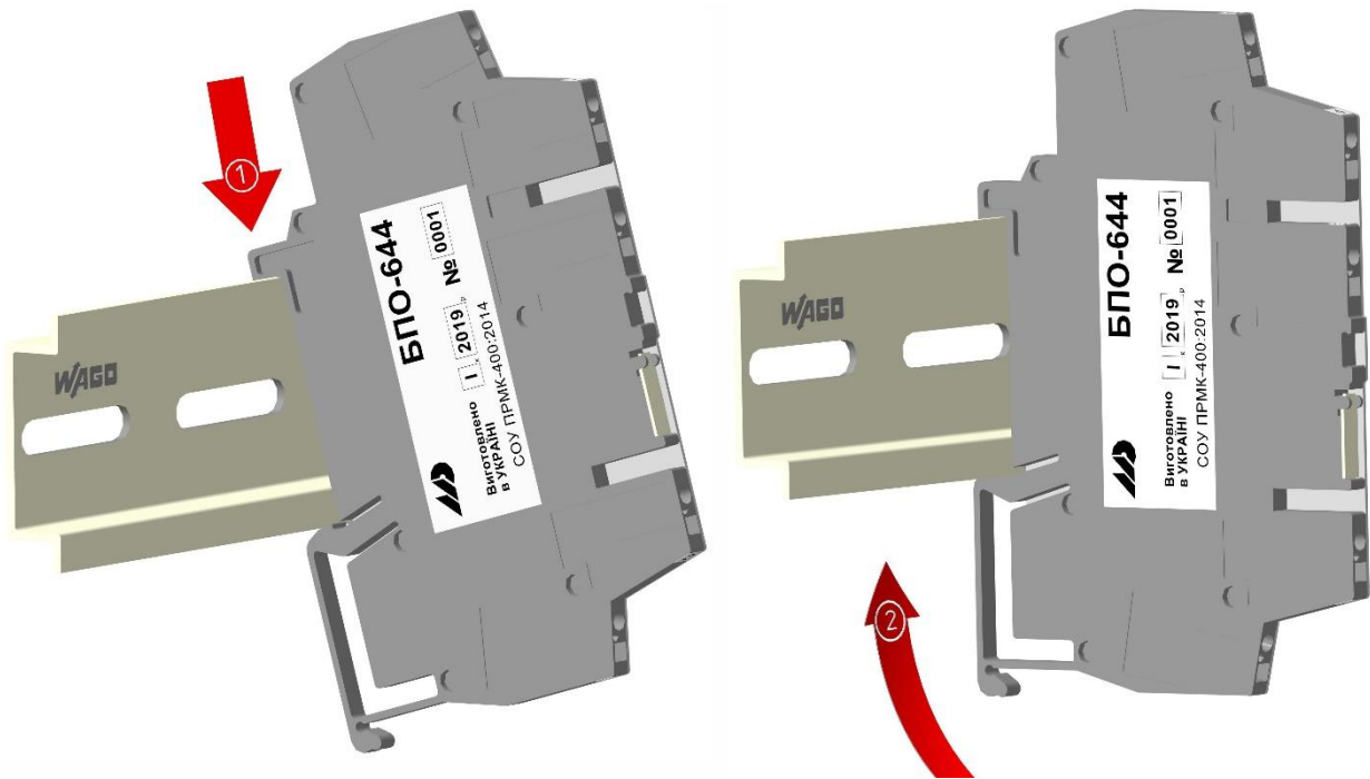
Рисунок 3.1 - Схема кріплення перетворювача БПО-644 на DIN-рейку
