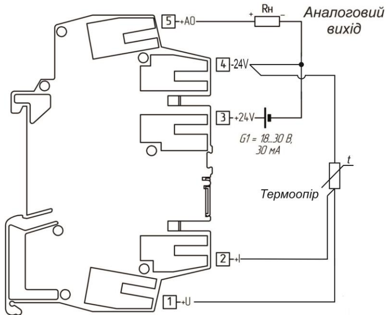
Рисунок 3.3 - Схема зовнішніх з'єднань перетворювача БПО-644
