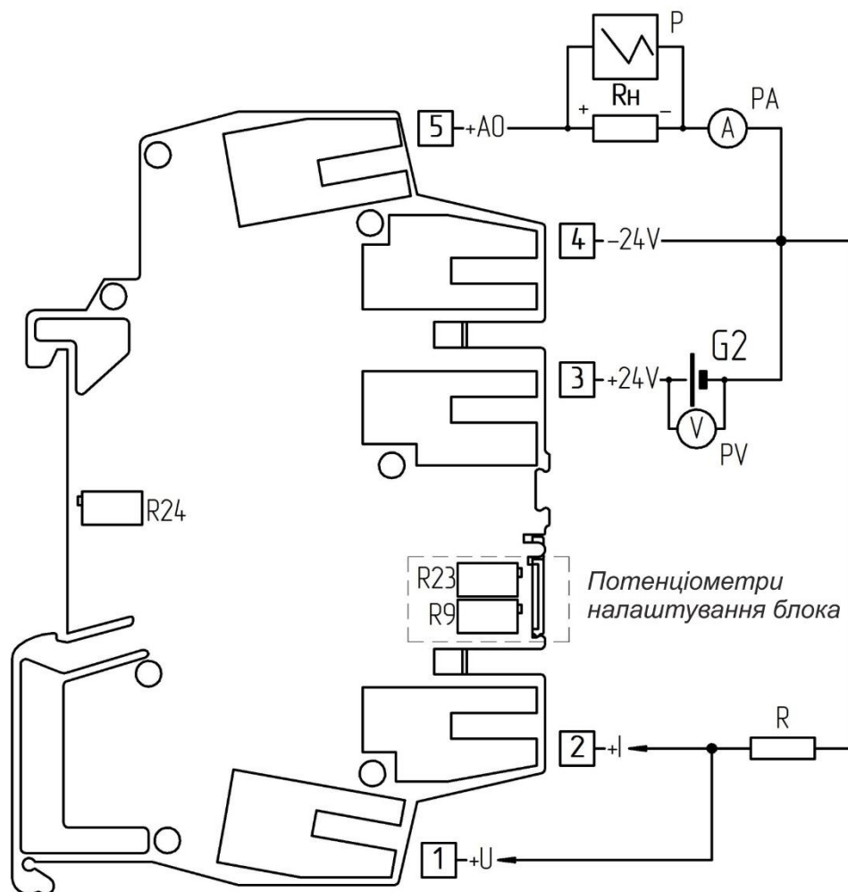
Рисунок А.1 —Схема контролю електричних параметрів перетворювача
