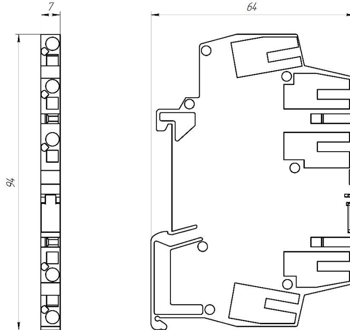
Рисунок 1.1 - Зовнішній вигляд і габаритні розміри перетворювача БПО-644
