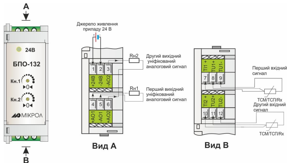
Рисунок 3.3 - Схема електрична підключень блоку БПО-132
