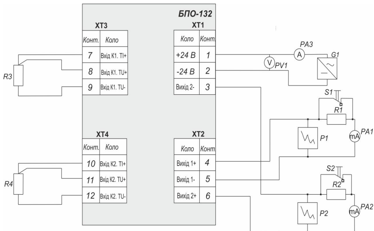
Рисунок Б.1 - Схема контролю електричних параметрів перетворювача
