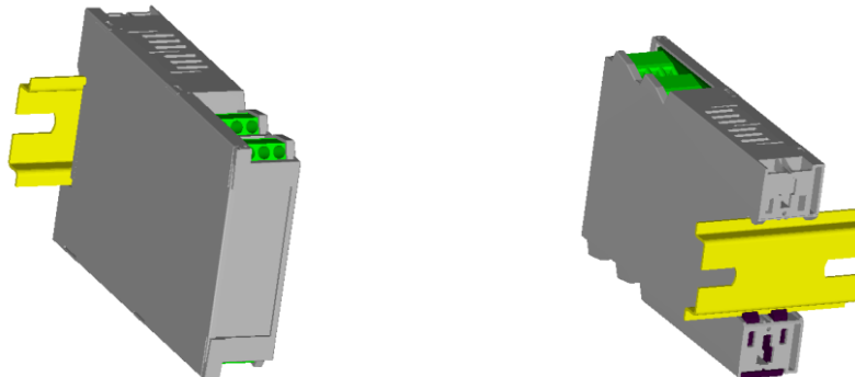
Рисунок 3.1 - Схема кріплення блоку на щит
