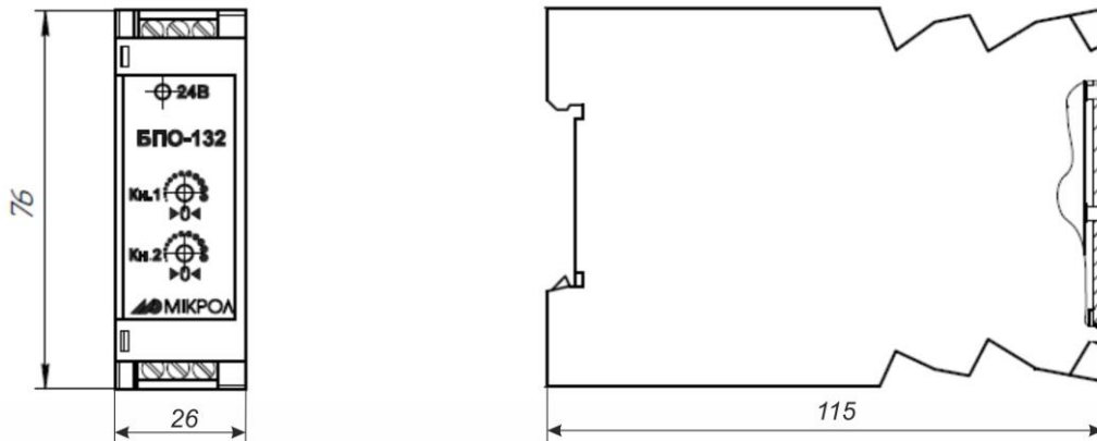
Рисунок 1.1 - Зовнішній вигляд і габаритні розміри БПО-132
