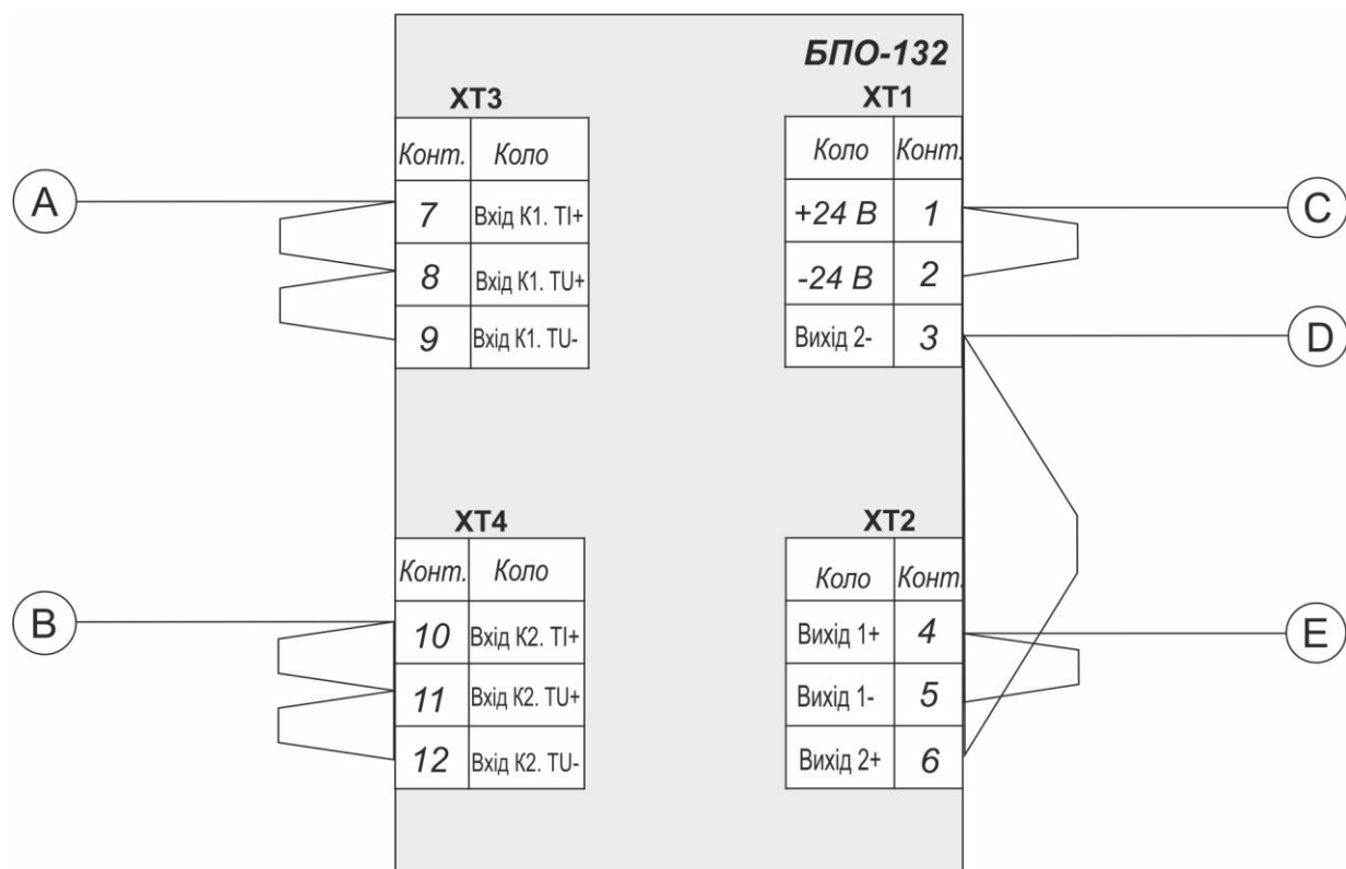
Рисунок А.1 - Схема перевірки опору ізоляції
