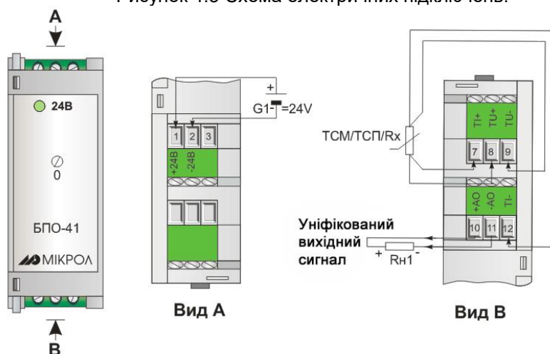
Рисунок 4.4 Схема електричних підключень.
