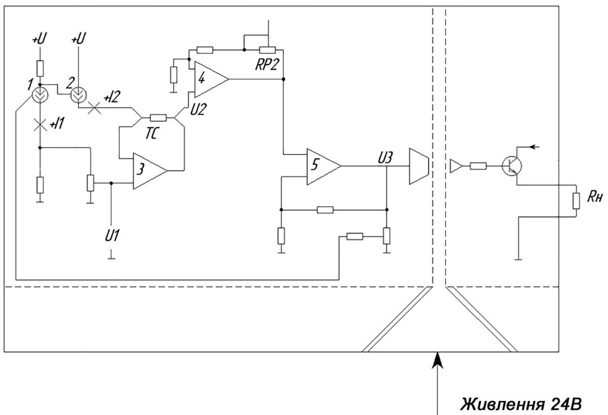
Рисунок 2.1 – Блок-схема перетворювача БПО-41
