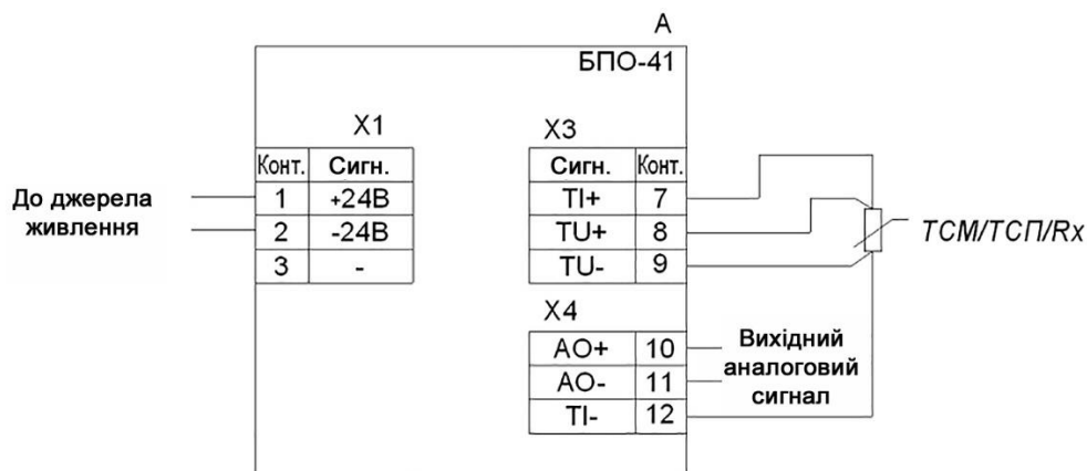
Рисунок 4.3 Схема електричних підключень.
