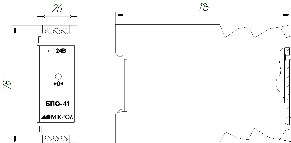
Рисунок 1.1 - Зовнішній вигляд та габаритні розміри БПО-41
