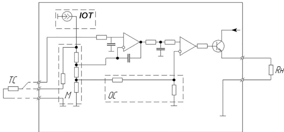
Рисунок 2.2 – Блок-схема перетворювача БПО-32
