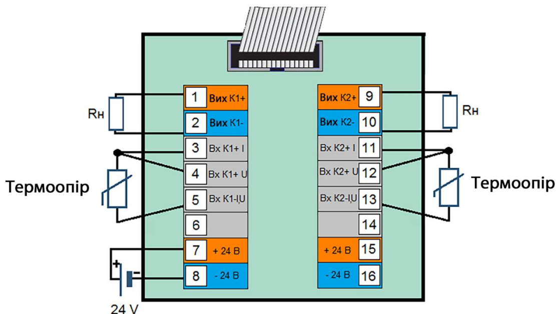
Рисунок 4.3 Схема електричних підключень до КБЗ-16-11
