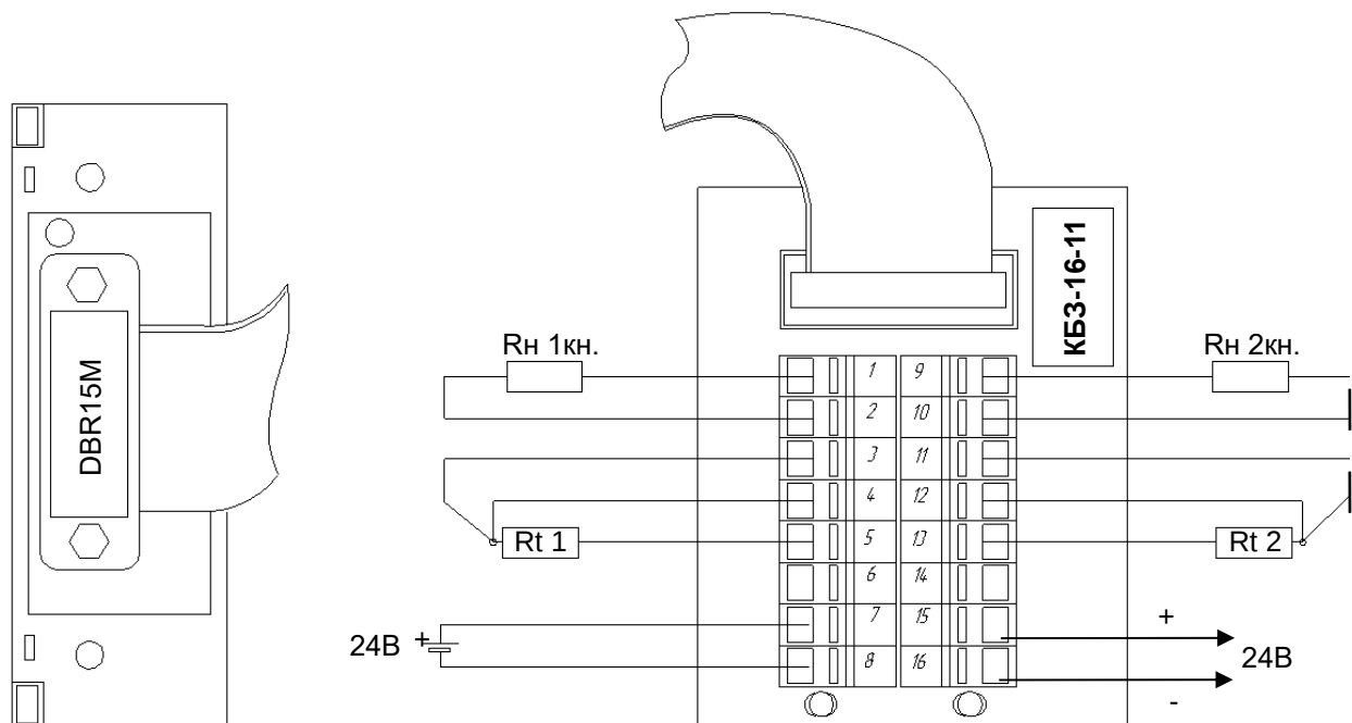
Рисунок 2.3 – Схема зовнішніх з'єднань БПО-32
