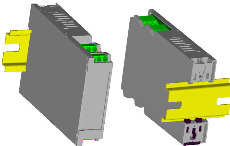
Рисунок 4.1 – Схема кріплення блоку на щит
