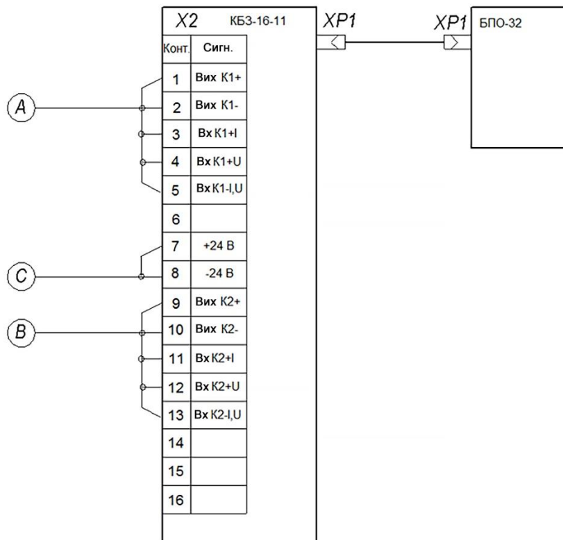
Рисунок А.1. Схема перевірки опору ізоляції
