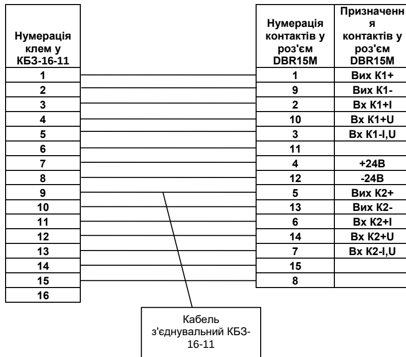
Рисунок 2.4 - Схема розпаювання кабелю клемно-блокового з'єднувача КБЗ-16-11 та зовнішні сигнали БПО-32
