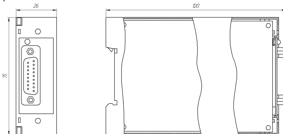
Рисунок 1.1 - Зовнішній вигляд та габаритні розміри БПО-32
