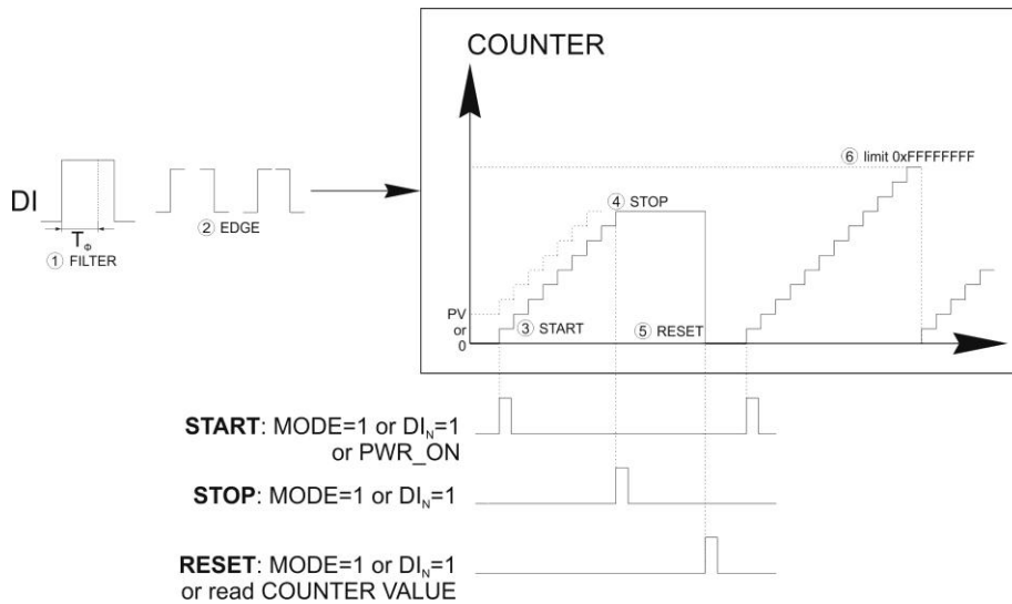
Рисунок 3.2 - Схема роботи лічильника
