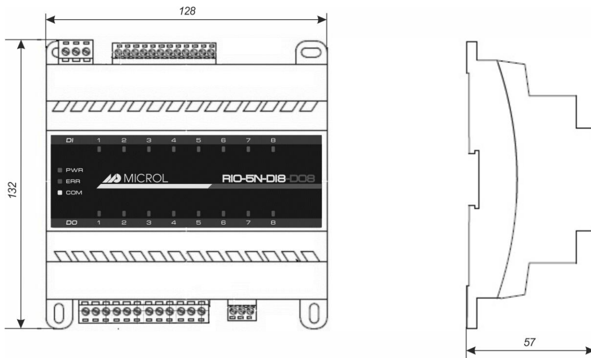
Рисунок А.1 - Габаритні розміри RIO-5N-DI8-DO8
