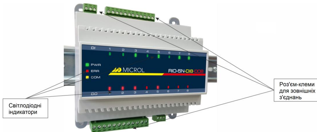
Рисунок. 3.1 - Зовнішній вигляд модуля дискретного вводу/виводу RIO-5N-DI8-DO8
