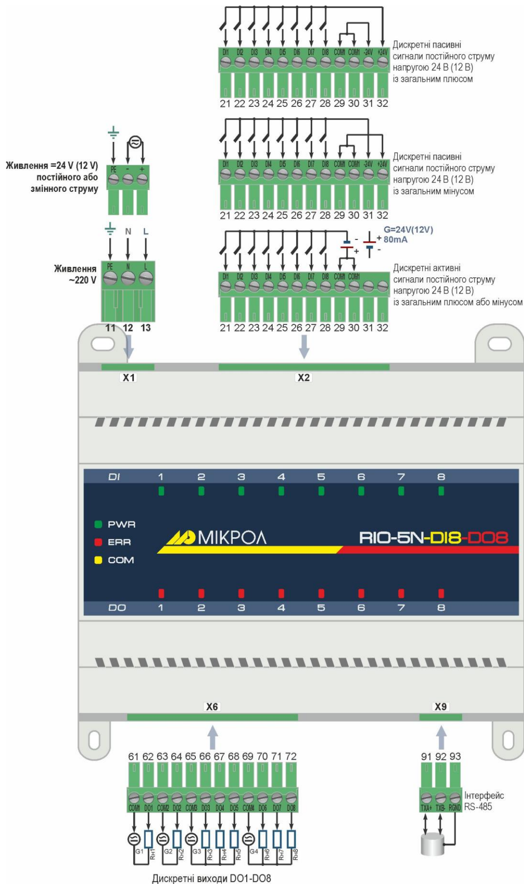
Рисунок Б.1 - Нумерація клем і зовнішні підключення модуля дискретного вводу/виводу RIO-5N-DI8-DO8
