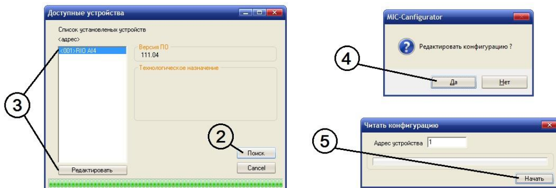
Рисунок 4.6 - Пошук доступних пристроїв і зчитування параметрів модуля
