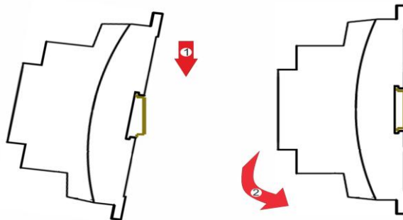
Рисунок 4.1 - Схема кріплення модуля на DIN-рейку
