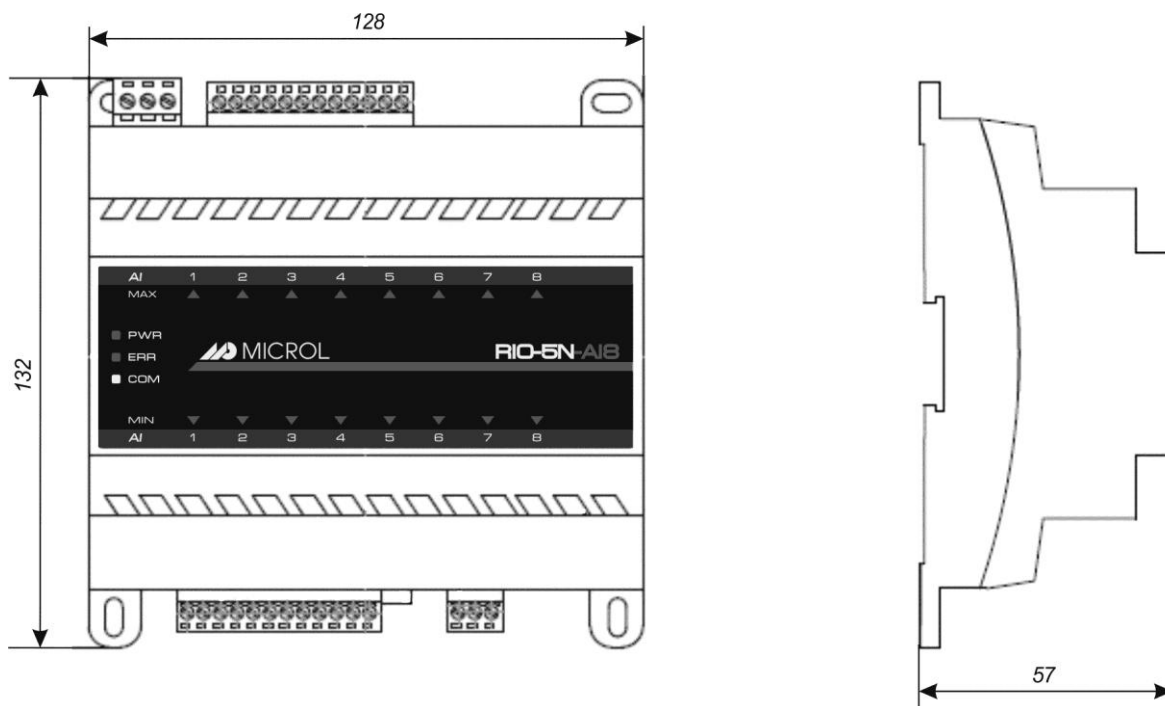
Рисунок А.1 - Габаритні розміри модуля RIO-5N-AI8
