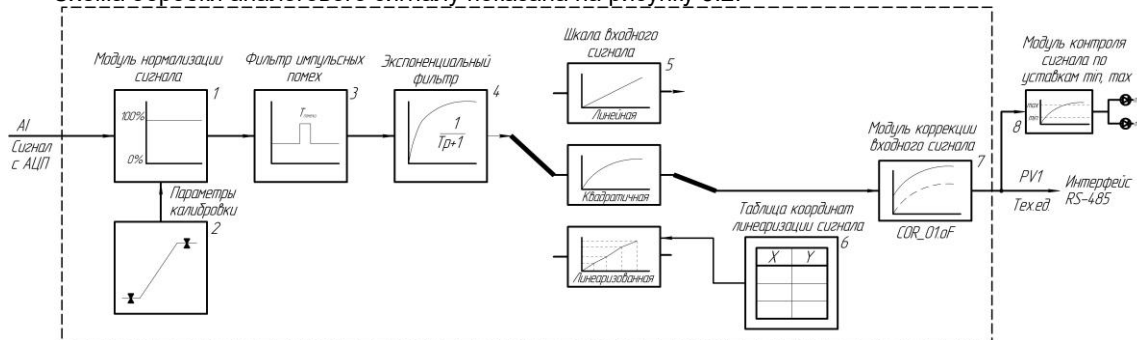
Рисунок 3.2 - Блок-схема обробки аналогового входу
