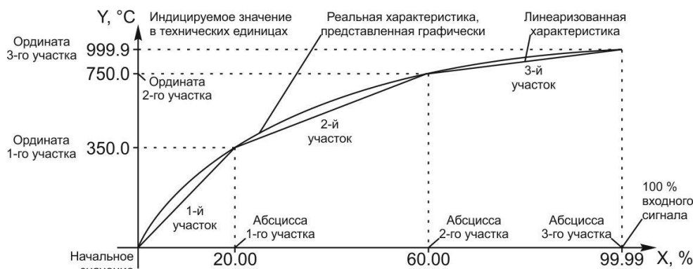
Рисунок 3.3 - Графік лінеаризованого сигналу
