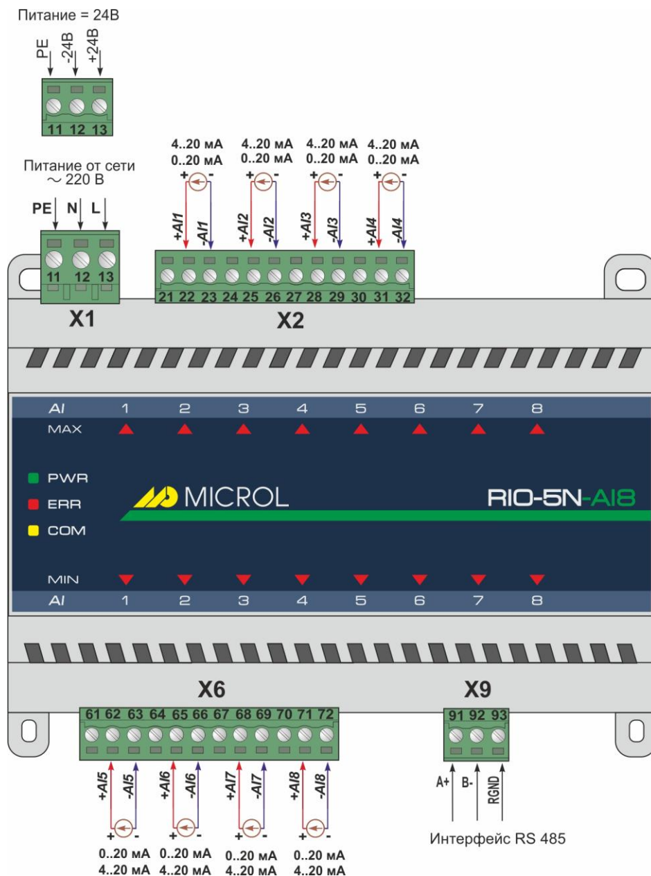
Рисунок Б.1 - Схема зовнішніх з'єднань для підключення давачів з вихідним уніфікованим сигналом постійного струму
