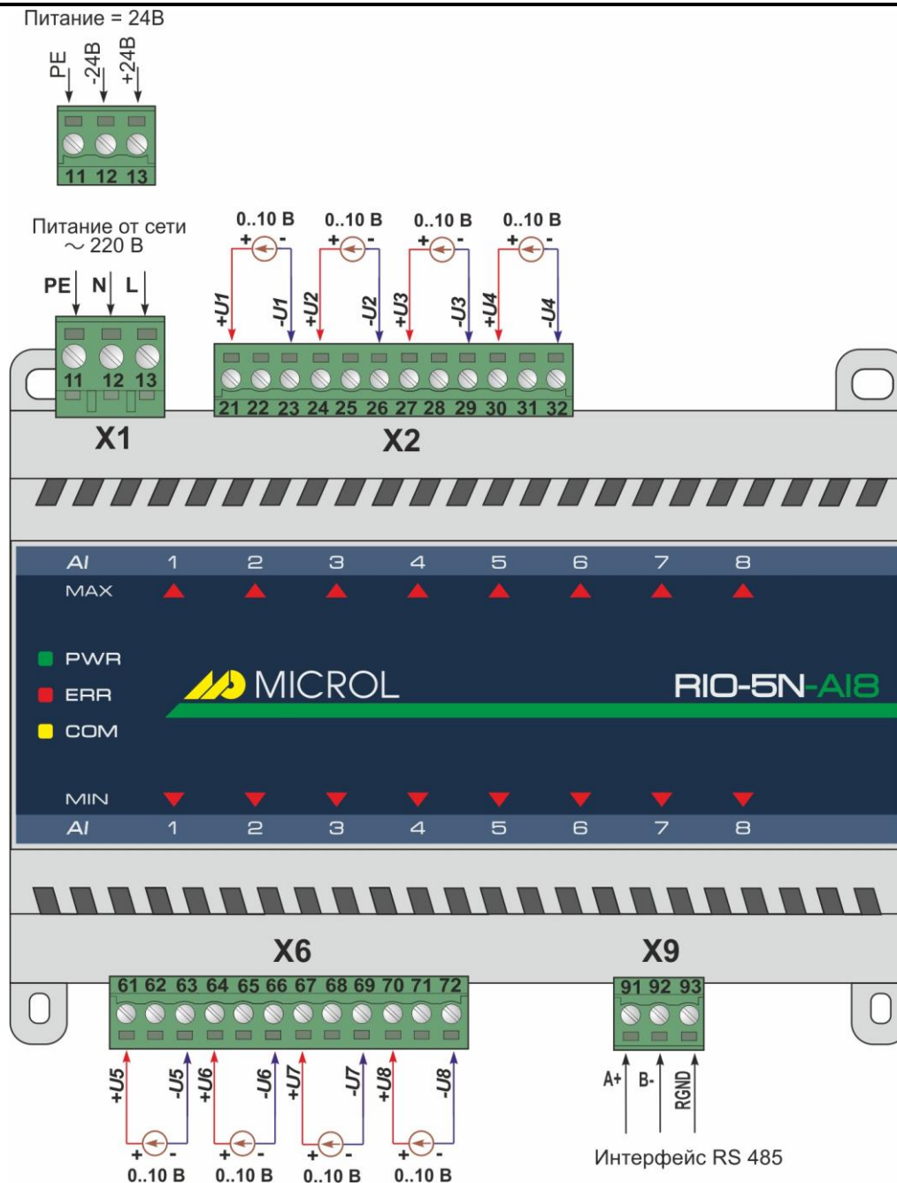
Рисунок Б.2 - Схема зовнішніх з'єднань для підключення датчиків з вихідним уніфікованим сигналом постійної напруги
