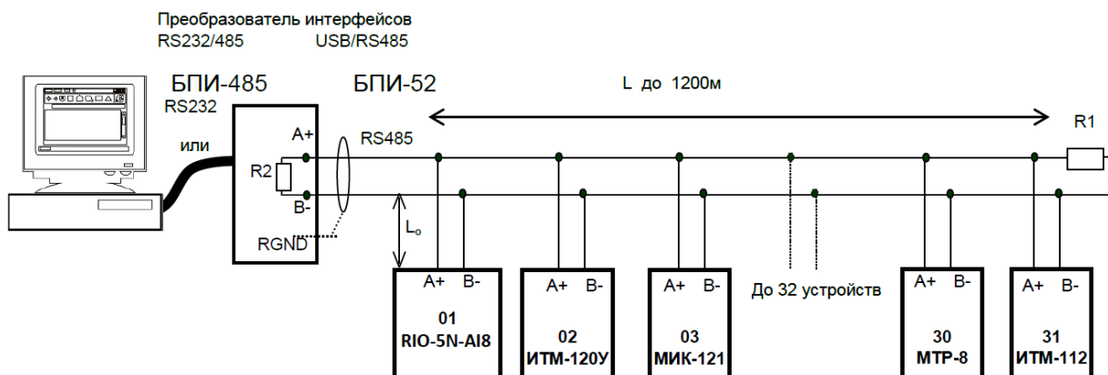
Рисунок Б.3 - Организация интерфейсного зв'язку між ПК і пристроями
