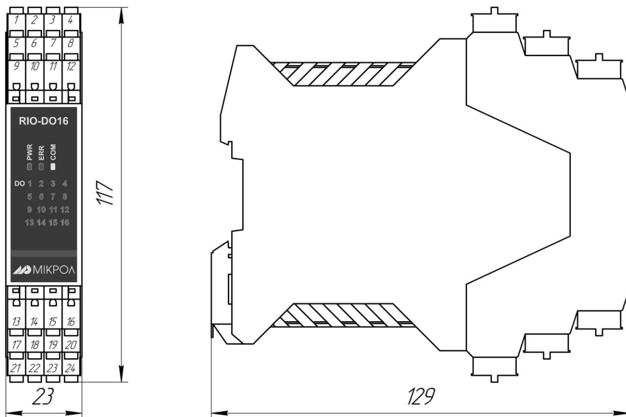
Рисунок А.1 - Габаритні розміри RIO-DO16
