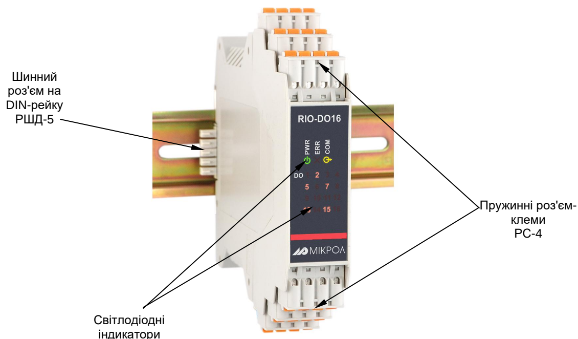
Рисунок 3.1 – Зовнішній вигляд модуля дискретного виходу RIO-DO16
