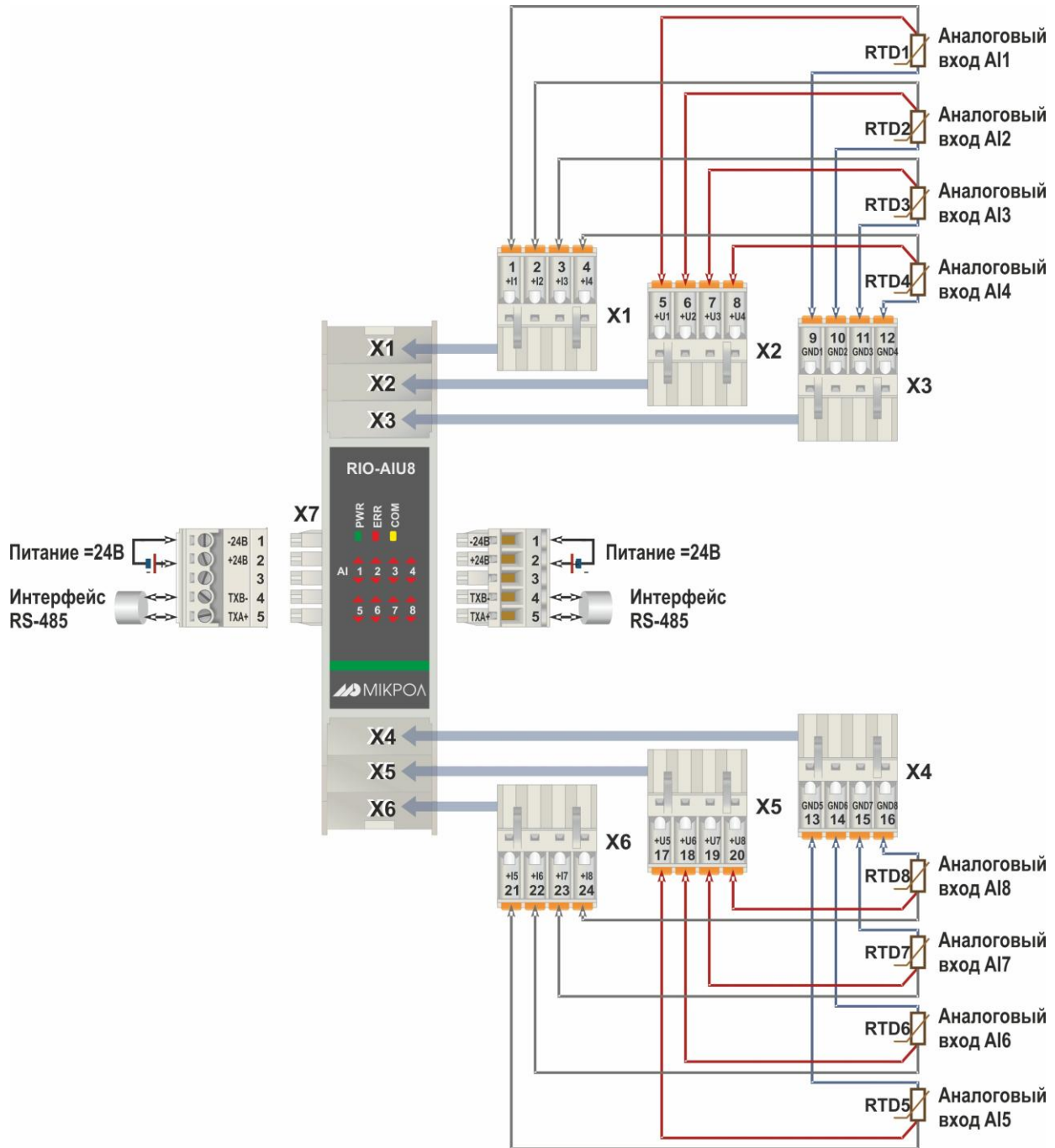
Рисунок Б.1 – Схема зовнішніх з'єднань для підключення датчиків термоопору до RIO-AIU8
