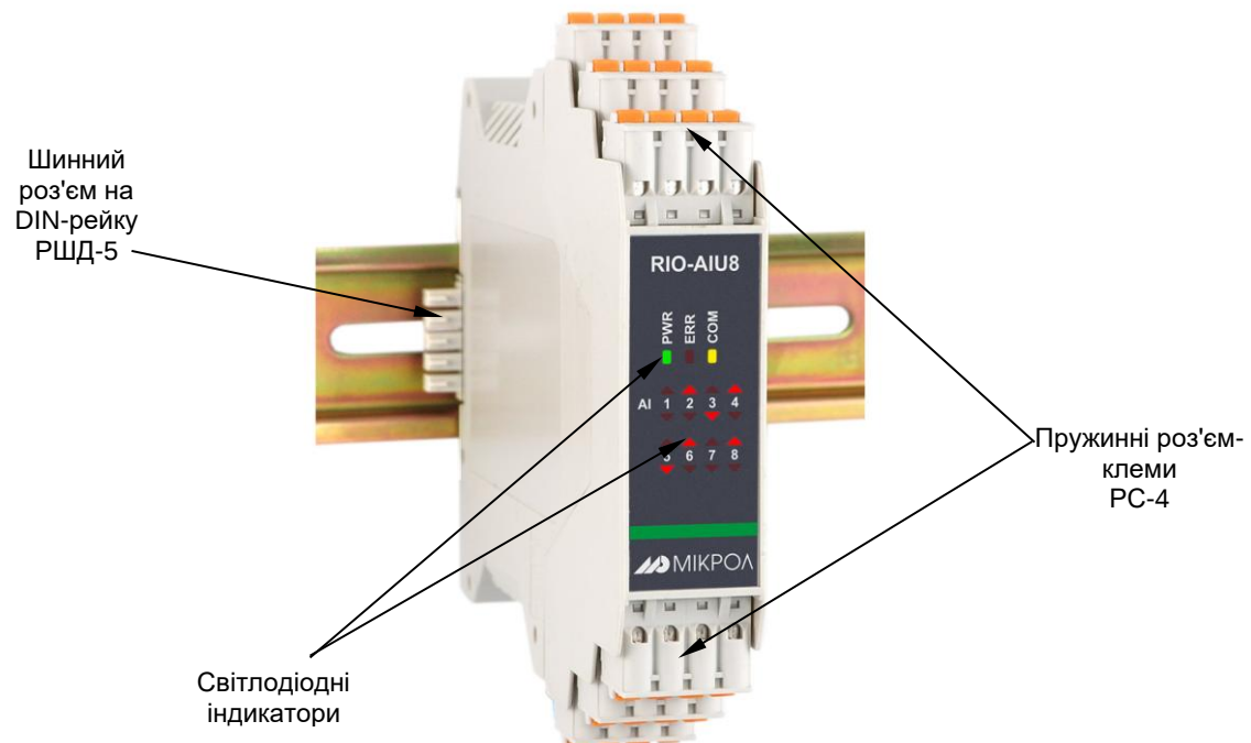
Рисунок. 3.1 - Зовнішній вигляд аналогового модуля RIO-AIU8
