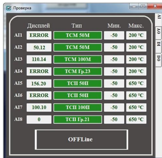
Рисунок 4.6 – Перевірка модуля
