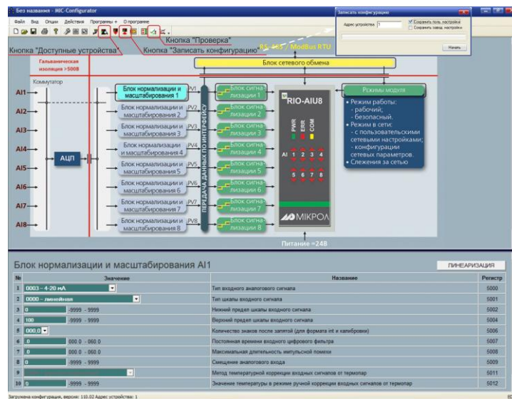
Рисунок 4.5 – Редагування конфігурації
