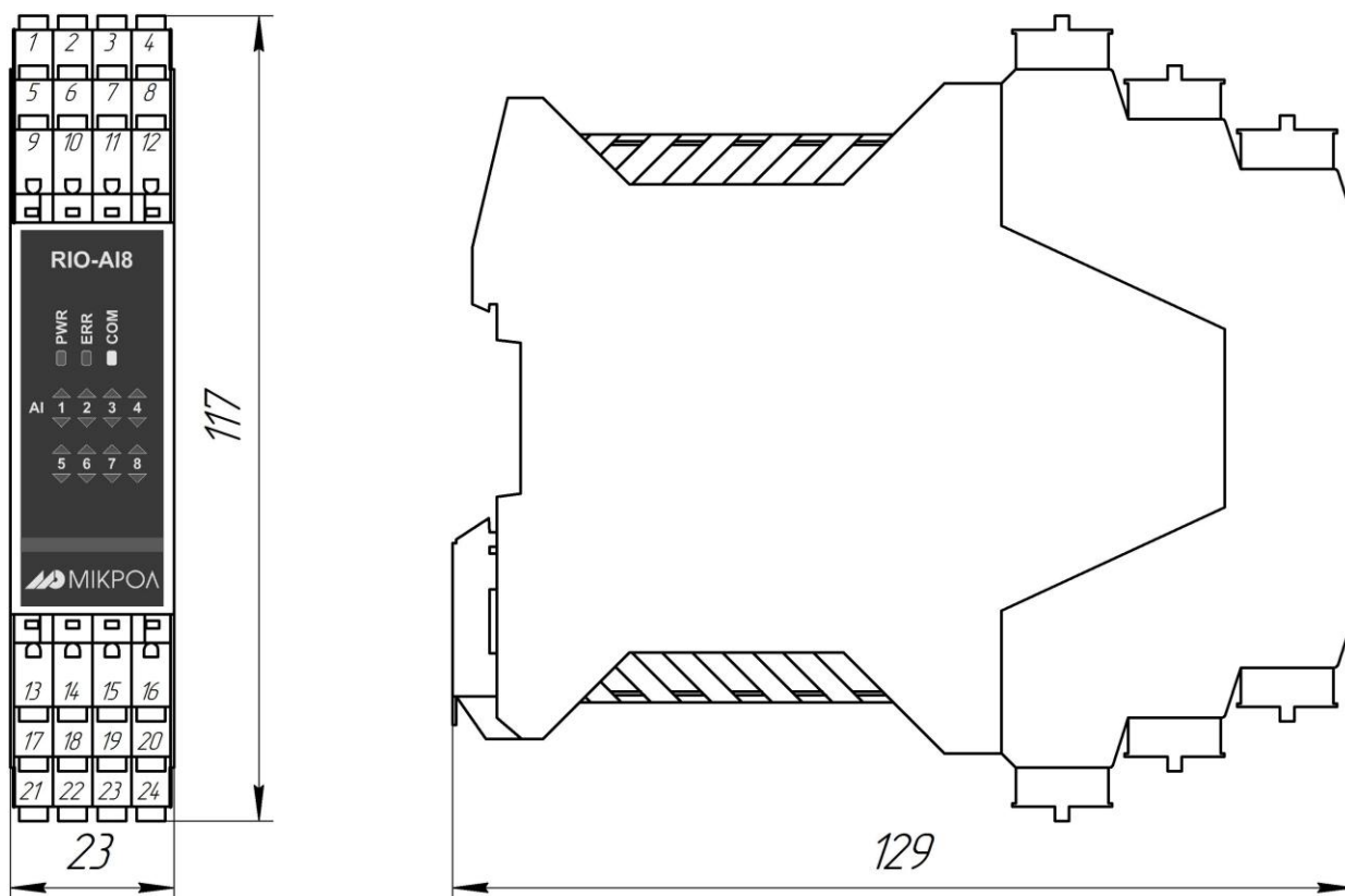
Рисунок А.1 – Габаритні розміри модуля RIO-AIU8
