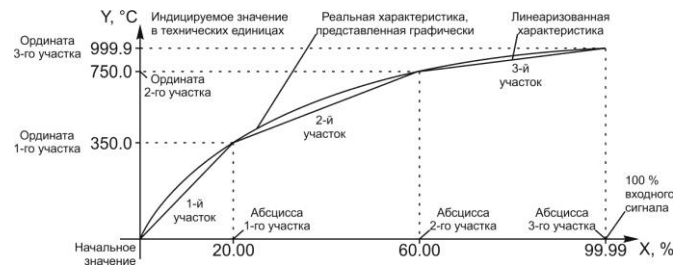
Рисунок 3.2 – Графік лінеаризованого сигналу
