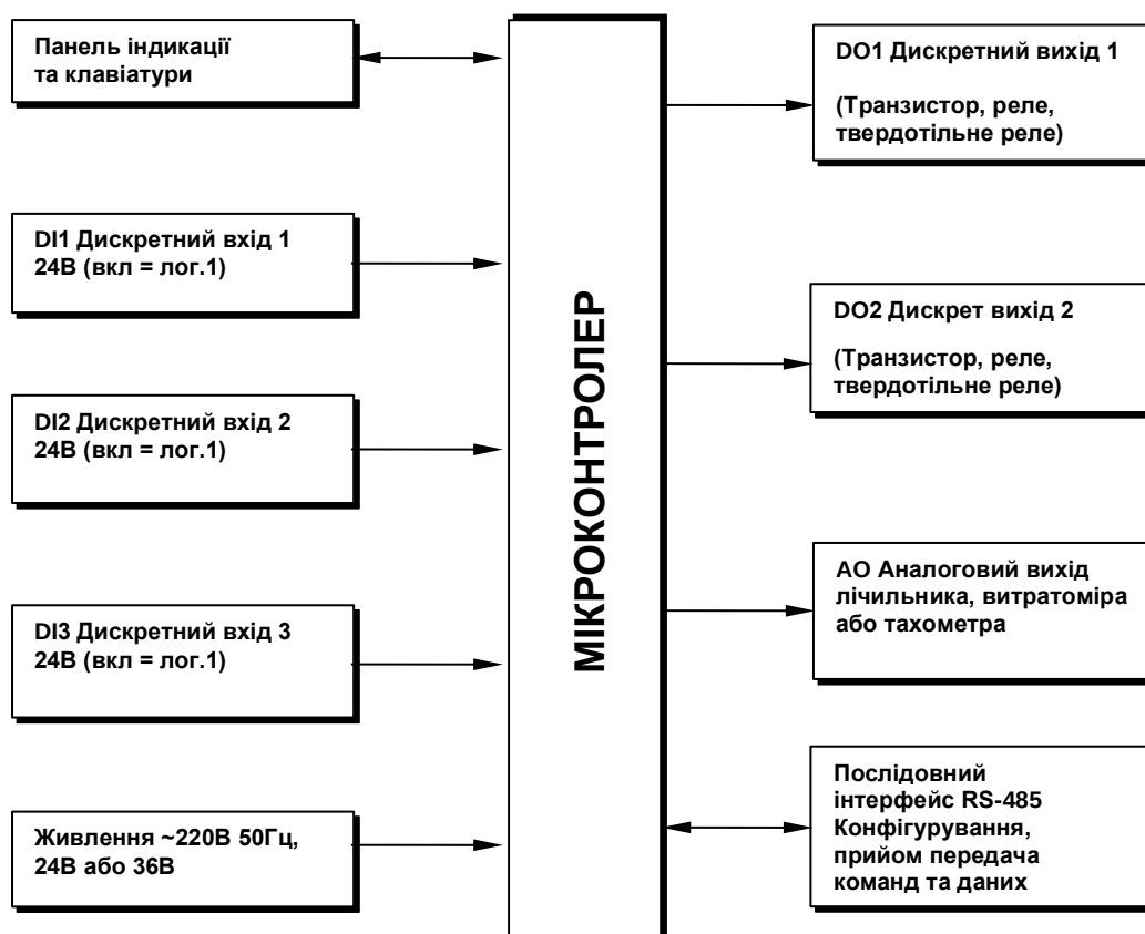
Рисунок 3.2 – Структурна схема лiчильника МТЛ-32Н
