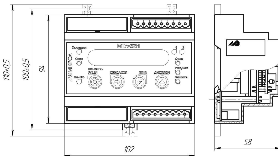
Рисунок А.2 - Габаритні розміри
