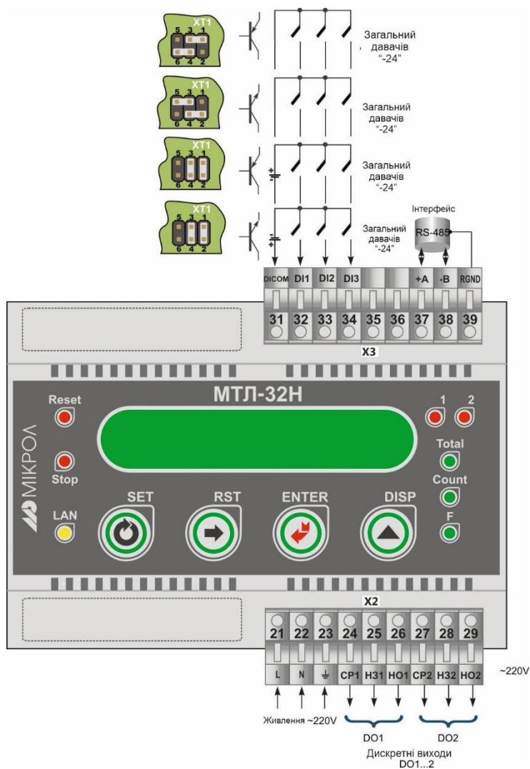
Рисунок Б.1.1 - Підключення зовнішніх ланцюгів лічильника МТЛ-32Н. Виконання на напругу 220 В змінного струму
