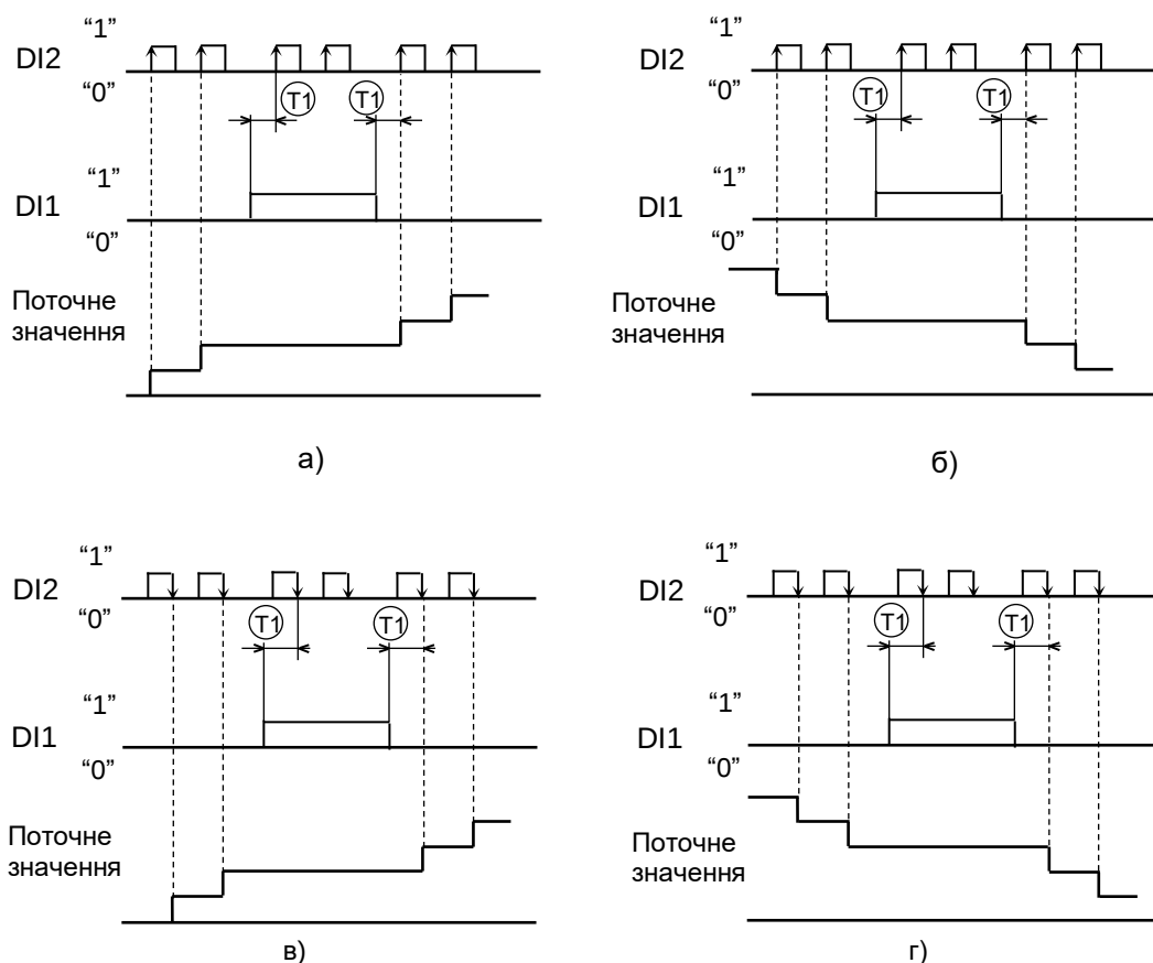
Рисунок 5.1 – Діаграми роботи лічильника МТЛ-32Н у сумарному та віднімаючому режимах рахунку
