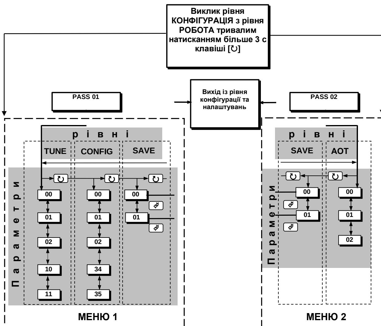
Рисунок 4.2 – Діаграма рівнів конфігурації та налаштувань.
