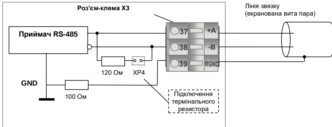
Рисунок Б.3 - Рекомендована схема підключення інтерфейсу RS-485
