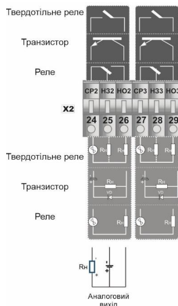
Рисунок Б.4 – Підключення аналогового виходу та дискретних навантажень до лічильника МТЛ-32Н
