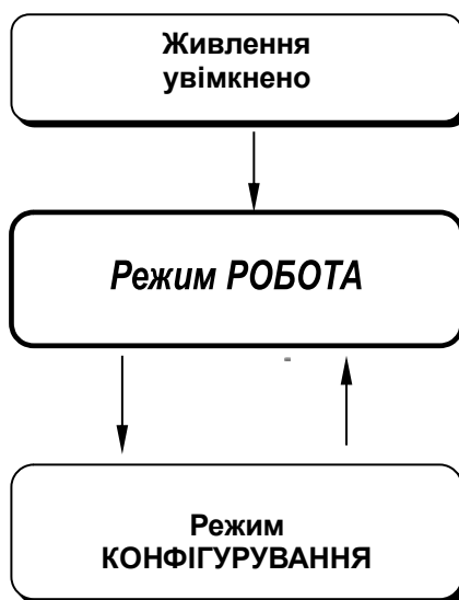
Рисунок 4.1 - Діаграма рівнів роботи, захисту та налаштувань лічильника МТЛ-32Н
