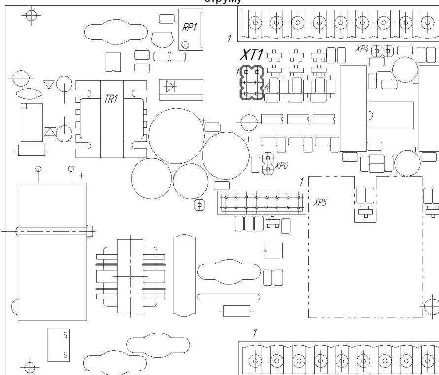
Рисунок Б.1.4 -Розташування перемичок XT1 для налаштування дискретних входів
