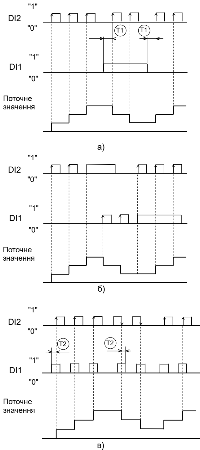
Рисунок 5.2 – Діаграми роботи лічильника МТЛ-32Н у реверсивних режимах рахунку
