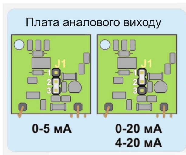
Рисунок Б.1.2 - Розташування перемичок для налаштування аналогового виходу
