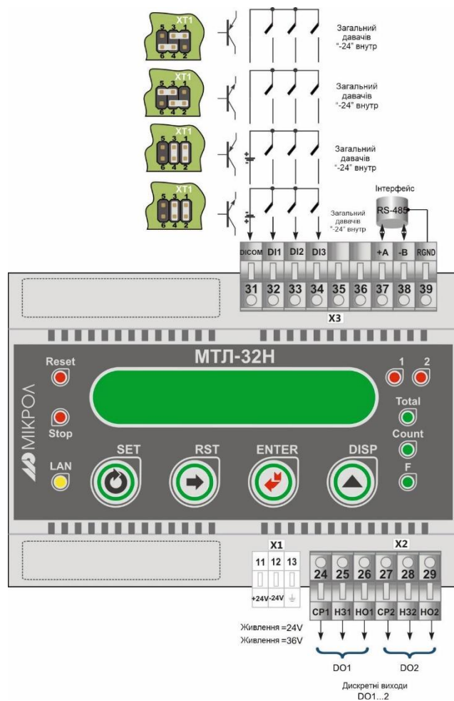
Рисунок Б.1.3 - Підключення зовнішніх ланцюгів лічильника МТЛ-32Н. Виконання на напругу 24 В постійного струму
