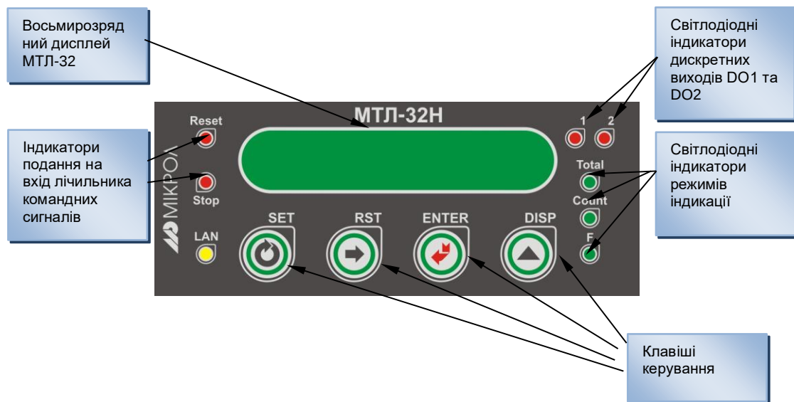
Рисунок 3.1 – Зовнішній вигляд передньої панелі лічильника МТЛ-32Н
