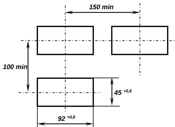
Рисунок А.2 – Розмітка отворів на щиті для встановлення тахометра
