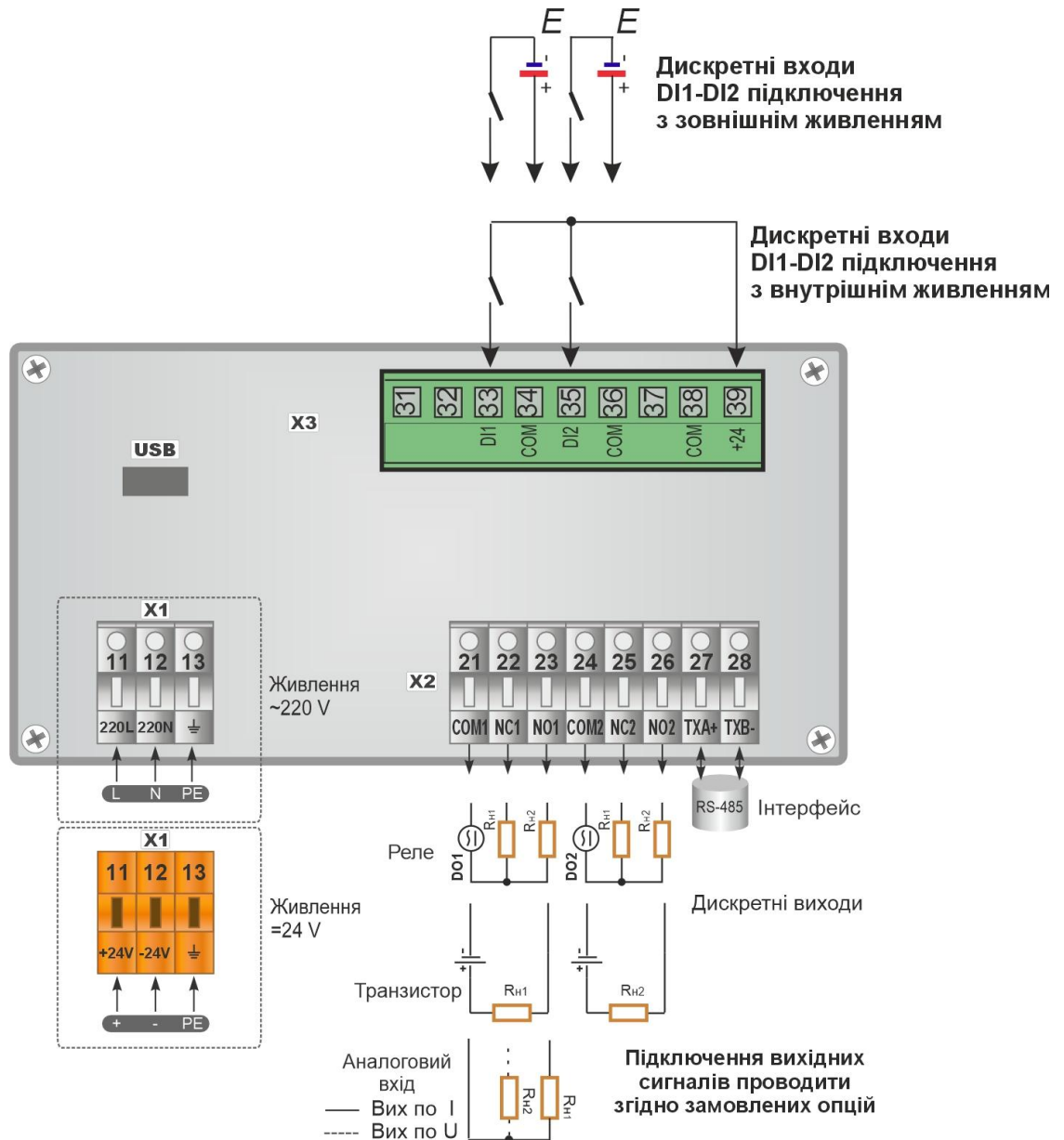
Рисунок Б.1 - Підключення зовнішніх ланцюгів тахометра ТНМ-11. Виконання на напругу 220 В змінного струму і на напругу 24 В постійного струму
