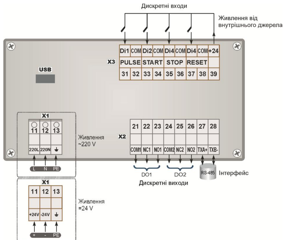
Рисунок Б.1.2 – Підключення зовнішніх ланцюгів лічильника CNT-11. Комутація вхідних сигналів від внутрішнього джерела живлення.
