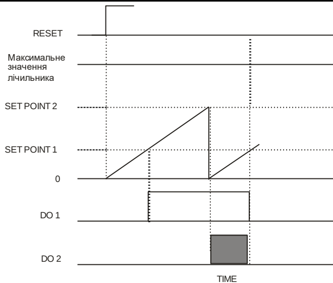
Рисунок 4.5 – Режим роботи лічильника D
