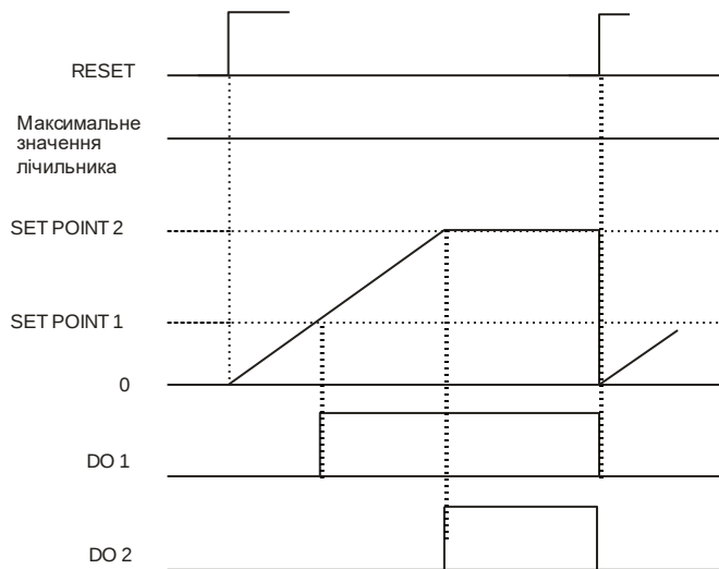
Рисунок 4.2 – Режим роботи лічильника В
