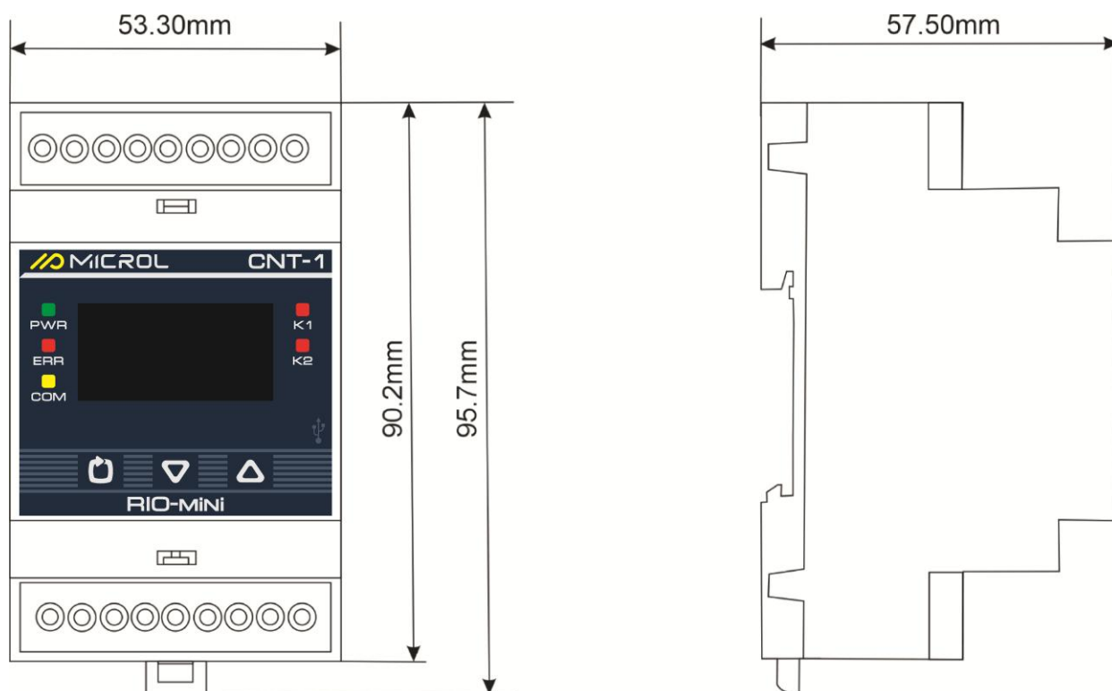
Рисунок А.1 - Габаритні розміри
