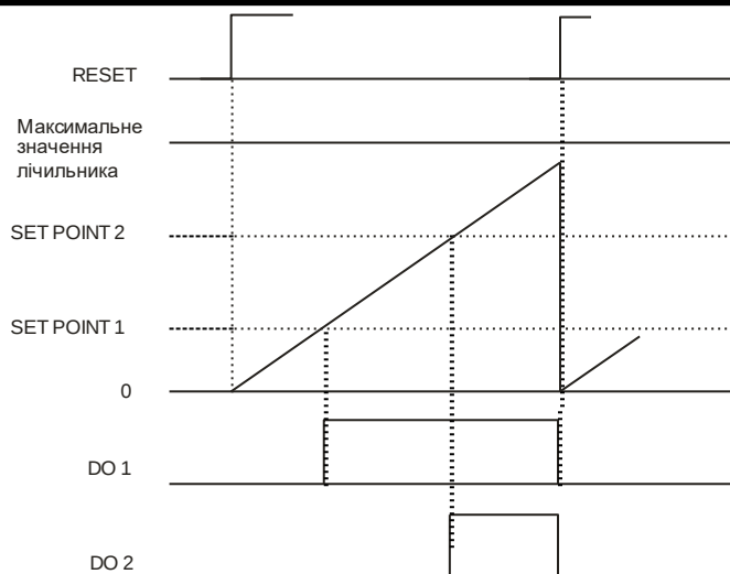
Рисунок 4.3 – Режим роботи лічильника C
