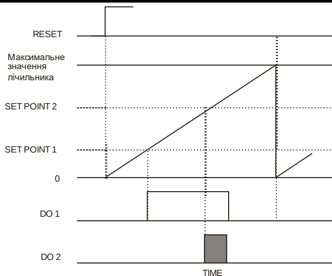
Рисунок 4.7 – Режим роботи лічильника F
