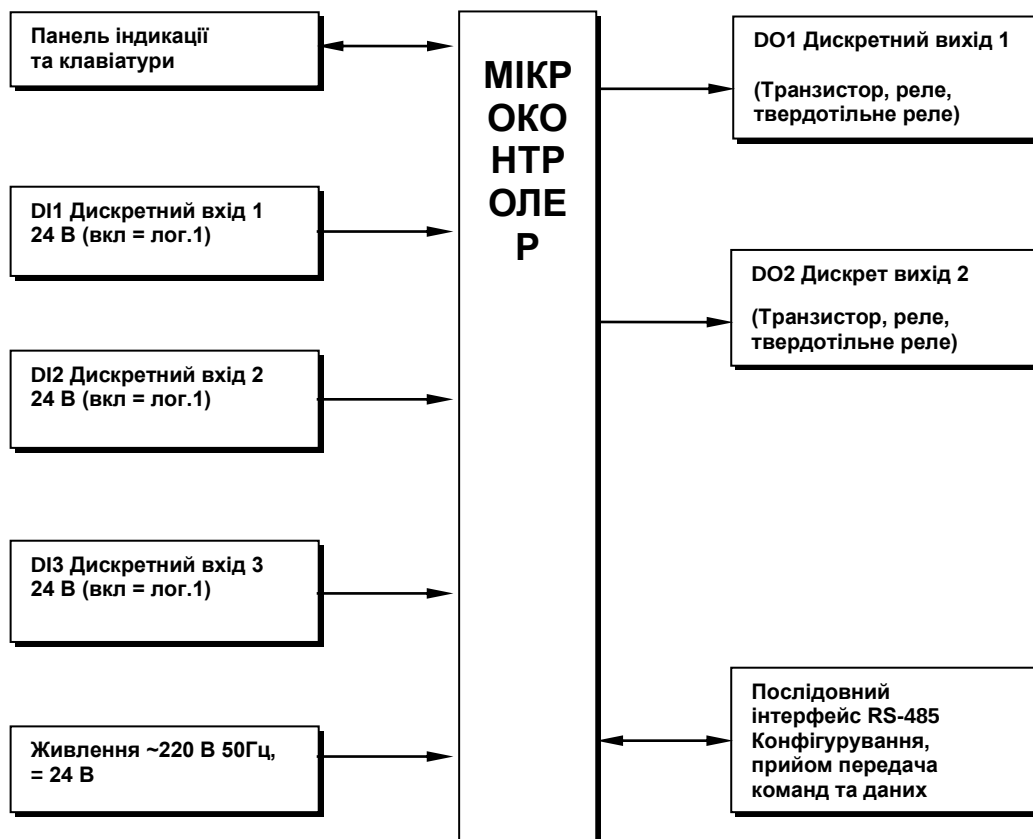
Рисунок 3.3 – Структурна схема лічильника CNT-1
