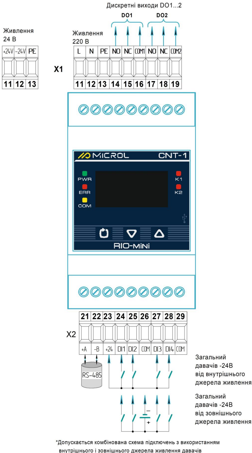
Рисунок Б.1 - Підключення зовнішніх ланцюгів лічильника CNT-1. Виконання на напругу 220 В змінного струму і на напругу 24 В постійного струму
