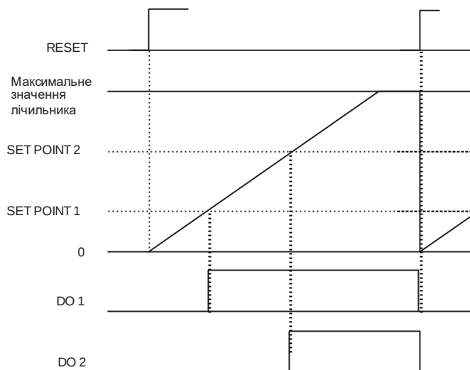
Рисунок 4.4 – Режим роботи лічильника C1
