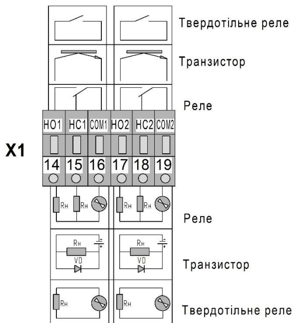
Рисунок Б.3 – Підключення аналогового виходу та дискретних навантажень до лічильника CNT1
