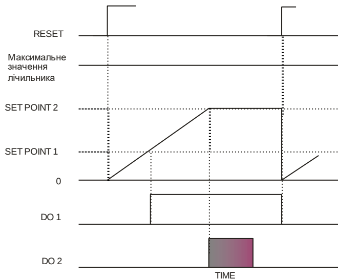
Рисунок 4.1 – Режим роботи лічильника А
