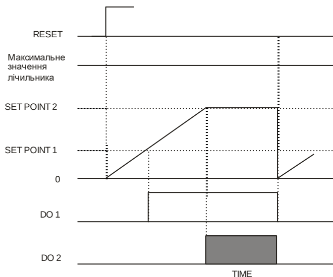
Рисунок 4.6 – Режим роботи лічильника E
