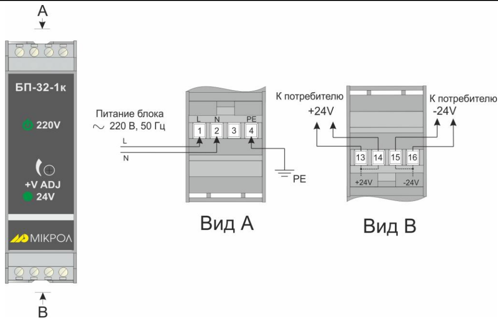
Рисунок 3.4 - Схема зовнішніх з'єднань БП-32-1к
