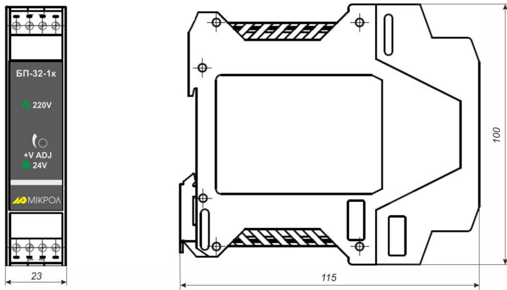
Рисунок 1.1 - Зовнішній вигляд і габаритні розміри БП-32-1к
