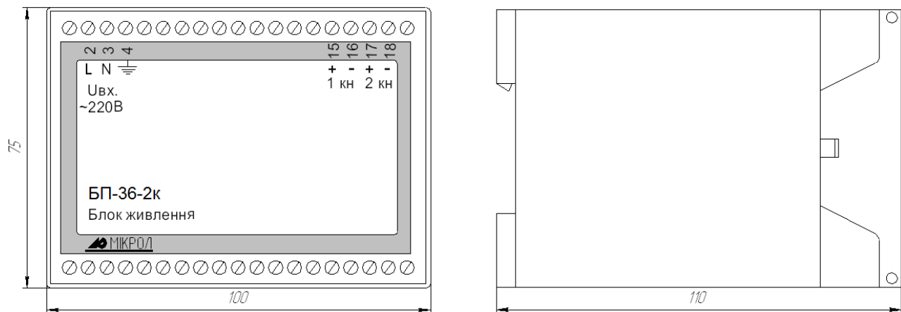
Рисунок 1.1 - Зовнішній вигляд та габаритні розміри блока живлення
