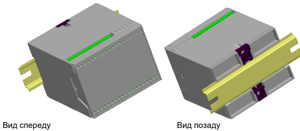
Рисунок 3.1 – Схема кріплення блока живлення на щиті
