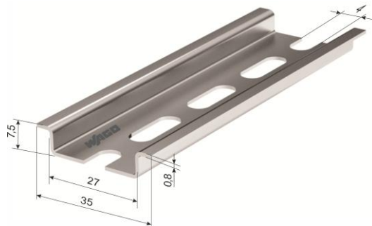
Рисунок 3.2 – Зовнішній вигляд та розміри DIN-рейки Wago
