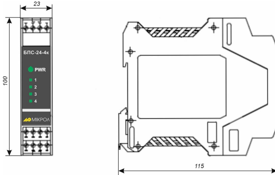
Рисунок 1.1 – Зовнішній вигляд та габаритні розміри блоку БПС-24-2К(4К)-H20
