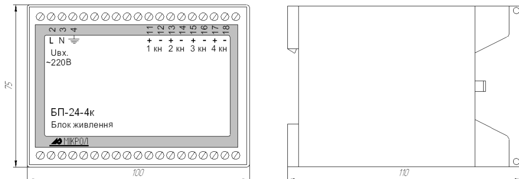
Рисунок 1.1 - Зовнішній вигляд та габаритні розміри блока живлення
