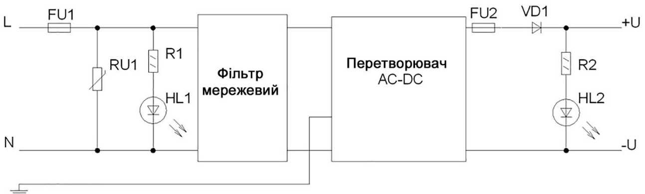
Рисунок 1.2- Схема структурного електричного блоку БП-30-2к
