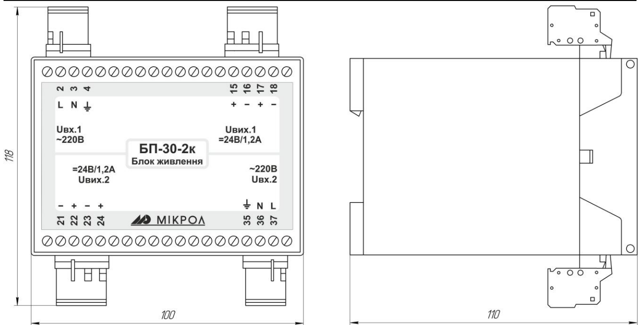
Рисунок 1.1 – Зовнішній вигляд та габаритні розміри БП-30-2к
