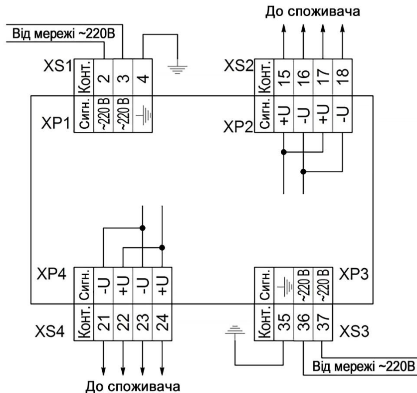
Рисунок 3.3 – Схема зовнішніх з'єднань БП-30-2к
