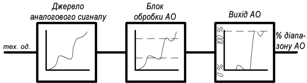
Рисунок 3.8 – Робота блоку аналогового виходу у режимі ретрансмісії
