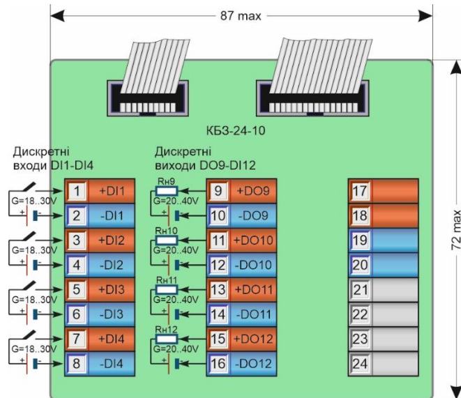
Рисунок Б.4.2 - Підключення сигналів модуля розширення MP-51-02 за допомогою клемно-блочного з'єднувача КБ3-24-10
