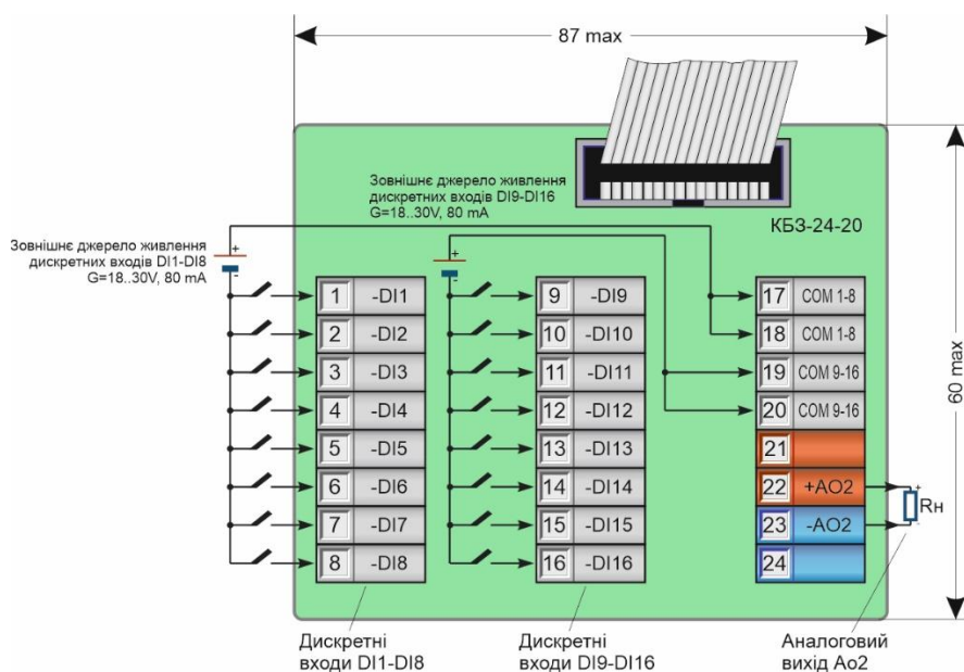
Рисунок Б.4.12 - Підключення сигналів модуля розширення MP-51-11 за допомогою клемно-блочного з'єднувача КБ3-24-20
