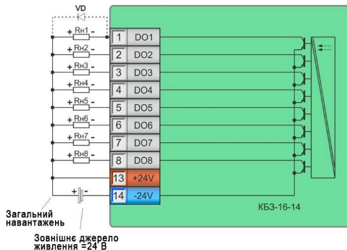
Рисунок Б.3.2 – Підключення дискретних виходів за допомогою клемно-блочного з'єднувача KB3-16-14
