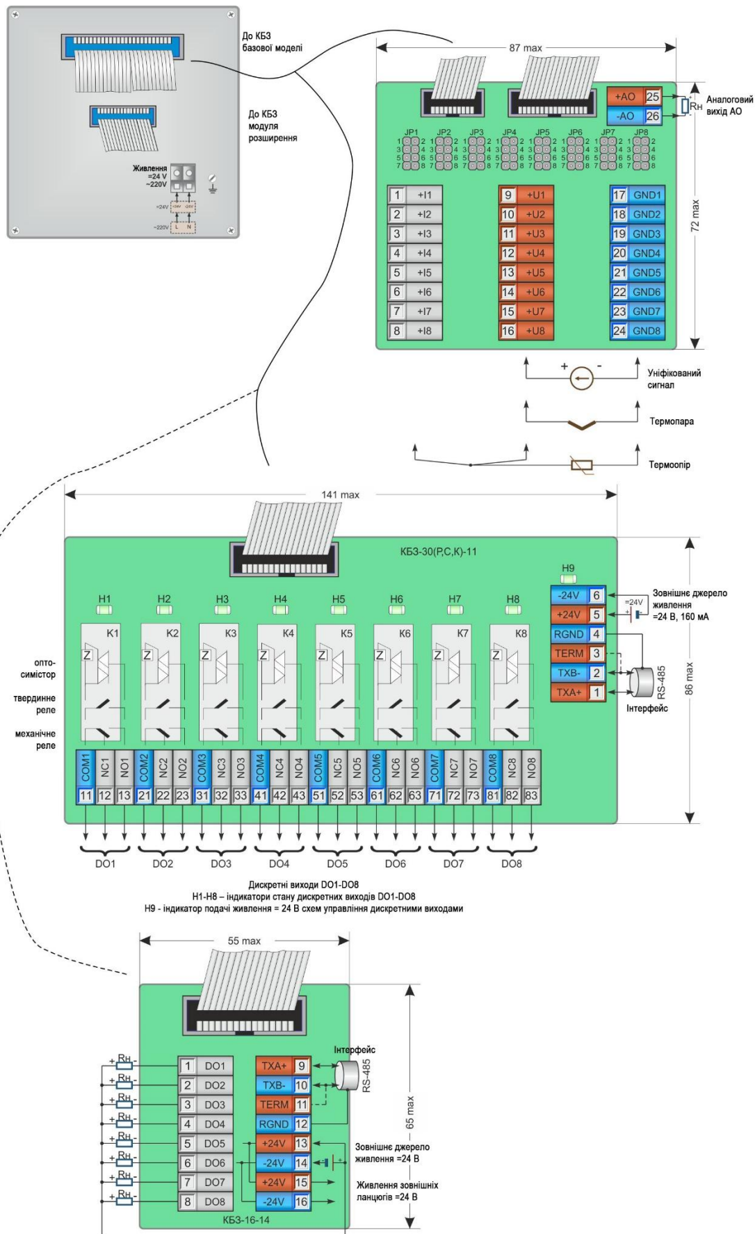
Рисунок Б.1 - Підключення клемно-блочних з'єднувачів КБЗ-24-17, КБЗ-30Р(С,К)-11, КБЗ-16-14 до регулятора
