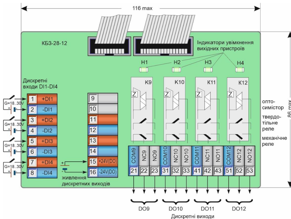
Рисунок Б.4.3 - Підключення сигналів модуля розширення MP-51-02 за допомогою клемно-блочного з'єднувача КБ3-28 (Р, С, К)-12
