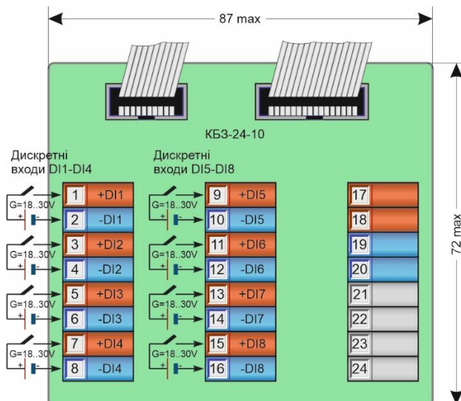
Рисунок Б.4.1 - Підключення сигналів модуля розширення MP-51-01 за допомогою клемно-блочного з'єднувача KB3-24-10
