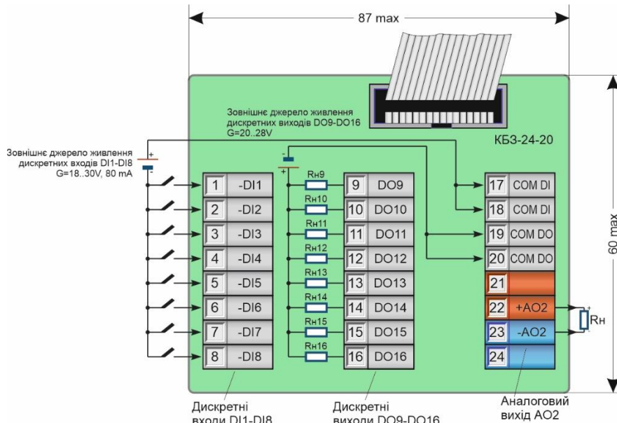
Рисунок Б.4.14 - Підключення сигналів модуля розширення MP-51-13 за допомогою клемно-блочного з'єднувача КБ3-24-20
