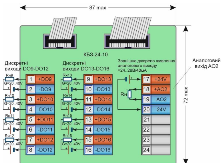
Рисунок Б.4.9 - Підключення сигналів модуля розширення МР-51-06 за допомогою клемно-блочного з'єднувача КБ3-24-10
