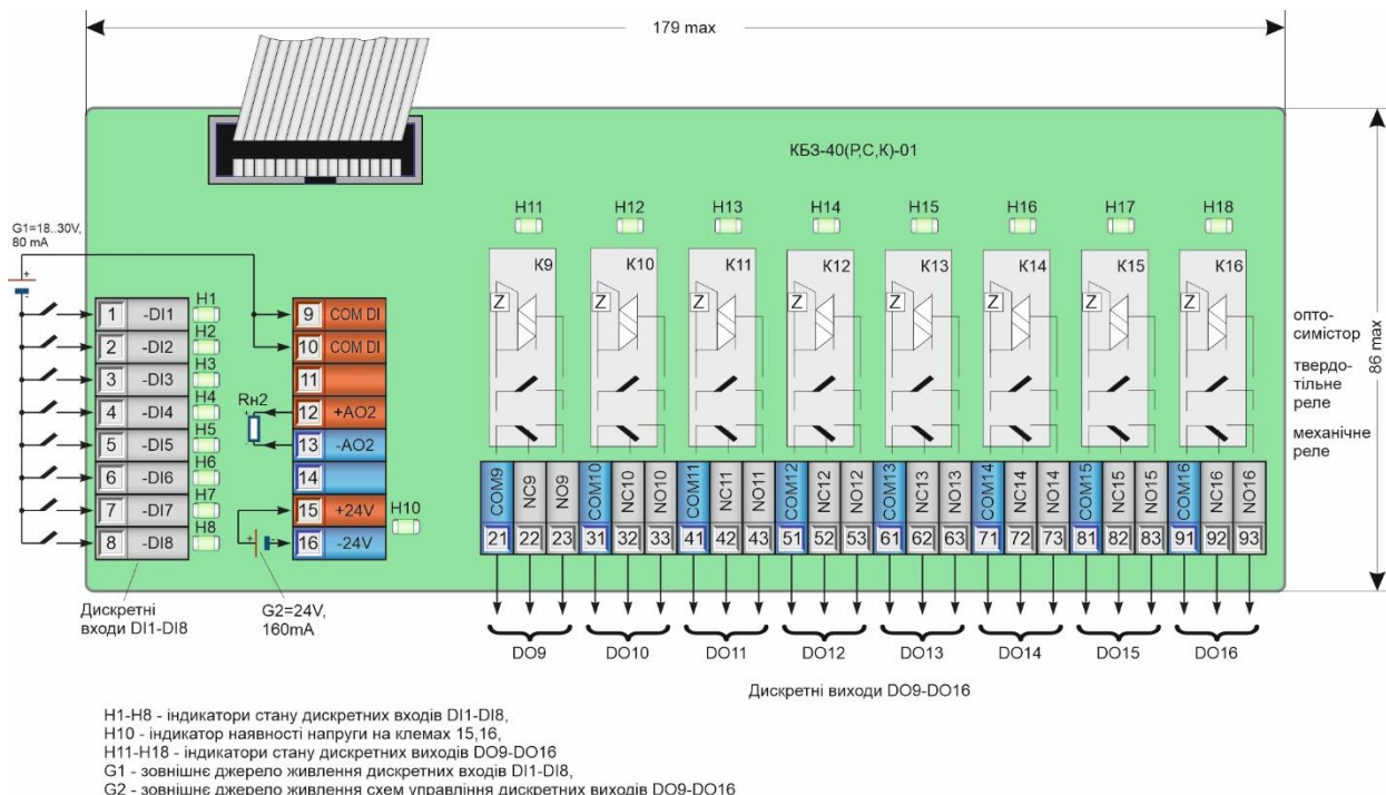
Рисунок Б.4.15 - Підключення сигналів модуля розширення MP-51-13 за допомогою клемно-блочного з'єднувача КБ3-40 (P, C, K)-01
