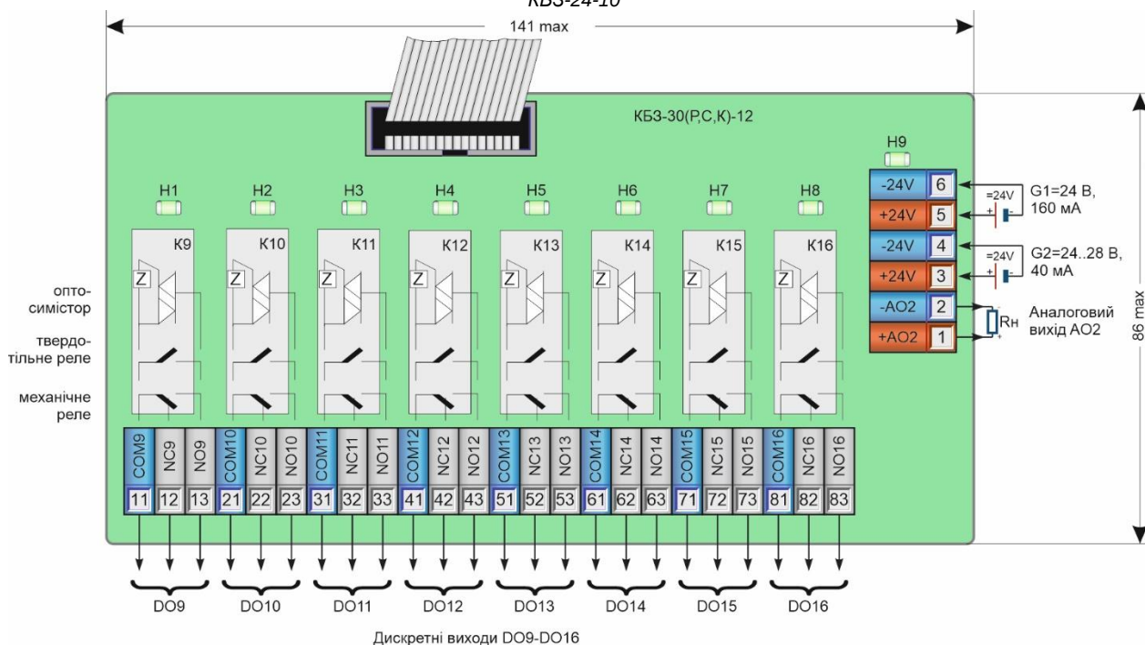
Рисунок Б.4.9 - Підключення сигналів модуля розширення МР-51-06 за допомогою клемно-блочного з'єднувача КБ3-24-10
