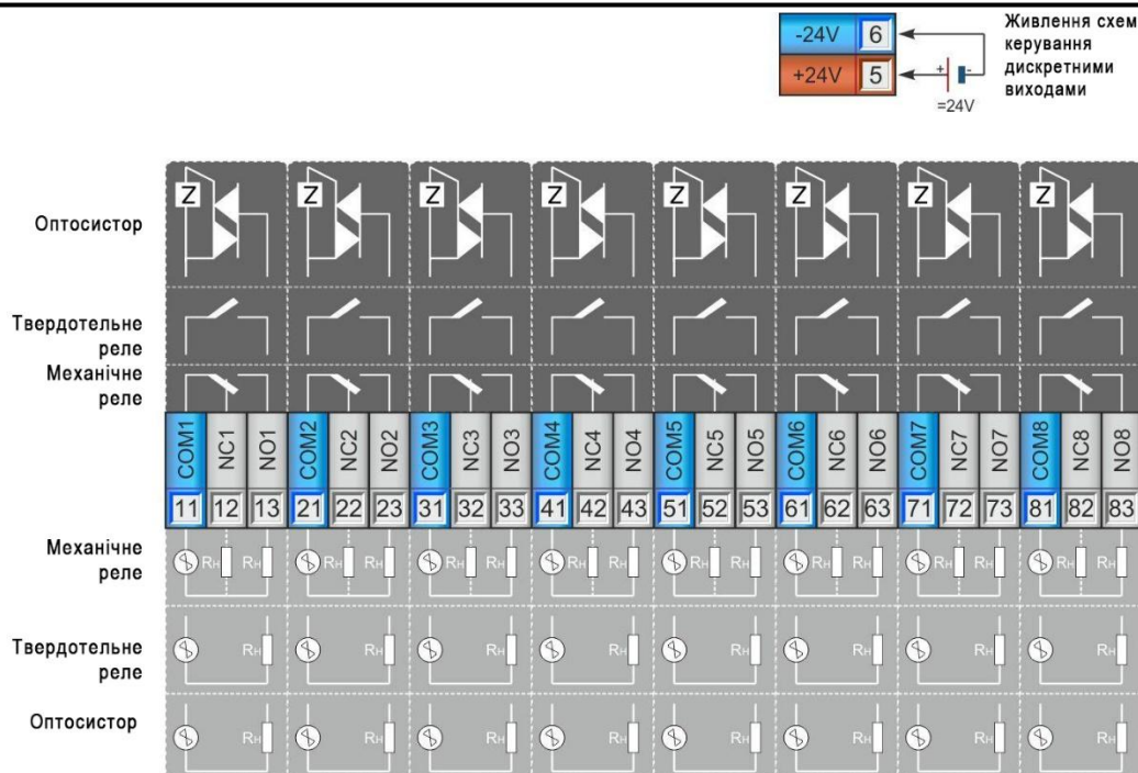
Рисунок Б.3.1 – Підключення дискретних виходів за допомогою клемно-блочного з'єднувача KB3-30P(C,K)-11
