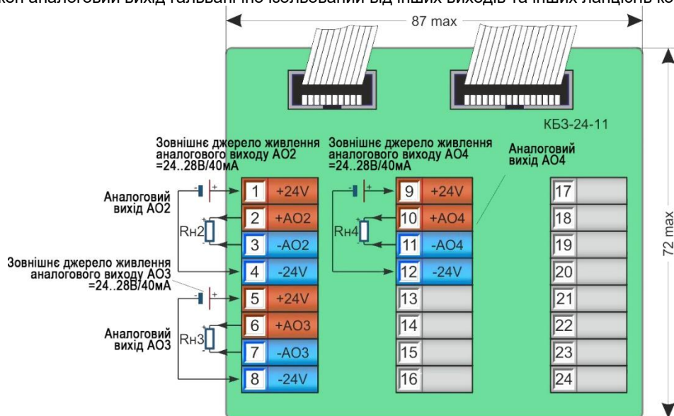
Рисунок Б.4.11 - Підключення сигналів модуля розширення MP-51-07 за допомогою клемно-блочного з'єднувача КБ3-24-11
