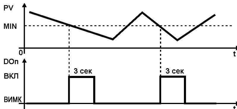
Рисунок 3.11 – Графік роботи дискретного виходу за імпульсного типу вихідного сигналу
