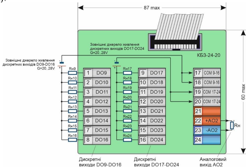
Рисунок Б.4.16 - Підключення сигналів модуля розширення МР-51-15 за допомогою клемно-блочного з'єднувача КБ3-24-20
