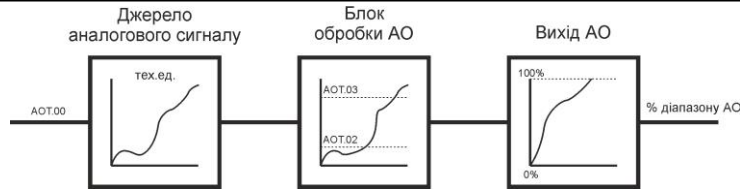
Рисунок 3.19 - Робота блоку аналогового виходу в режимі ретрансмісії
