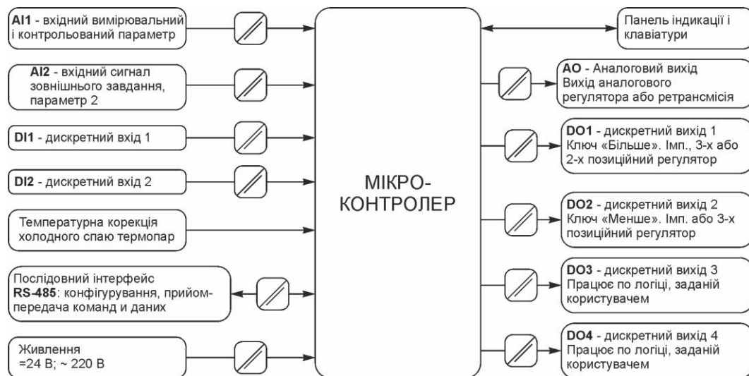
Рисунок 3.2 – Структурная схема регулятора МІК-121-К7
