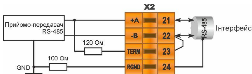
Рисунок Б.8 - Рекомендована схема підключення інтерфейсу RS-485
