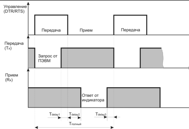
Рисунок В.1 - Тимчасові діаграми управління передачею і прийомом блоку інтерфейсів БПІ-485 (БПІ-52)
