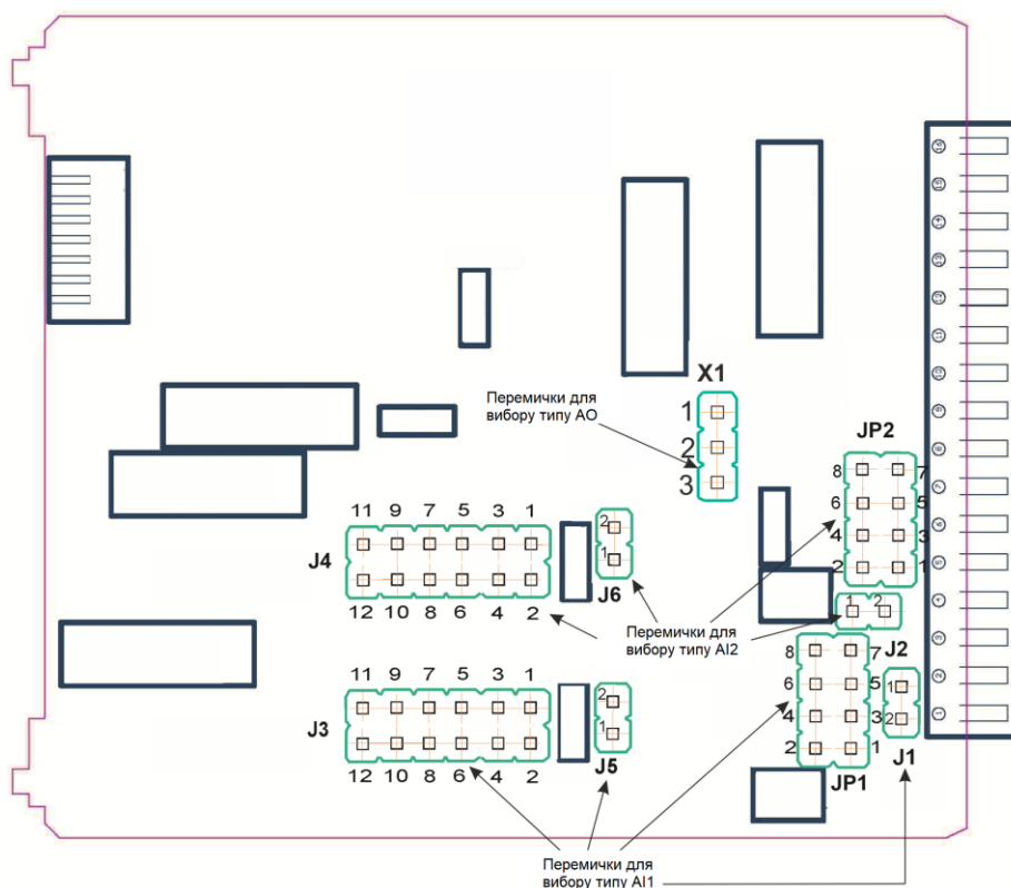
Рисунок 5.1 – Положення переминок на платі вхідних-вихідних сигналів
