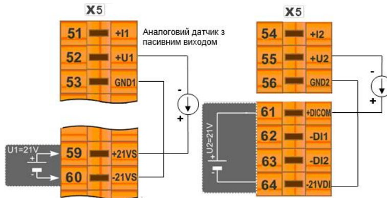
Рисунок Б.3 - Підключення до регулятора МІК-121-К7 аналогових давачів з пасивними виходами
