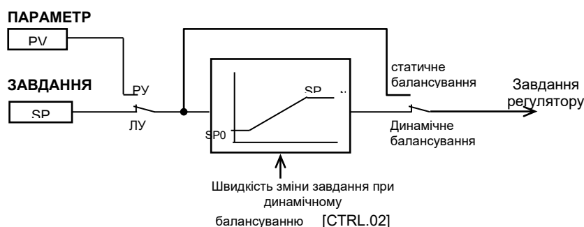
Рисунок 4.1 - Функціональна схема балансування регулятора MIK-121-K7
