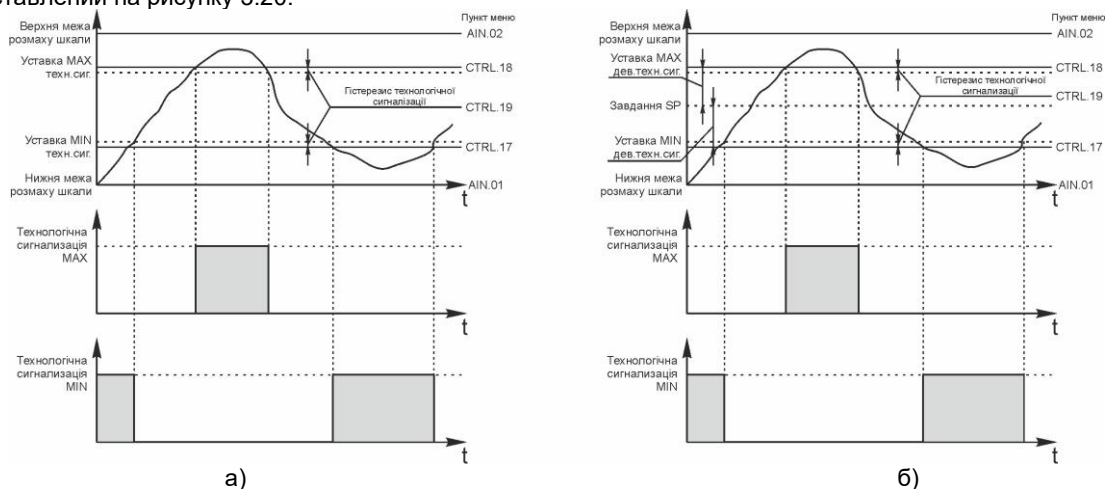
Рисунок 3.20 - Графік спрацьовування:
