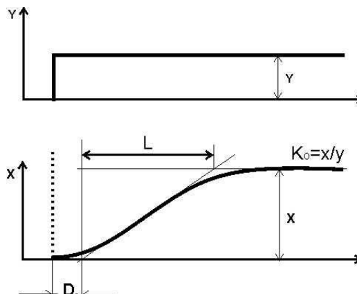
Рисунок 4.7 - Перехідна функція об'єкта регулювання з самовирівнюванням
