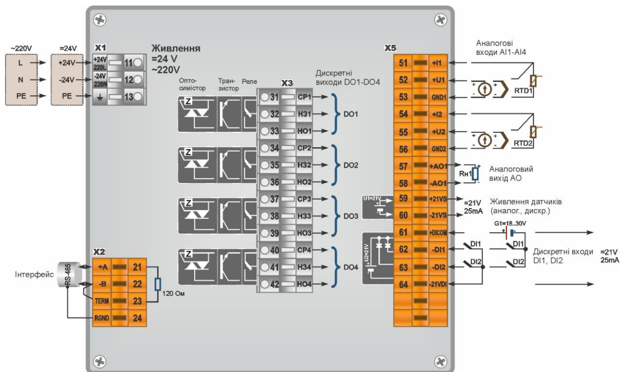
Рисунок Б.2 - Схема зовнішніх з'єднань регулятора МІК-121-К7
