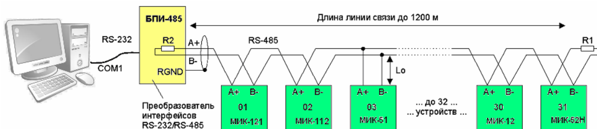
Рисунок Б.7 - Організація інтерфейсного зв'язку між комп'ютером і регуляторами
