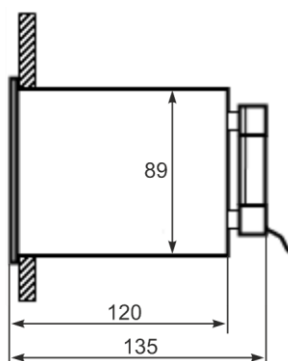
Рисунок А.2 - Габаритні розміри
