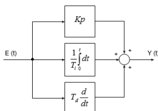
Рисунок 4.6 - Паралельна структура ПІД регулятора
