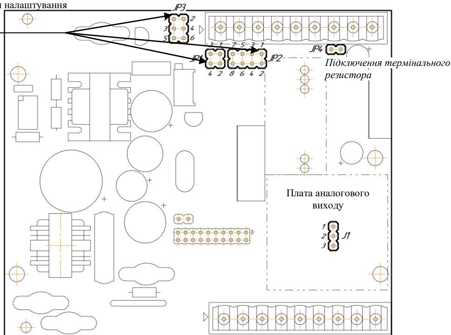
Рисунок 4.5 - Положення перемичок на платах регулятора МІК-111Н
