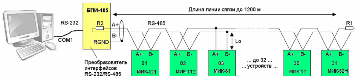
Рисунок Б.4 - Організація інтерфейсного зв'язку між комп'ютером і регуляторами
