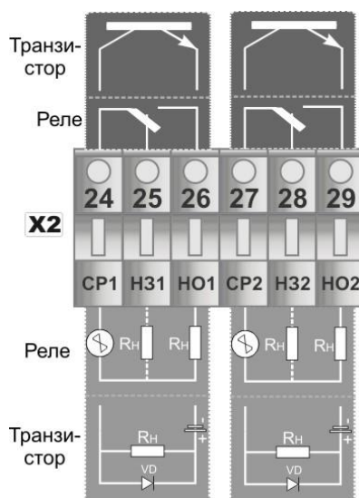
Рисунок Б.2 - Підключення індуктивних навантажень до регулятора МІК-111Н
