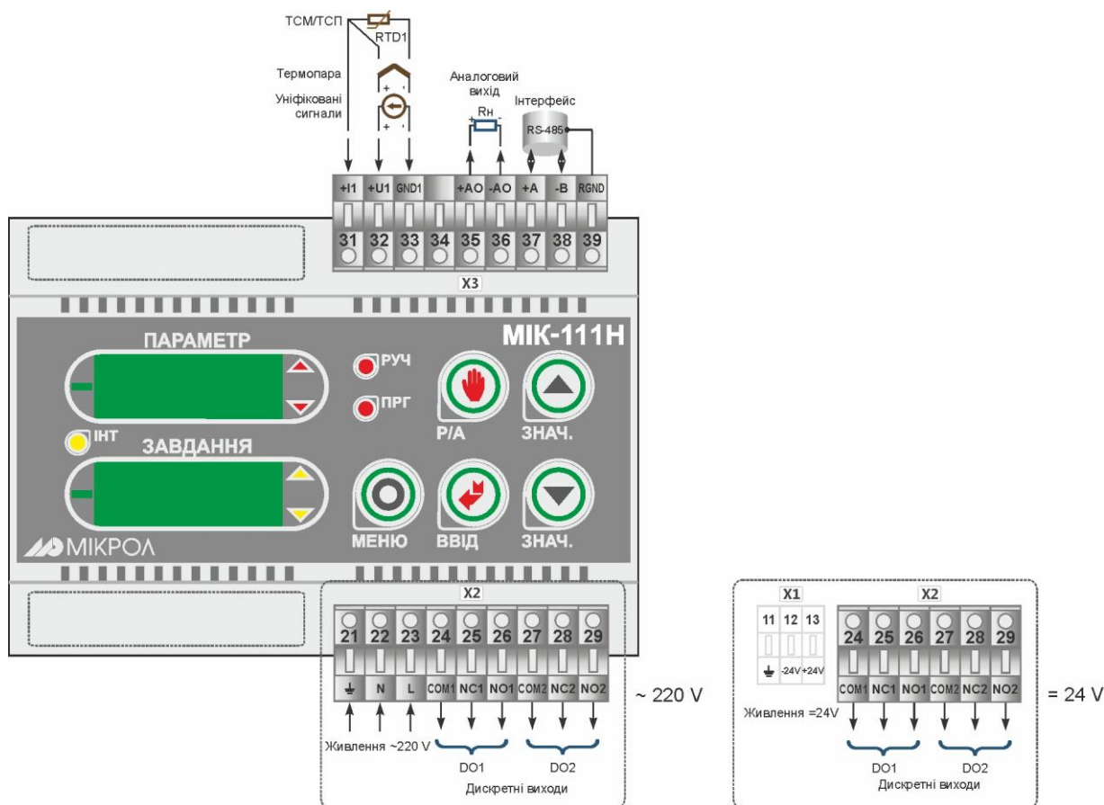
Рисунок Б.1 - Схема зовнішніх з'єднань регулятора МІК-111Н
