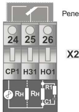
Рисунок Б.3 - Схема підключення індуктивного навантаження для механічного реле
