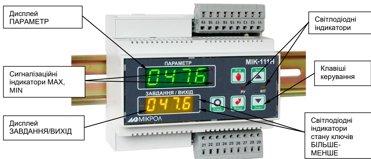
Рисунок 3.1 - Зовнішній вигляд регулятора МІК-111Н
