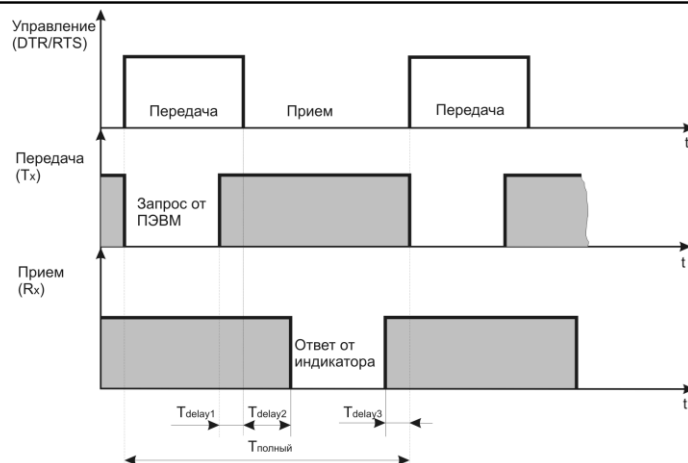
Рисунок В.1 - Часові діаграми управління передачею і прийомом блоку інтерфейсів БПИ-485 (БПИ-52)
