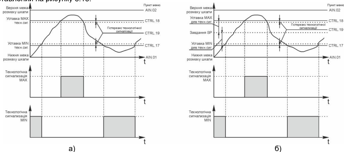
Рисунок 3.13 - Графік спрацьовування: а) абсолютної технологічної сигналізації п. CTRL.16 = 0000 б) деіаційної технологічної сигналізації п. CTRL.16 = 0001.
