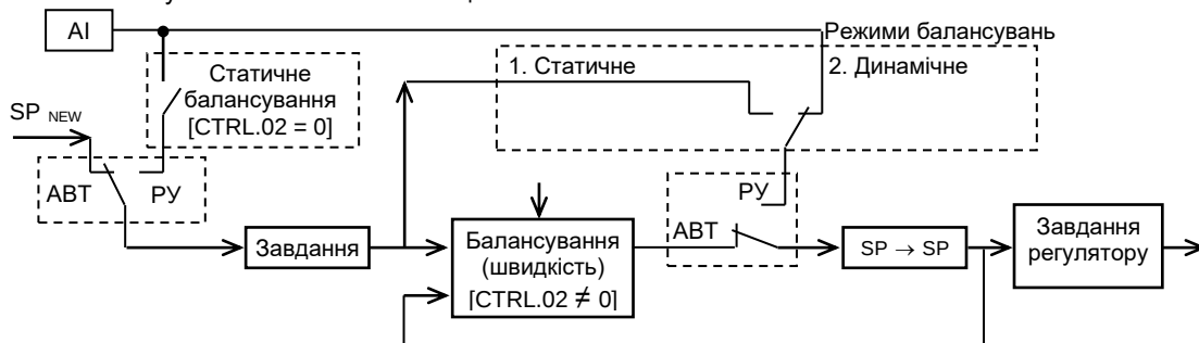
Рисунок 4.2 - Функціональна схема балансування регулятора МІК-111Н
