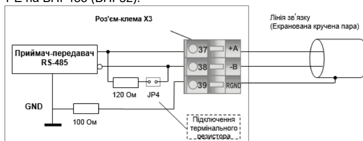
Рисунок Б. 8. - Рекомендована схема підключення інтерфейсу RS-485
