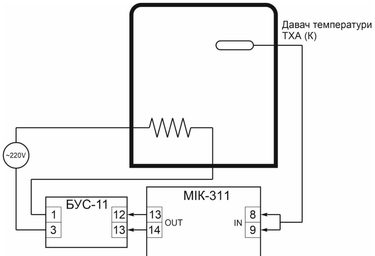
Рисунок 4.11 – Схема та процес термічної обробки
