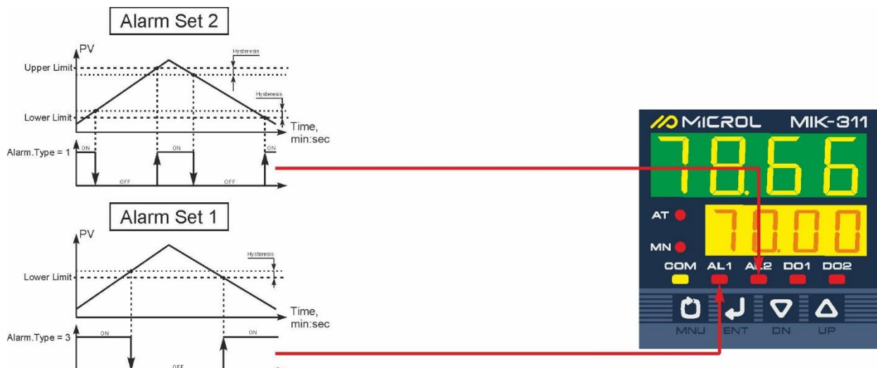
Рисунок 4.9 – Принцип роботи сигналізації
