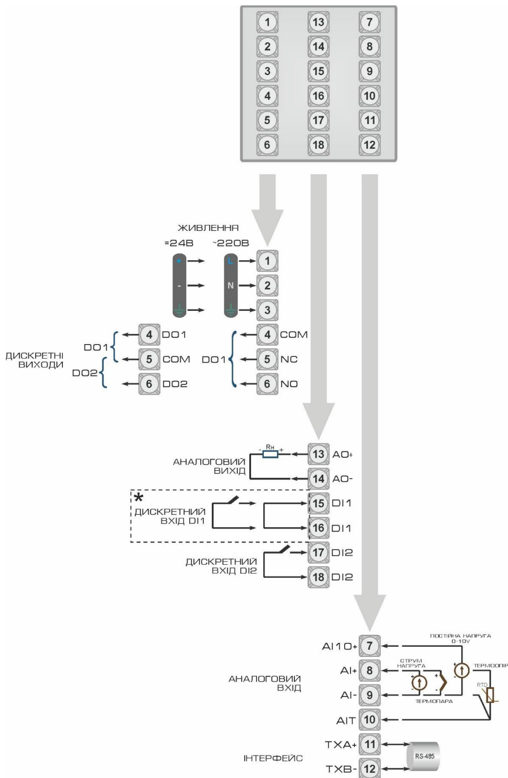
Рисунок Б.1 - Схема зовнішніх з'єднань регулятора МІК-311-К11
