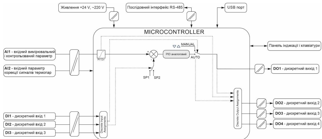
Рисунок 4.7 - Структурна схема регулятора МІК-311-К11 в режимі роботи ПІД-ШІМ регулятора
