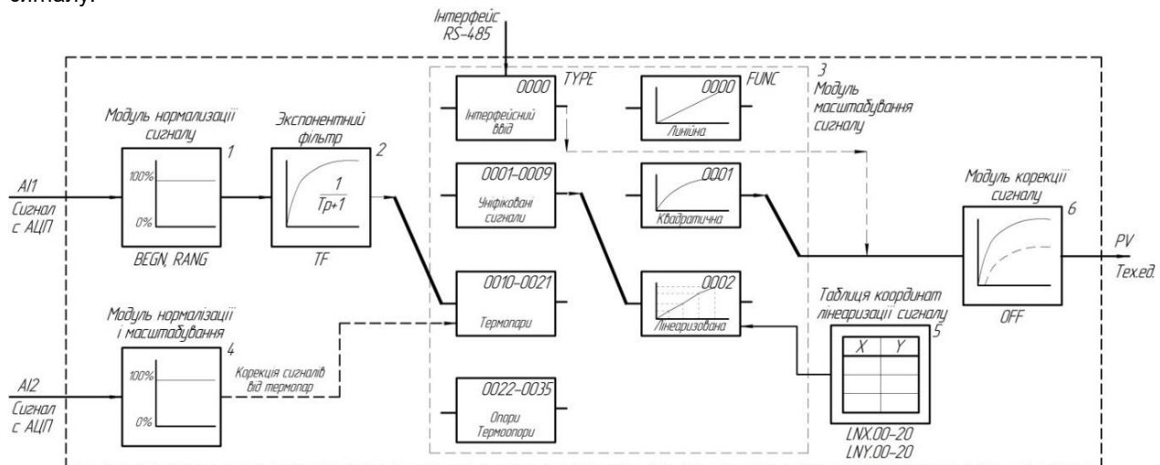
Рисунок 3.6 - Функціональна схема блоку перетворення вхідного сигналу
