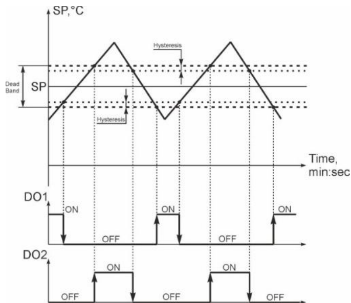
Рисунок 4.5 – Графік роботи дискретними виходами трипозиційного регулятора з використання зони нечутливості
