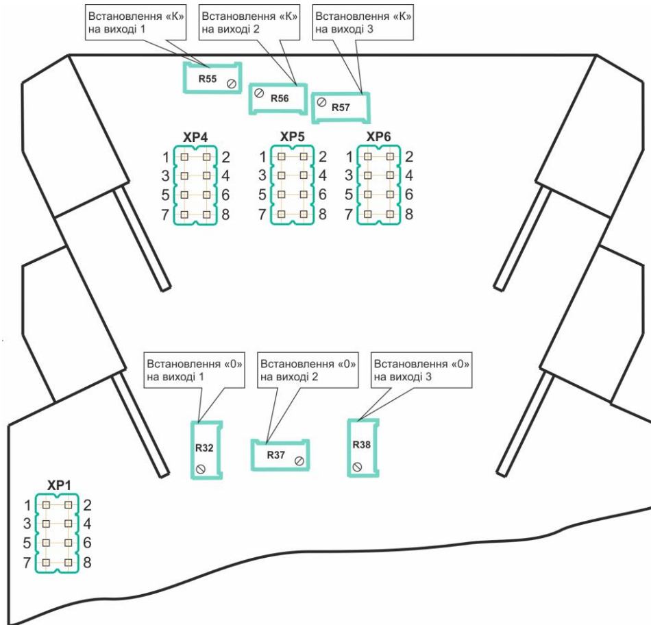
Рисунок 3.1- Розміщення блоків перемичок вибору вхідних і вихідних сигналів
