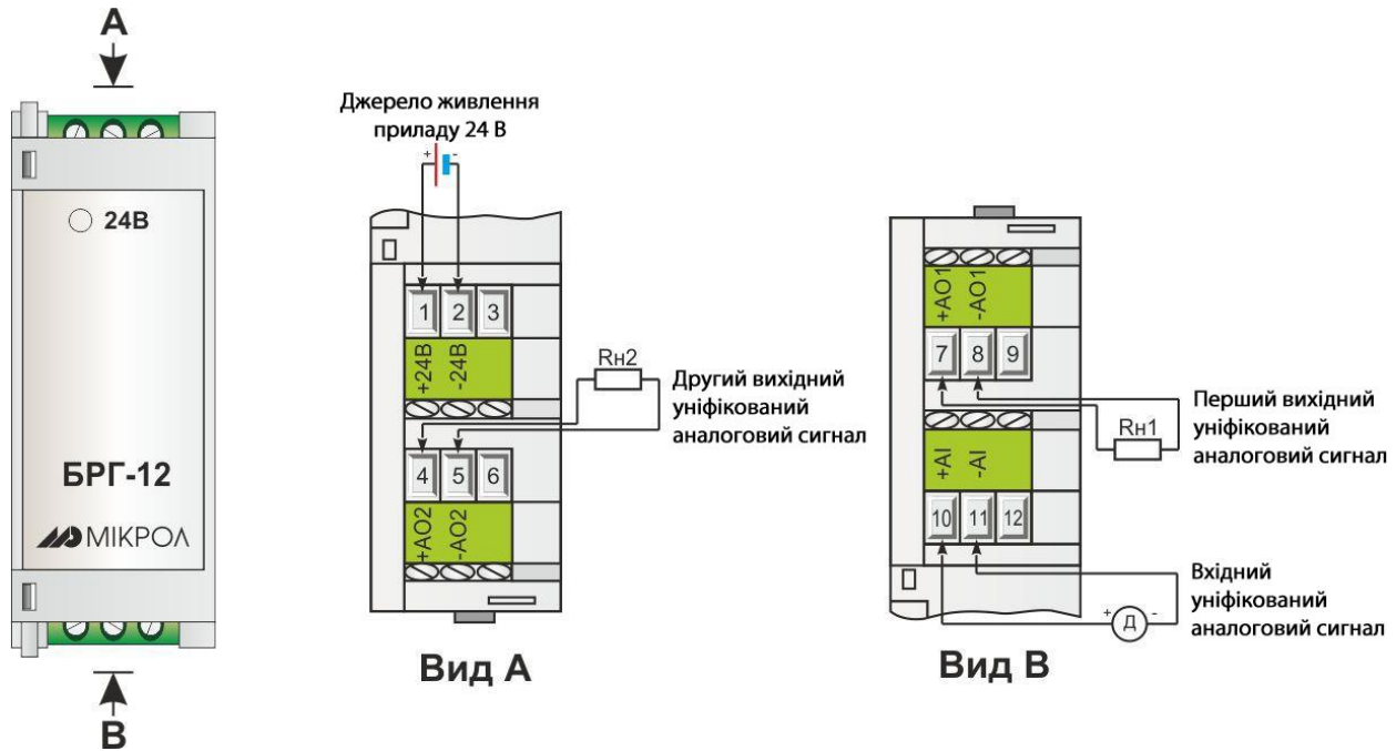
Рисунок 3.3 - Схема електрична підключення блоку БРГ-12
