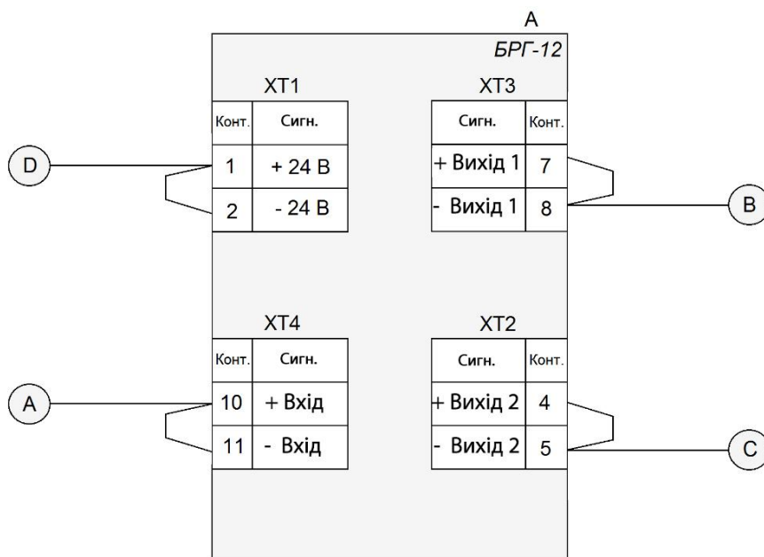
Рисунок Б.1 – Схема перевірки опору ізоляції
