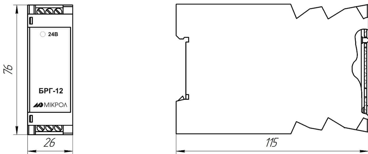
Рисунок 1.1 - Перетворювач-розгалужувач аналогових сигналів БРГ-12
