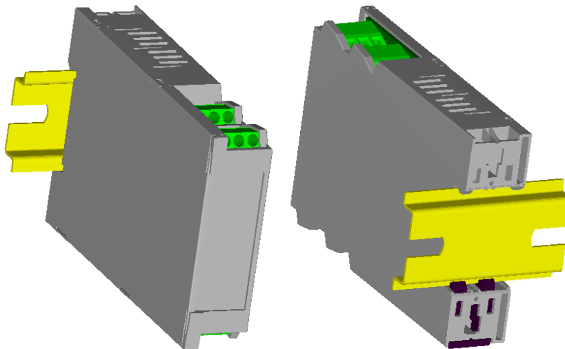
Рисунок 3.2 – Схема кріплення блоку БРГ-12 на DIN-рейку
