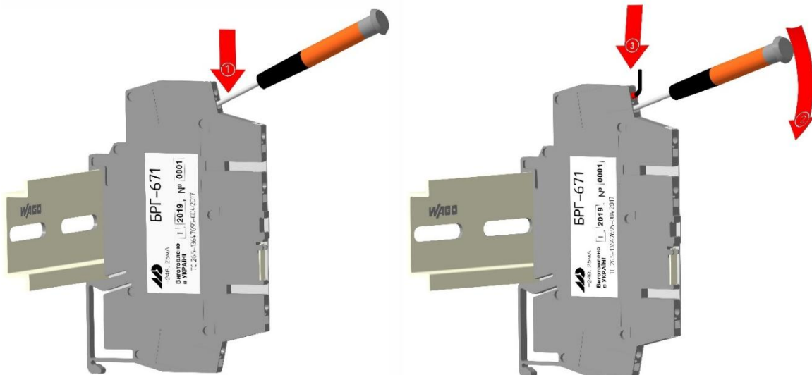
Рисунок 3.3 - Схема установки дротів за допомогою плоскої викрутки
