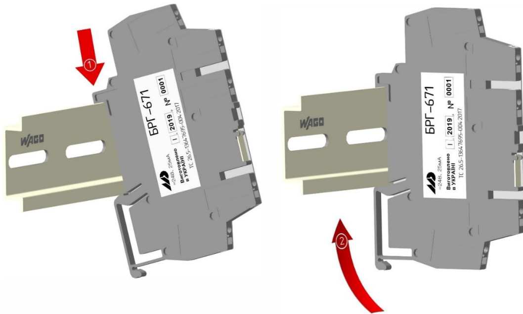
Рисунок 3.2 - Схема кріплення блоку БРГ-671 на DIN-рейку
