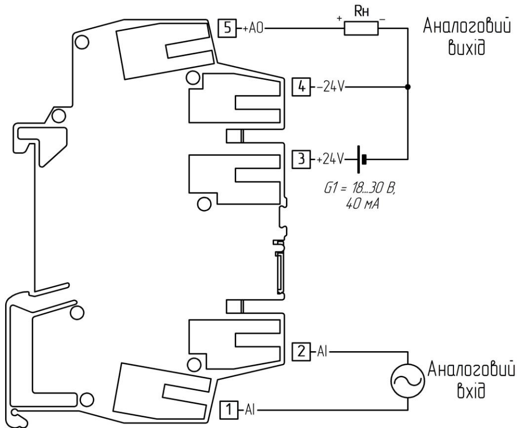
Рисунок 3.4 - Схема зовнішніх з'єднань перетворювача ПНС-653
