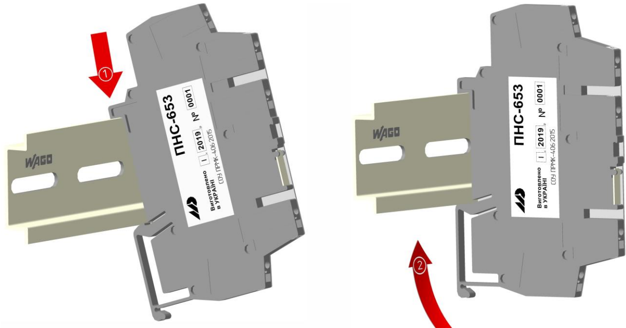
Рисунок 3.2 - Схема кріплення перетворювача ПНС-653 на DIN-рейку
